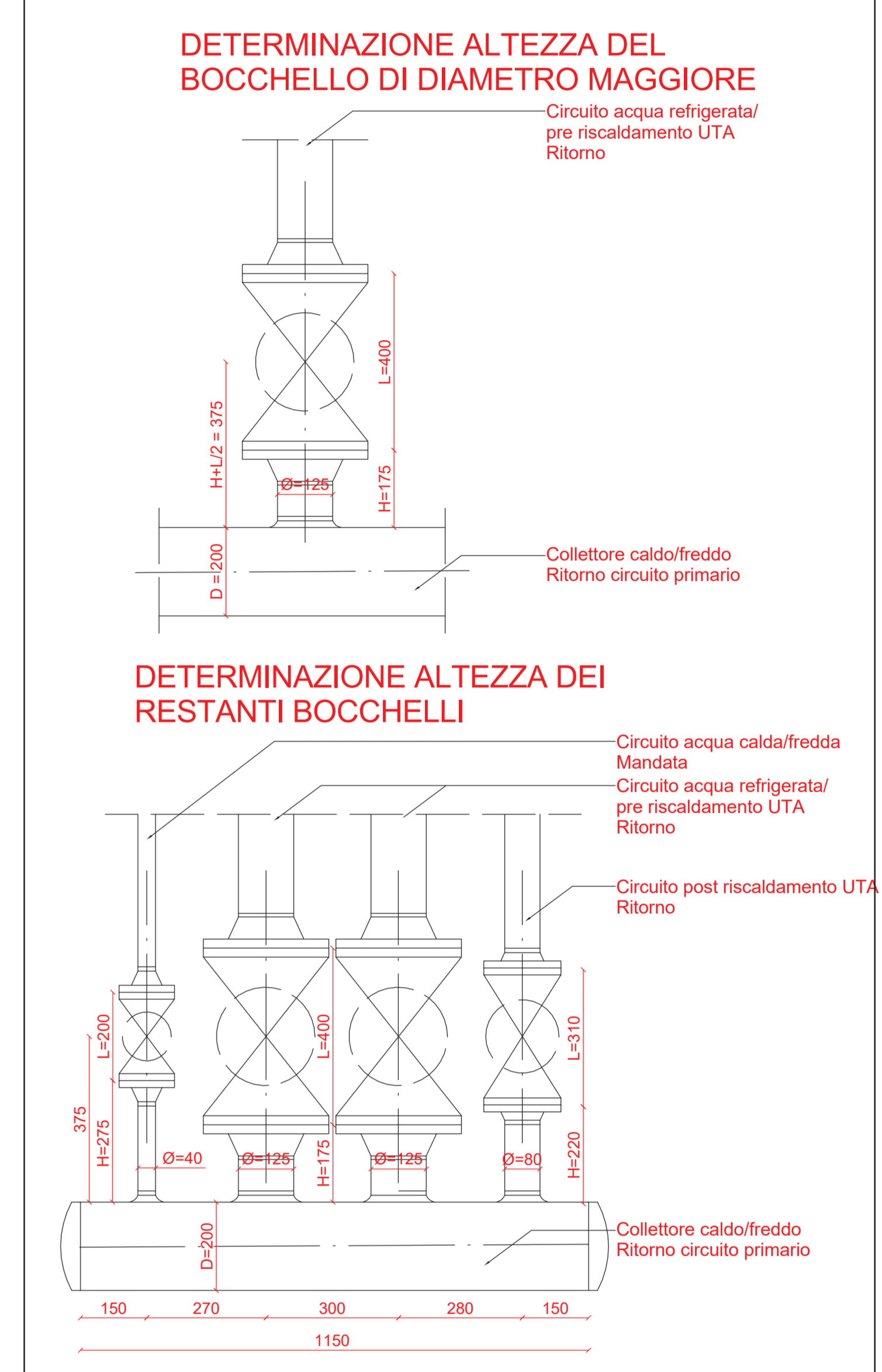
Dettaglio collettori SCALA 1:10
