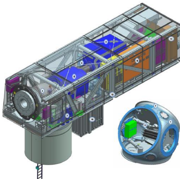
Figura 2. VSG 6.0-170. Disposizione dei componenti in navicella
