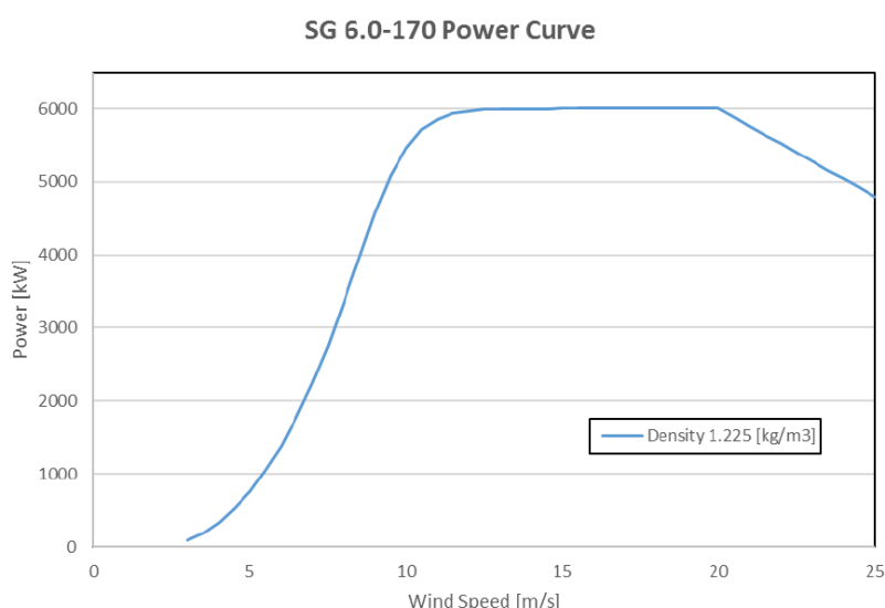
Figura 1. Curva di Potenza di una SG 6.0-170
