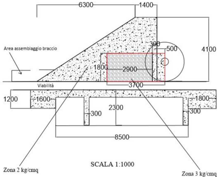
Figura 5. Piazzola aerogeneratore
