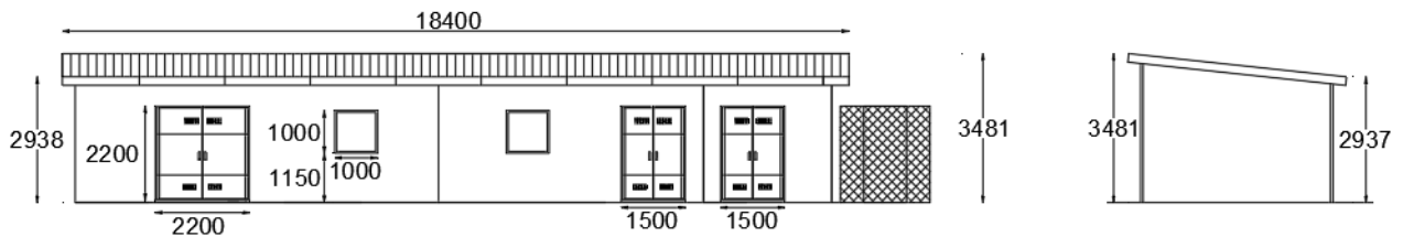
Fig. 3 – Prospetto fabbricato tecnologico.
