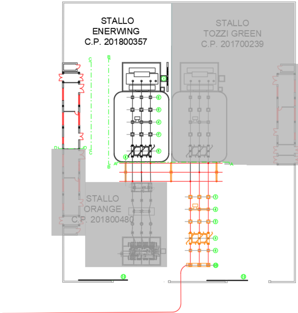
Fig. 2 – Layout in SSE Produttore in corso di autorizzazione.
