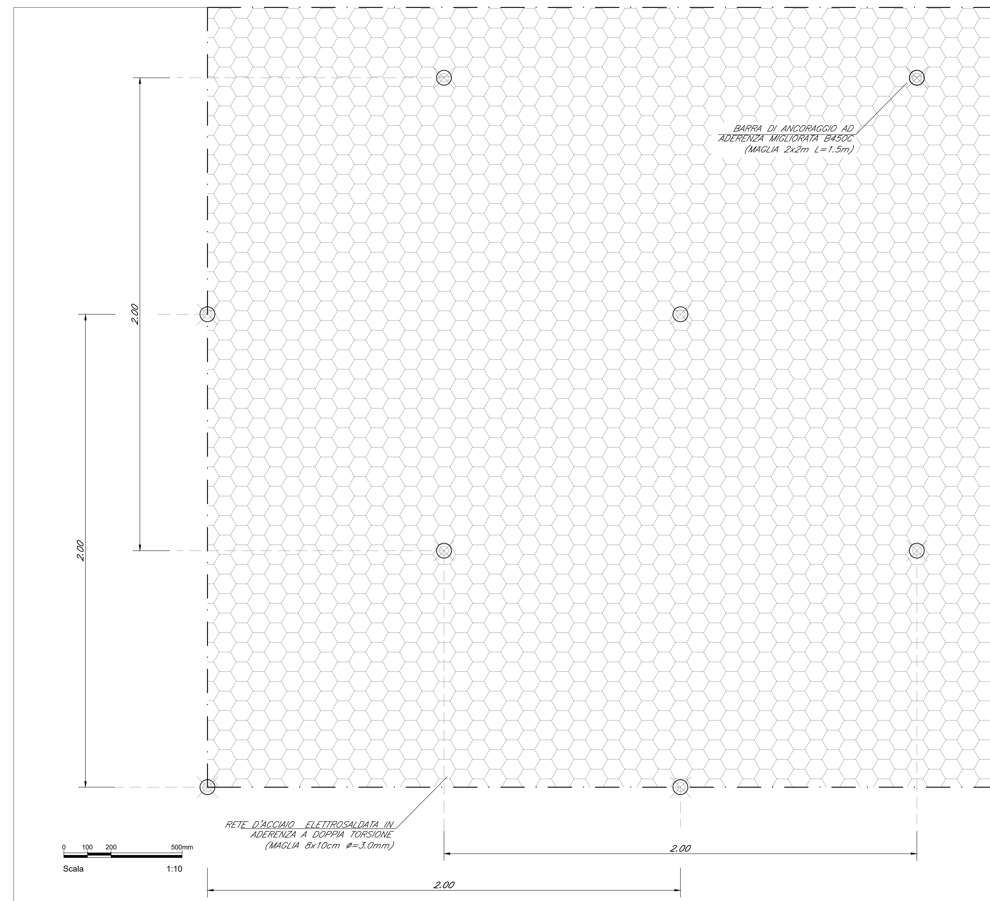
DETTAGLIO 2 Rete in aderenza - Prospetto Scala 1:10
