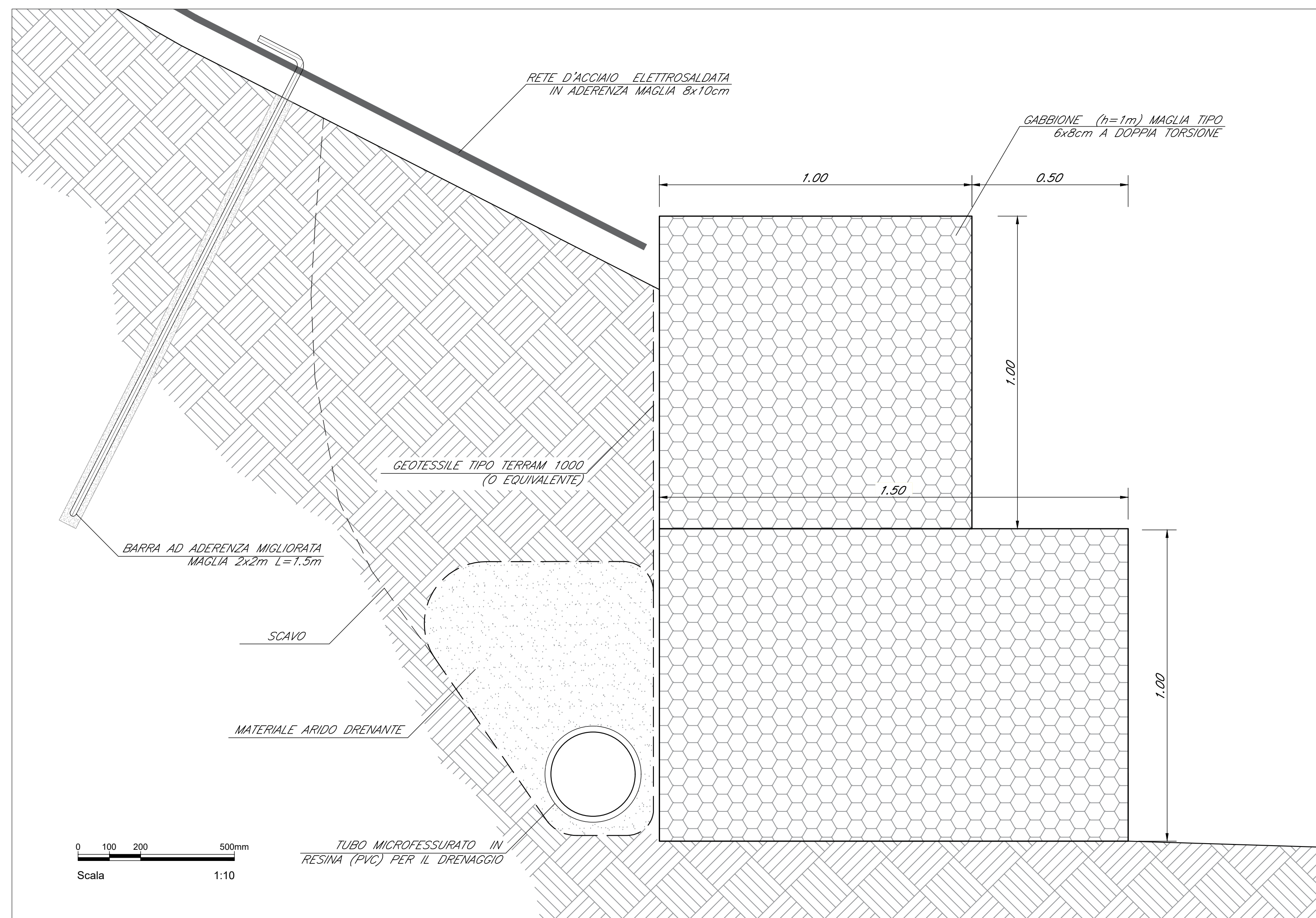
DETTAGLIO 3 Muro di gabbioni Scala 1:10
