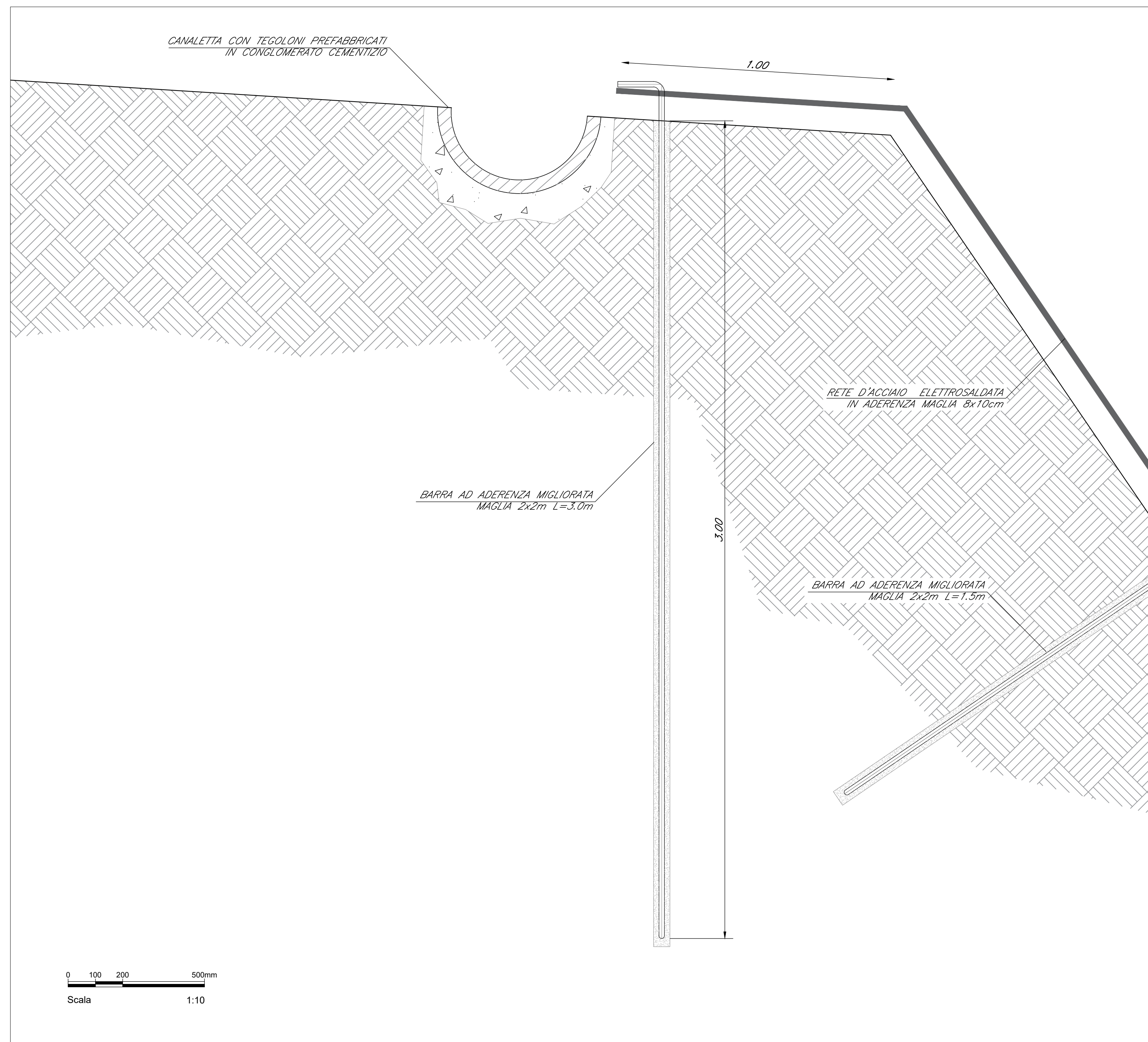
DETTAGLIO 1 Canaletta in conglomerato cementizio Scala 1:10
