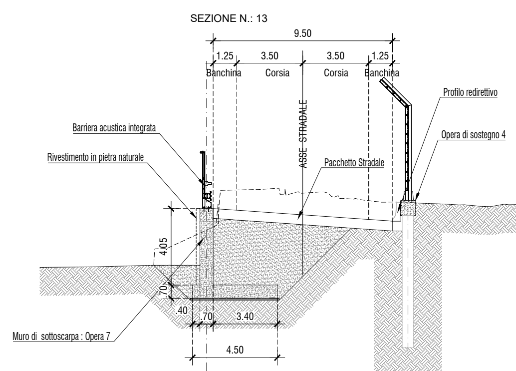
SEZIONE TRASVERSALE scala 1:200
