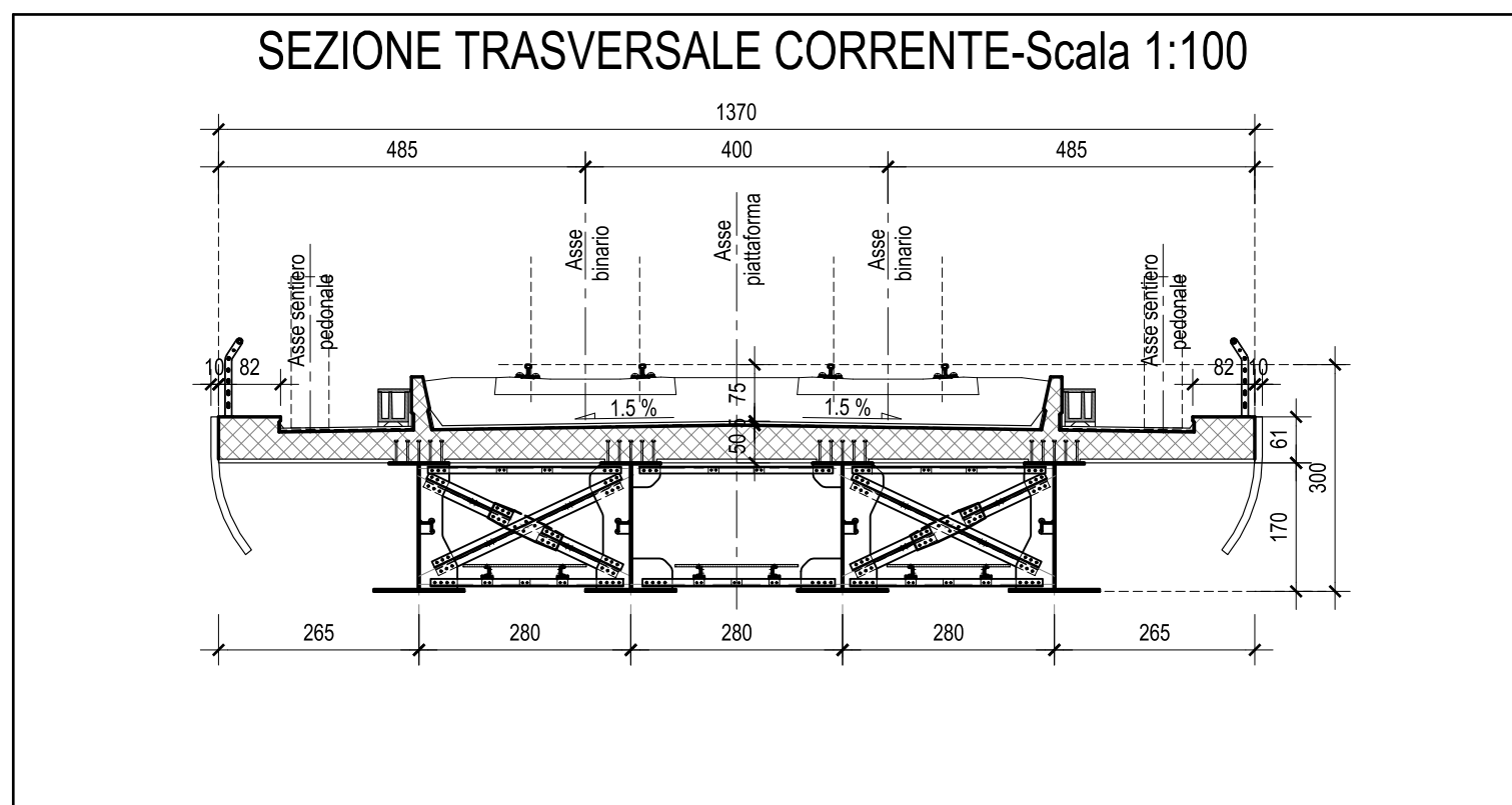
SEZIONE TRASVERSALE CORRENTE-Scala 1:100
