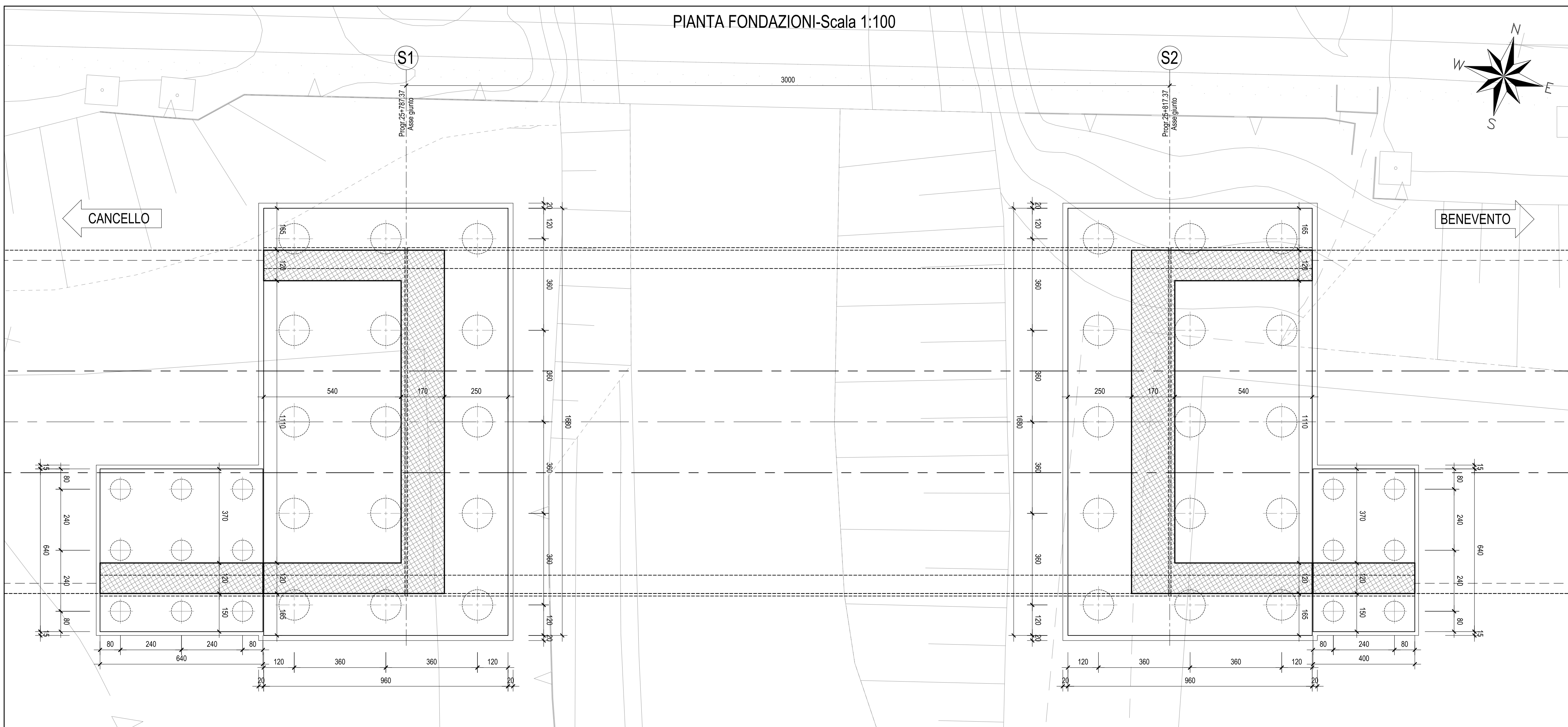
PIANTA FONDAZIONI-Scala 1:100
