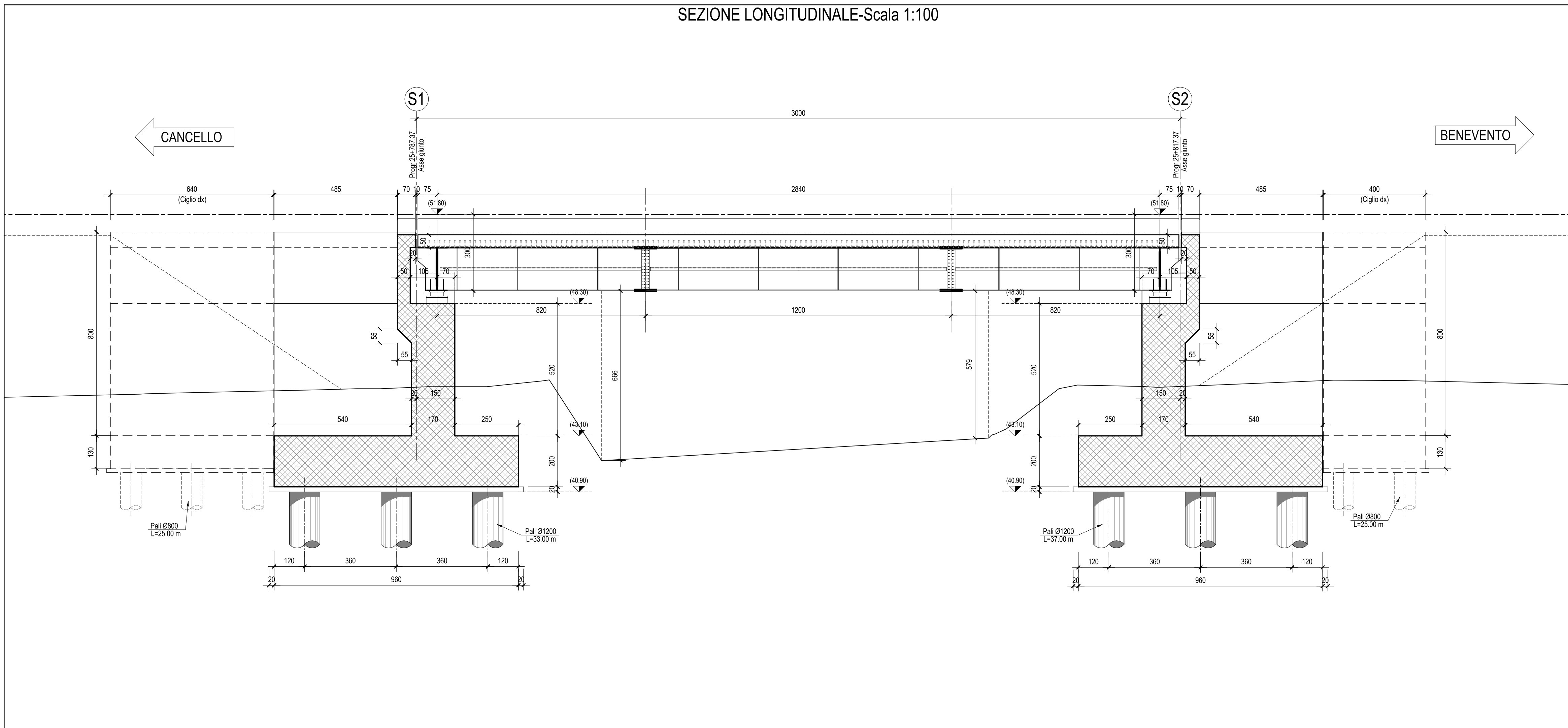
SEZIONE LONGITUDINALE-Scala 1:100
