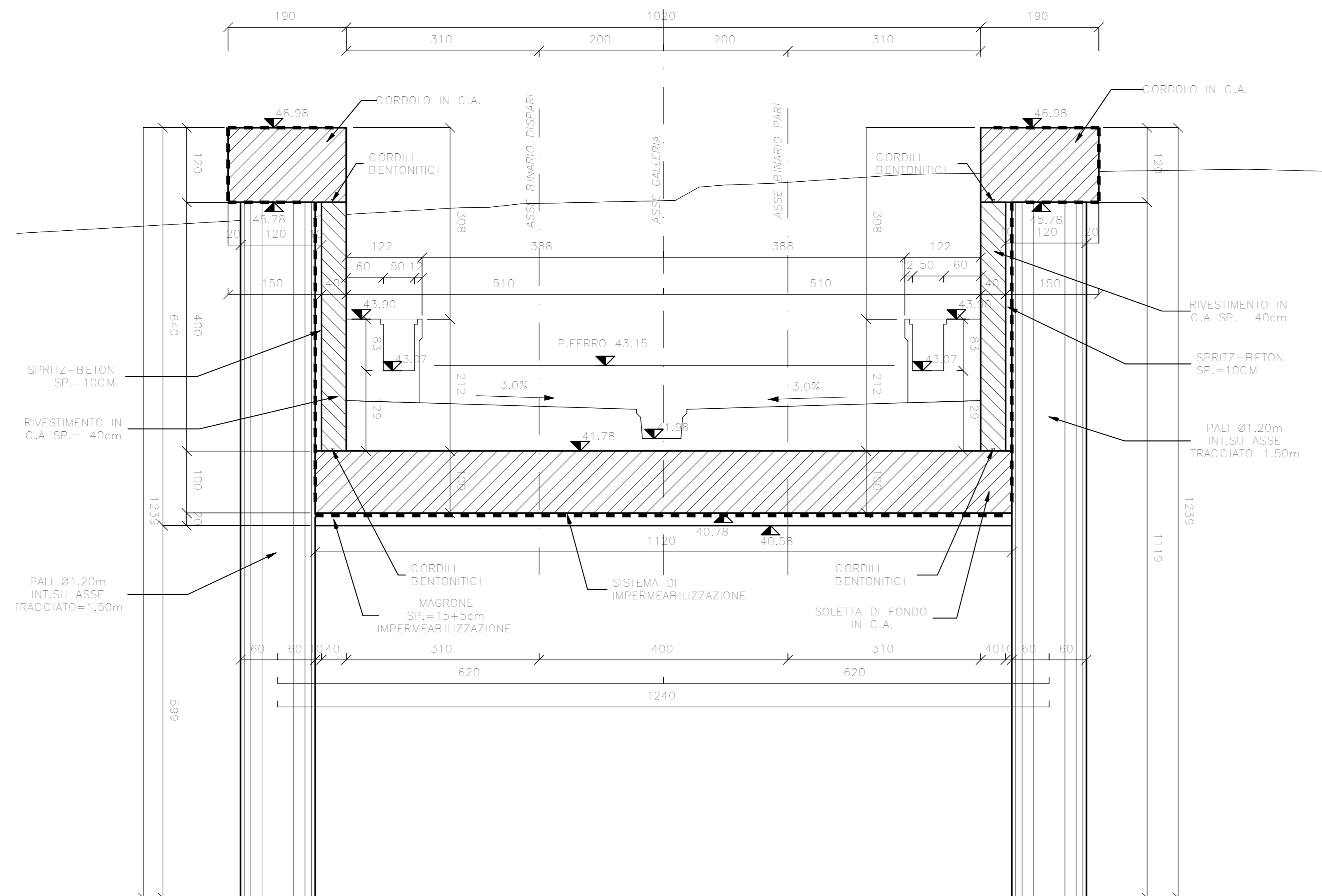
SEZIONE D-D -Scala 1 : 50
