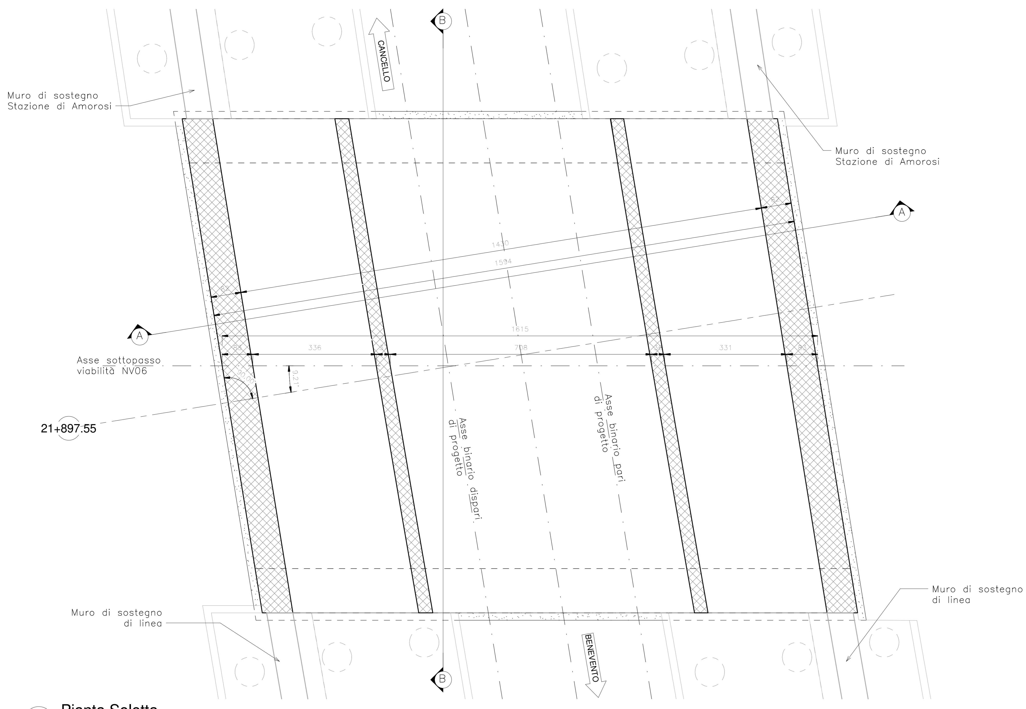
2 Pianta Soletta BB.SL.04.0.0.001 1:50
