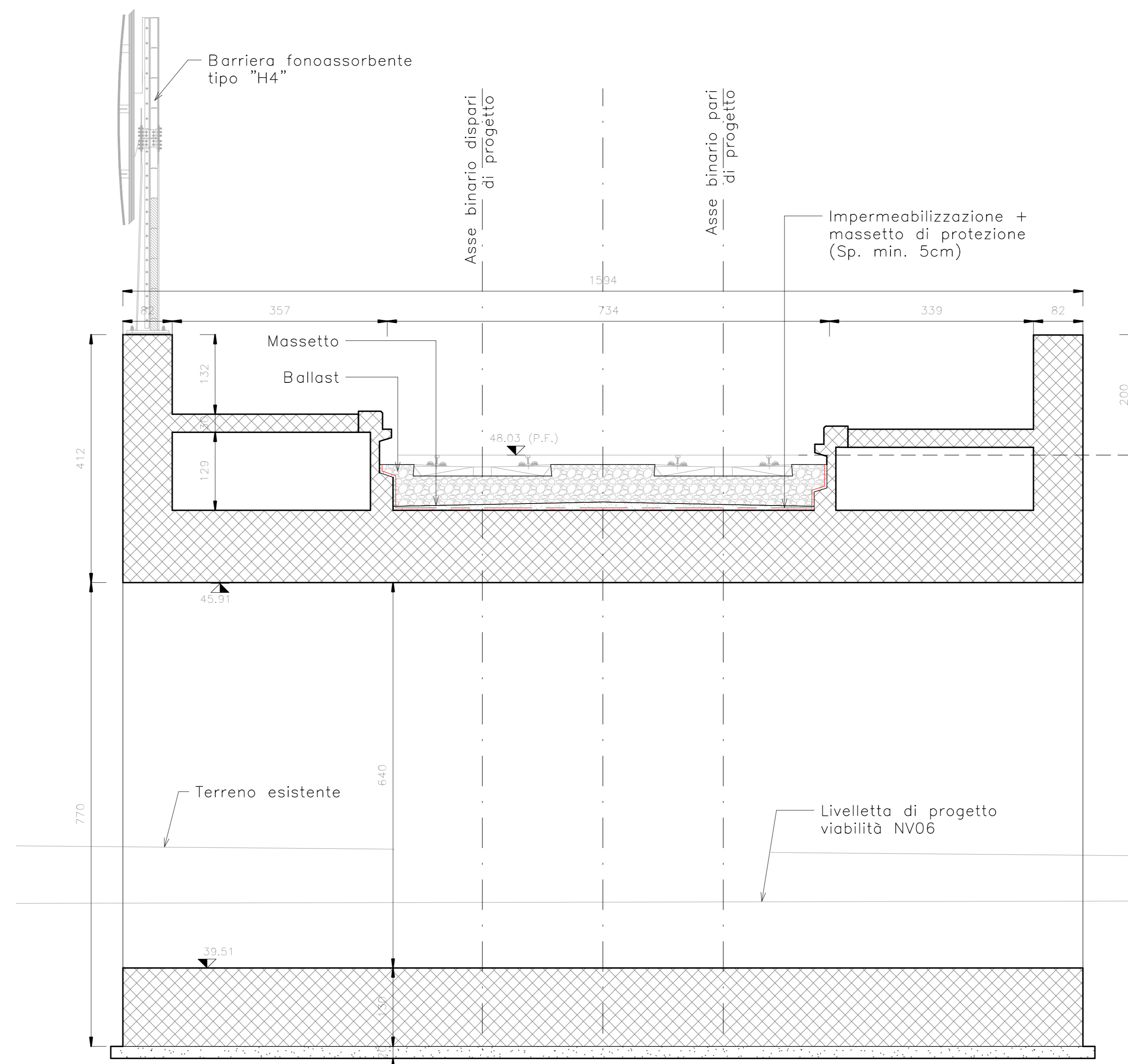
A Sezione A-A BB.SL.04.0.0.001 1:50
