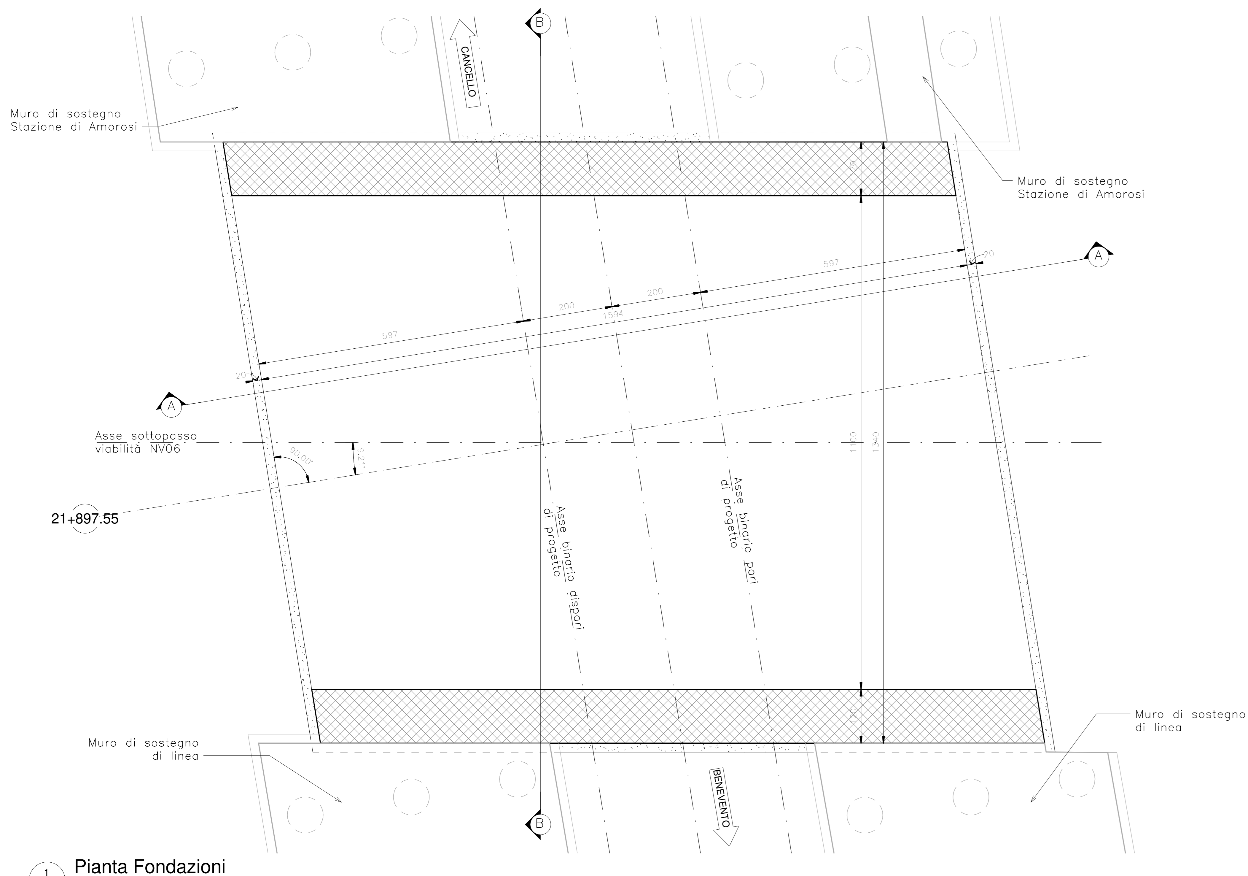
1 Pianta Fondazioni BB.SL.04.0.0.001 1:50
