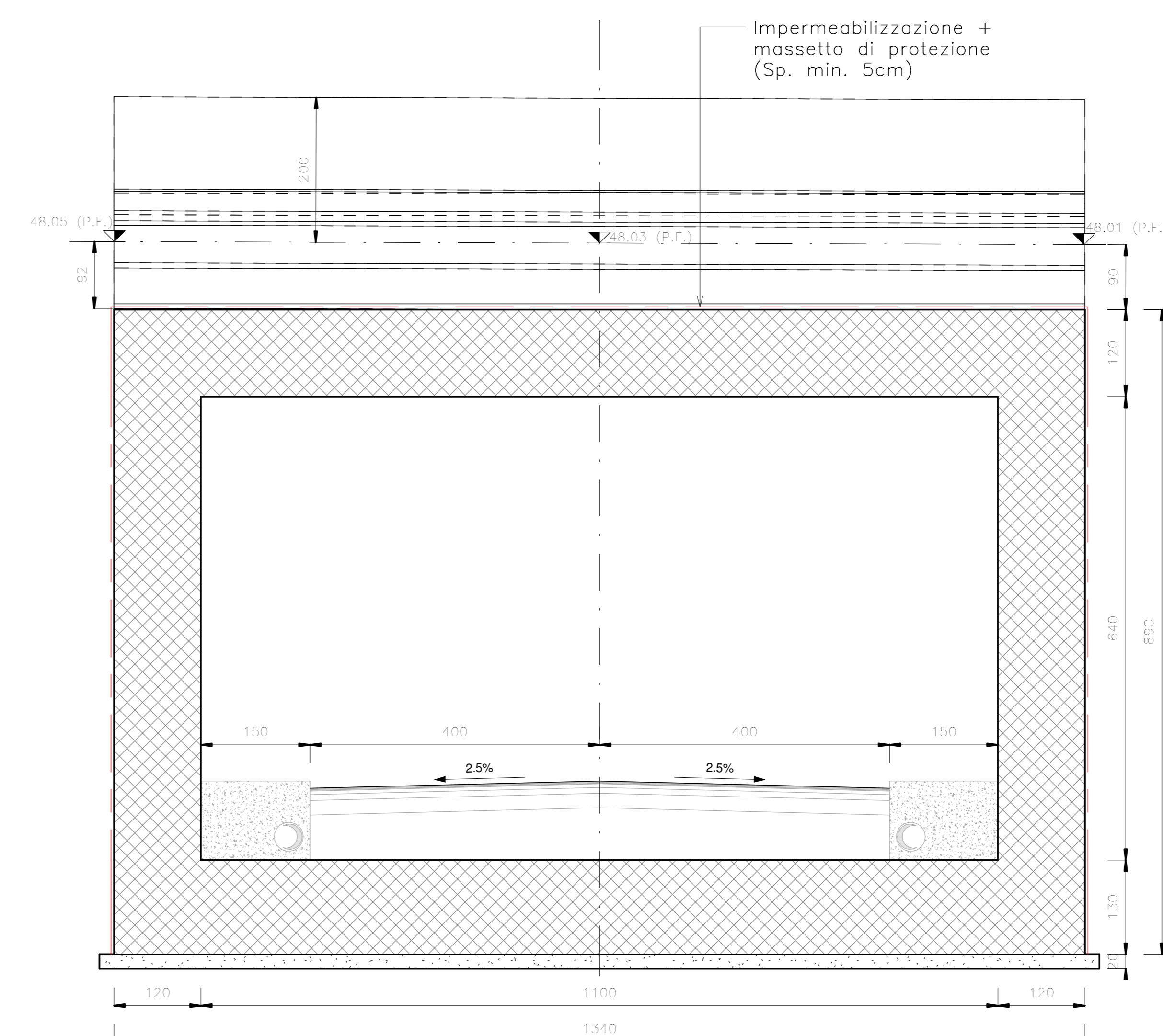
B Sezione B-B BB.SL.04.0.0.001 1:50
