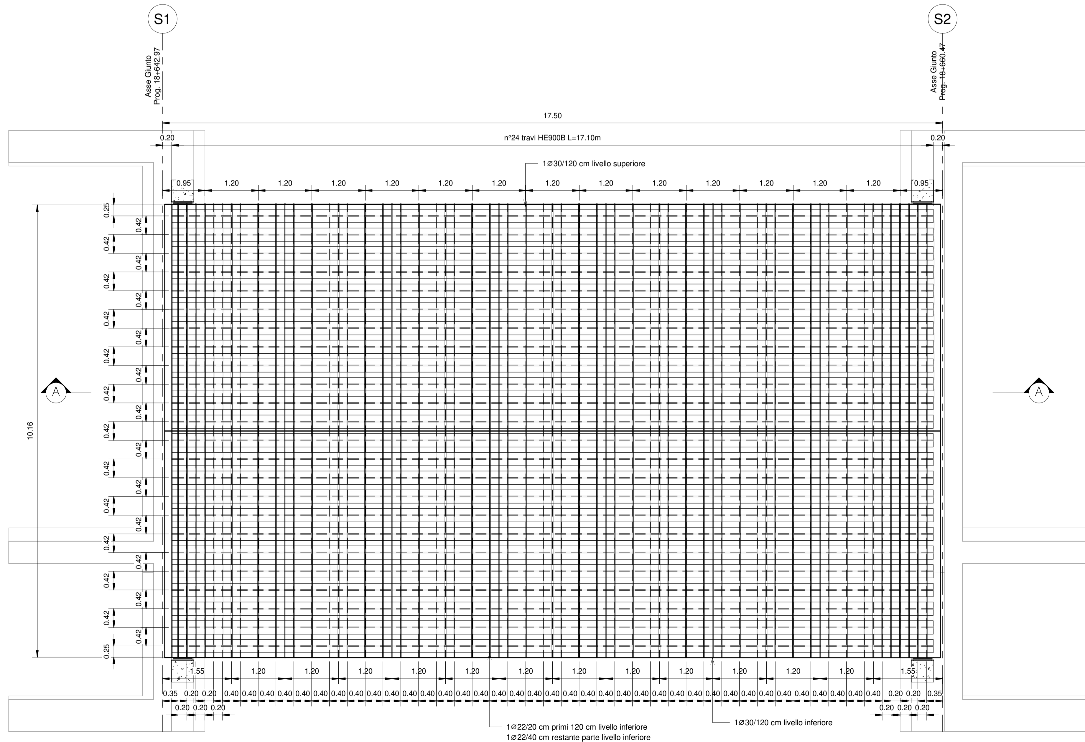
B Pianta Impalcato - Sezione B-B BZ.VI03.0.7.001 1 : 50
