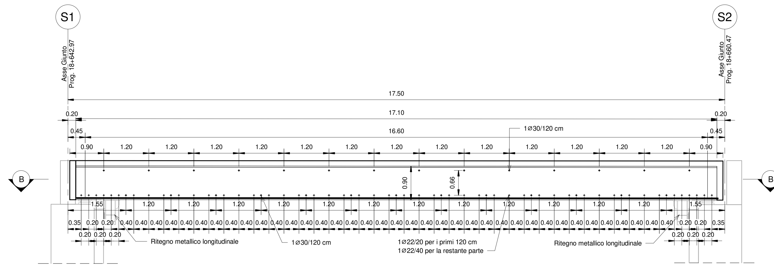
A Sezione Impalcato - Sezione A-A BZ.VI03.0.7.001 1 : 50
