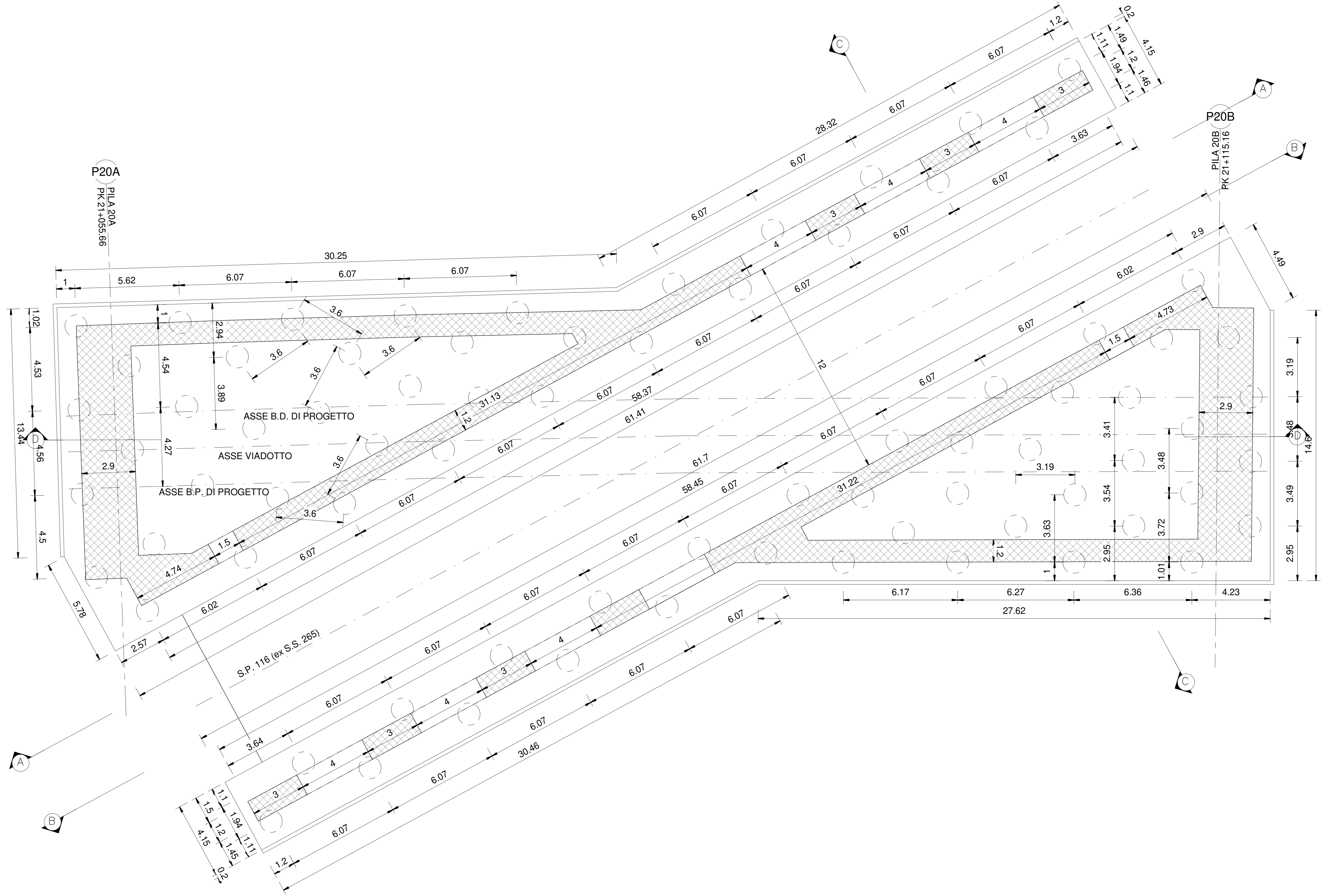
1 B2V0600002A Struttura ad archi - Pianta fondazioni 1 : 100
