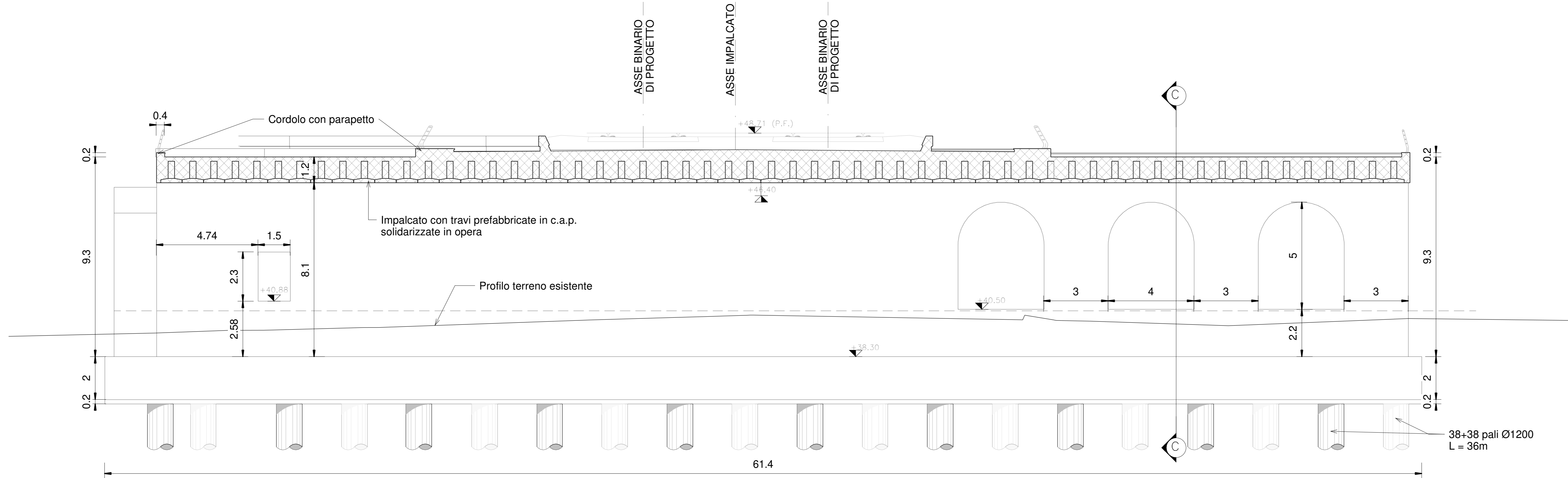
A B2V0600002A Struttura ad archi - Sezione A-A 1 : 100
