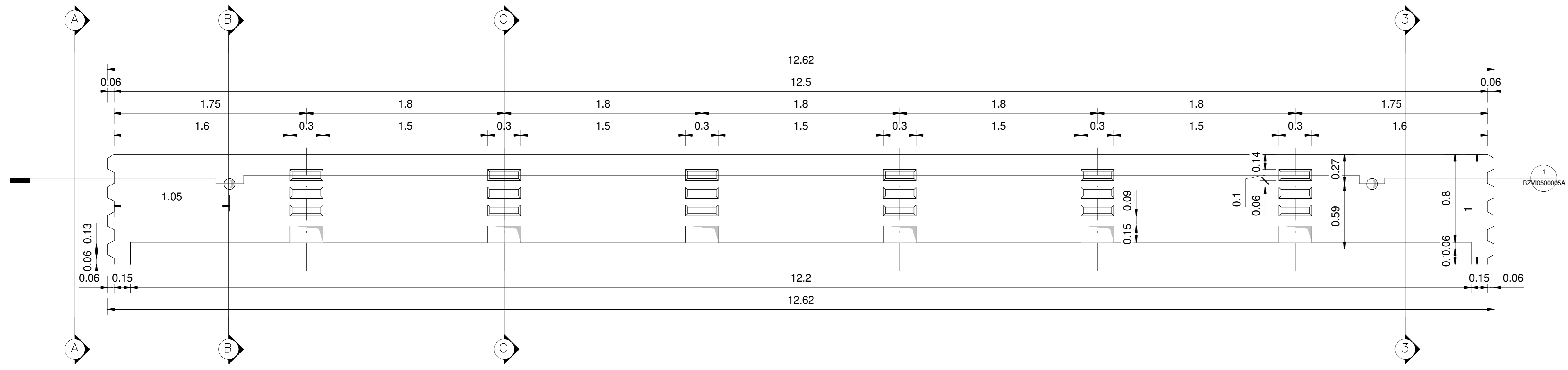
2 Travi in c.a.p. - Prospetto 1 : 20
