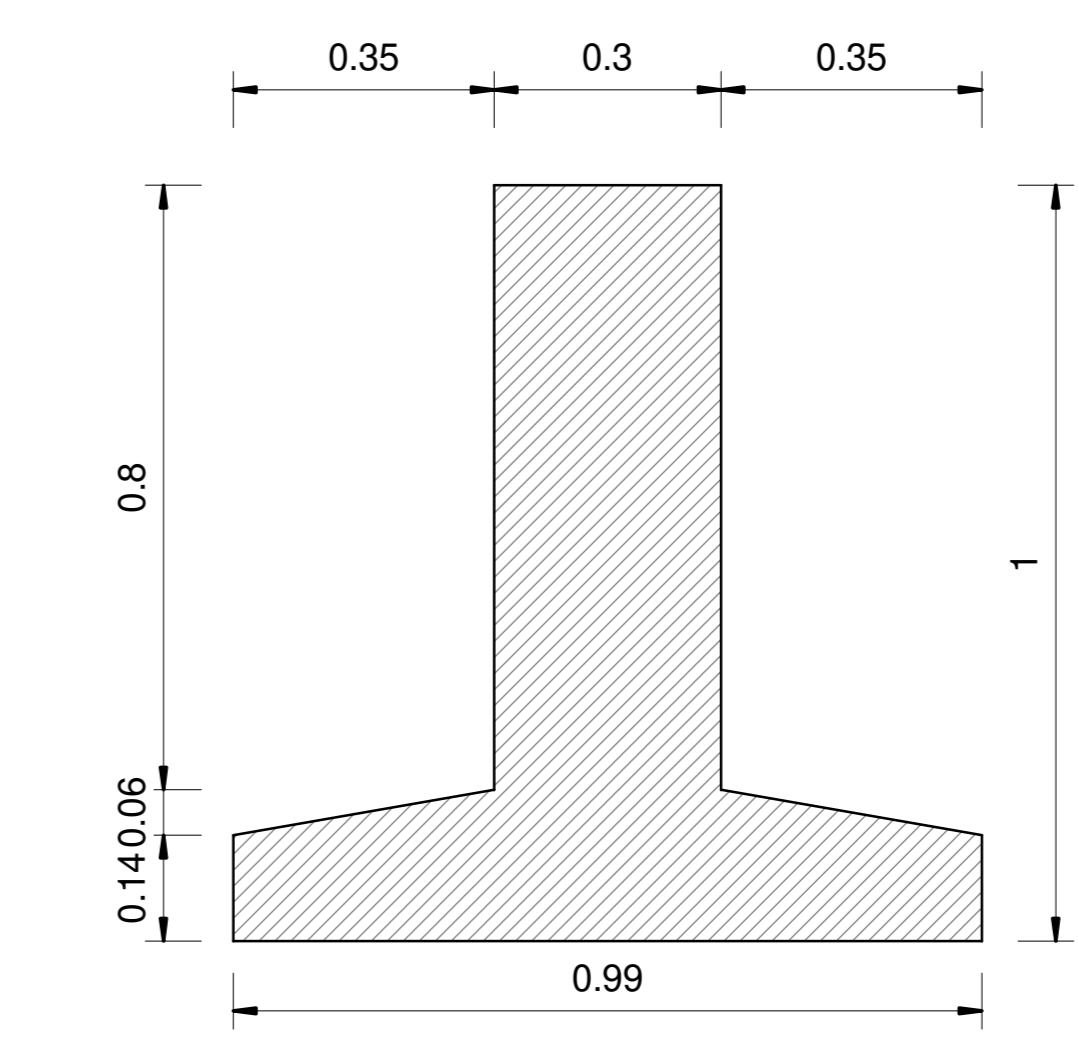
C Trave in c.a.p. - Sezione C-C 1 : 10
