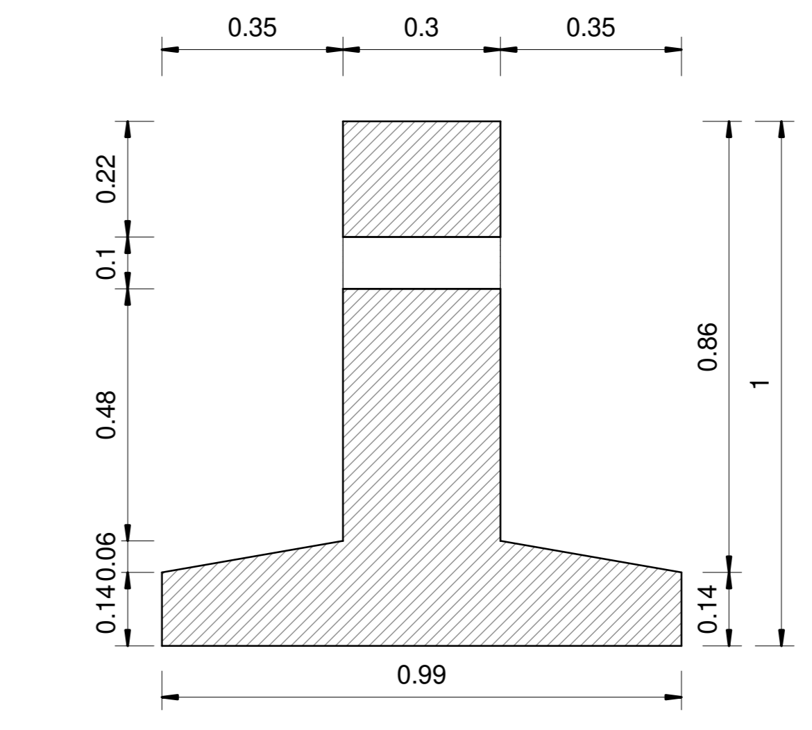
B Trave in c.a.p. - Sezione B-B 1 : 10
