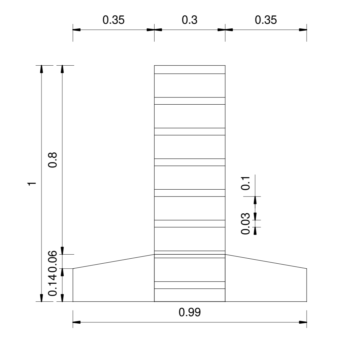
A Trave in c.a.p. - Sezione A-A 1 : 10
