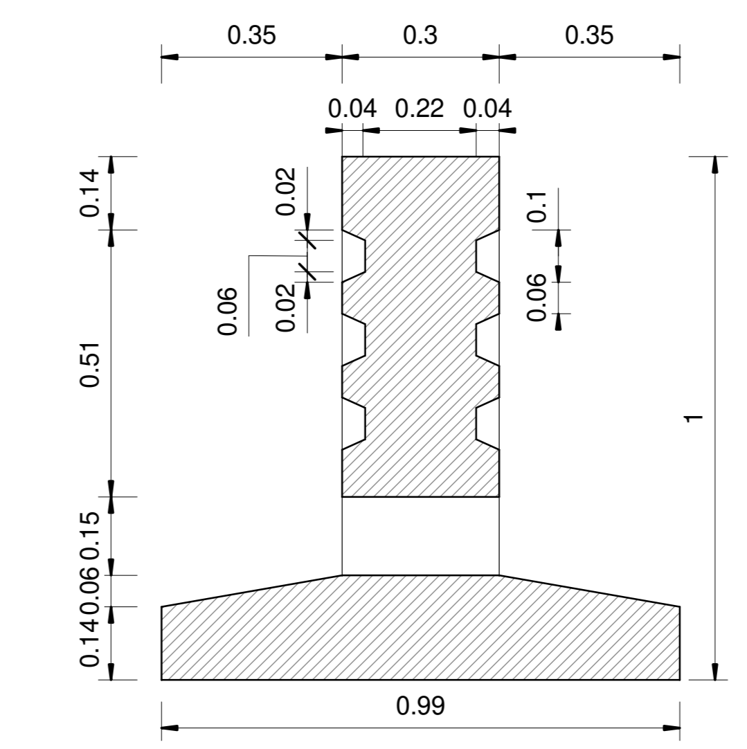
C Trave in c.a.p. - Sezione C-C 1 : 10
