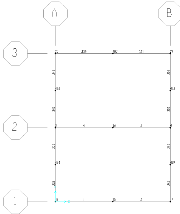
Figura 7-2 Numerazione frames e nodi piano copertura.
