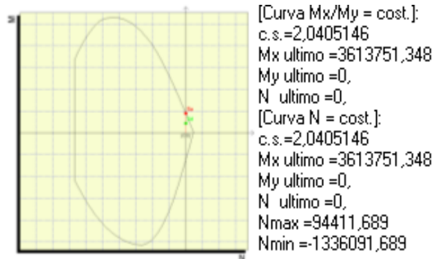
Figura 9-1 Sezione di sx: armatura sotto pilastro (momento positivo), sezione di dx: armatura in campata (momento negativo).
