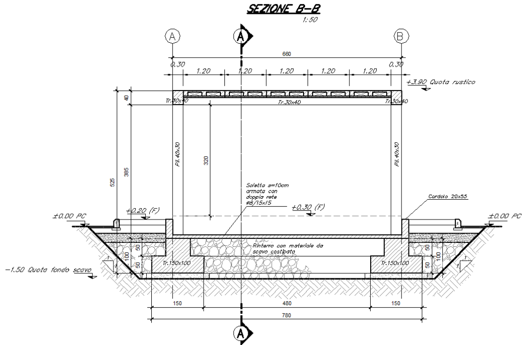
Figura 2 – Sezione Trasversale
