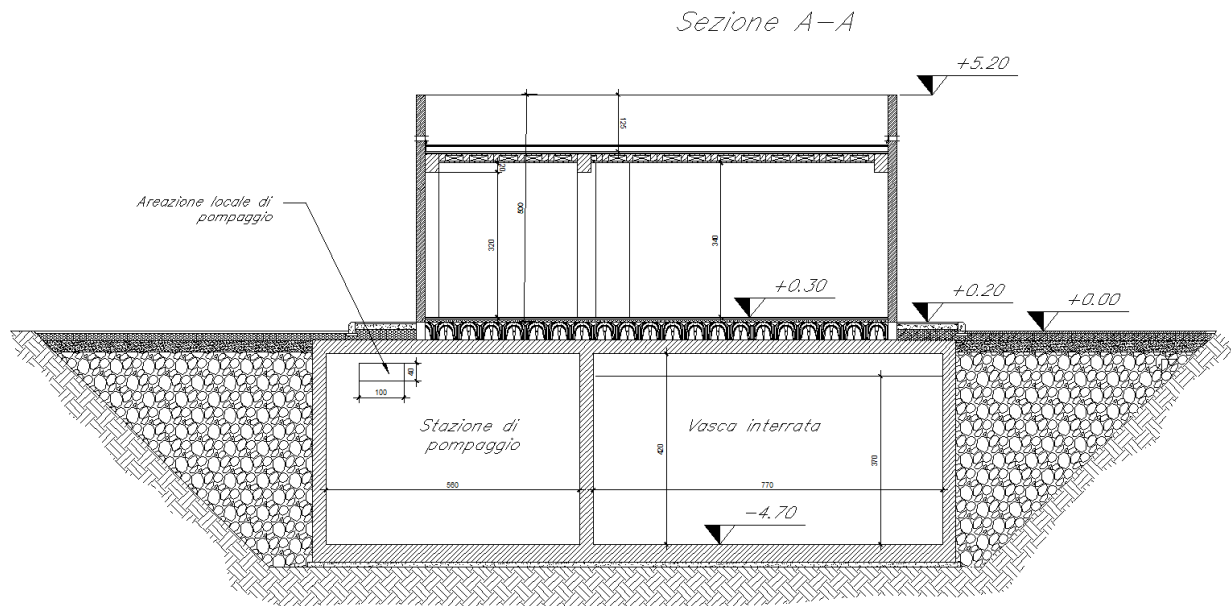
Figura 1 – Sezione Longitudinale
