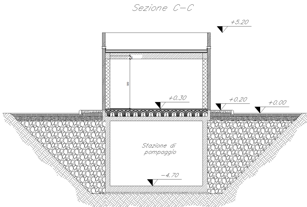
Figura 2 – Sezione Trasversale
