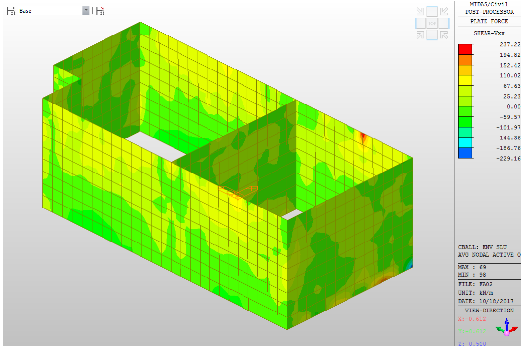
Figura 9 – Vxx: Involuppo SLU
