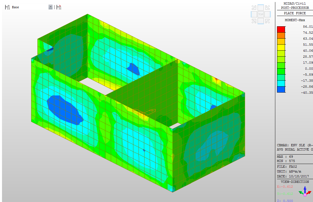
Figura 11 – Mxx: Involuppo SLE
