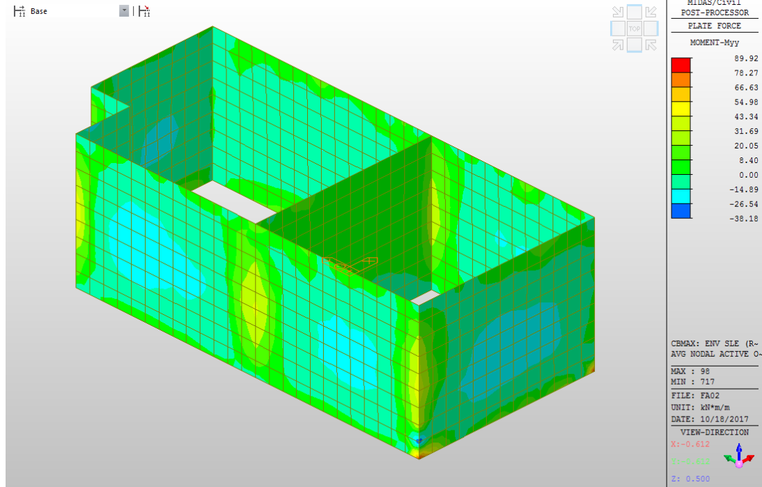
Figura 12 – Myy: Involuppo SLE
