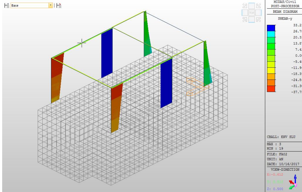
Figura 7-5 Diagramma del taglio V_y – COMB_INV_SLU.
