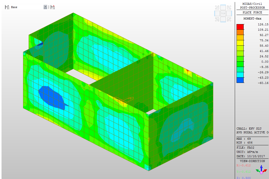
Figura 7 – Mxx: Inviluppo SLU
