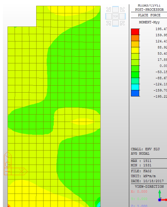
Figura 13 – Myy: Involuppo SLU
