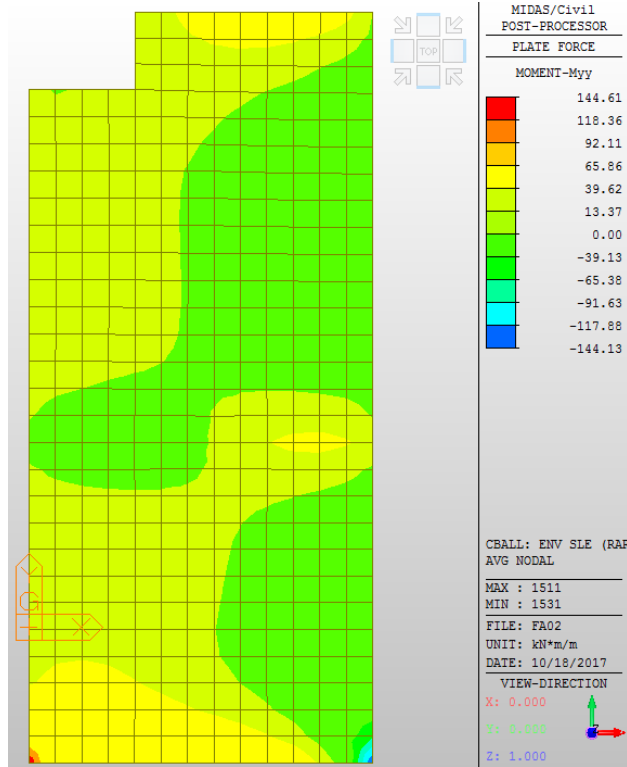
Figura 18 – Myy: Involuppo SLE
