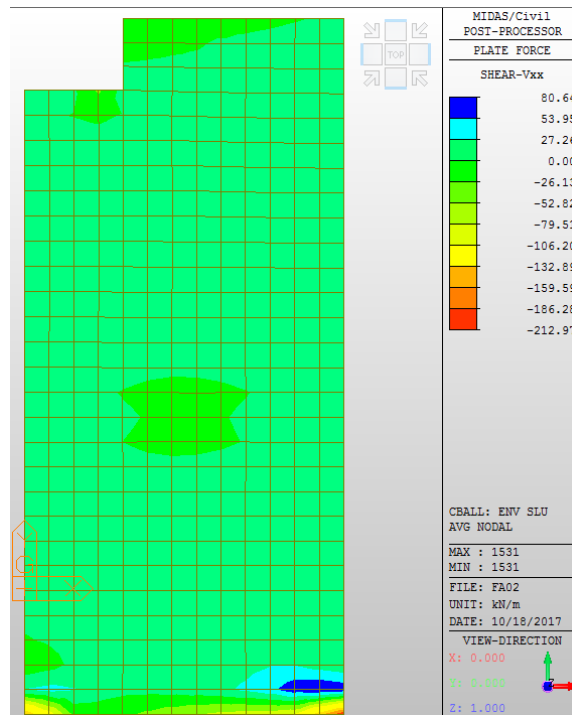
Figura 16 – Vxx: Inviluppo SLU
