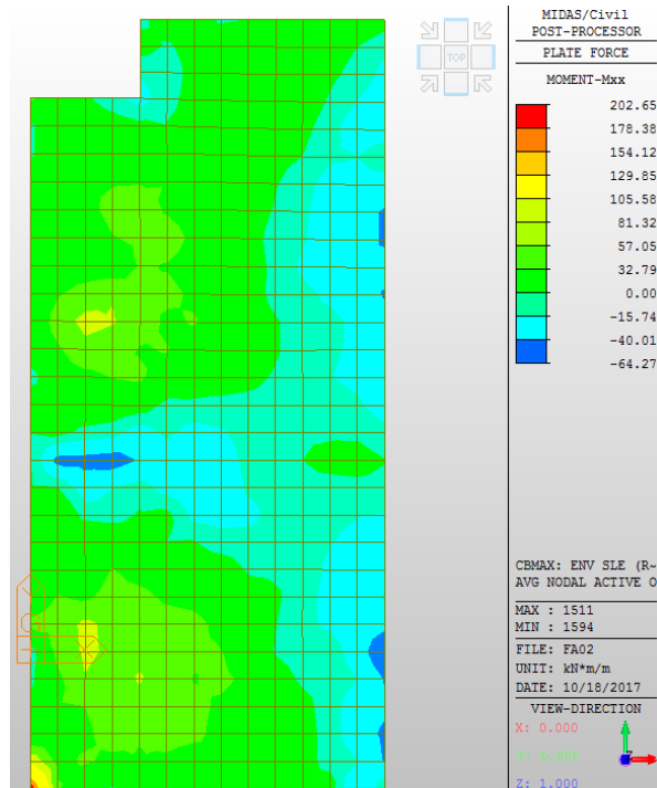
Figura 17 – Mxx: Involuppo SLE
