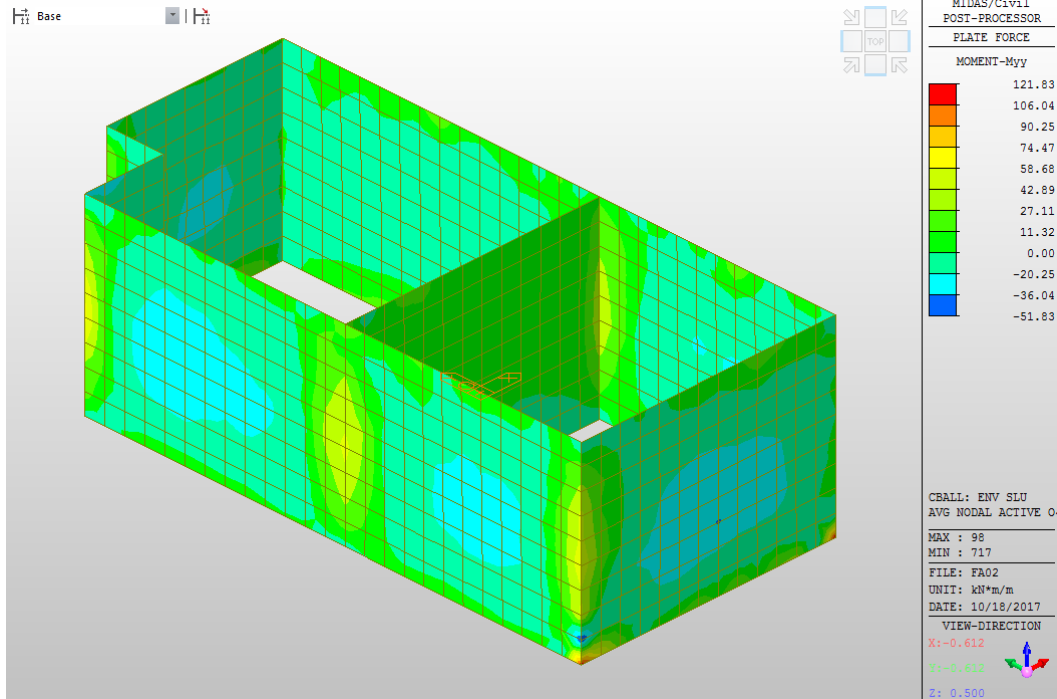
Figura 8 – Myy: Involuppo SLU
