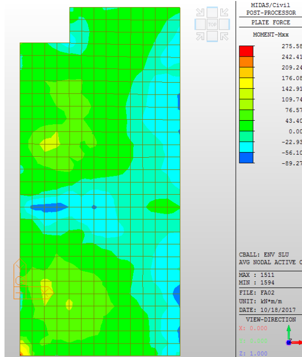
Figura 14 – Mxx: Involuppo SLU
