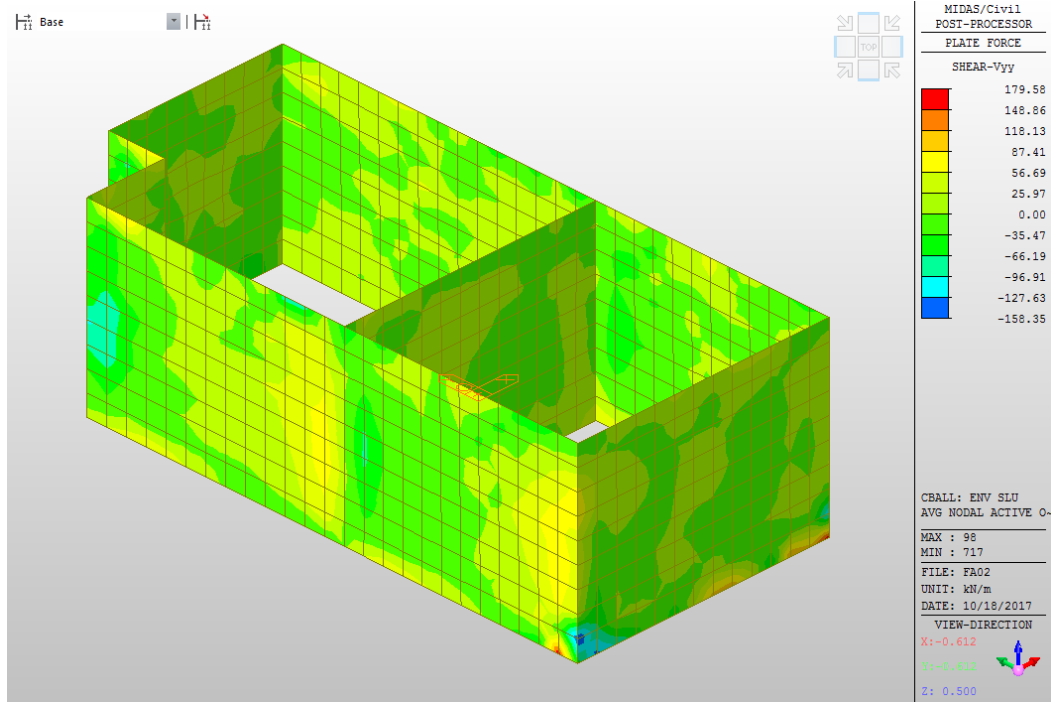
Figura 10 – Vyy: Involuppo SLU
