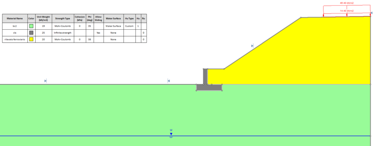
Figura 12 – Dominio di calcolo
