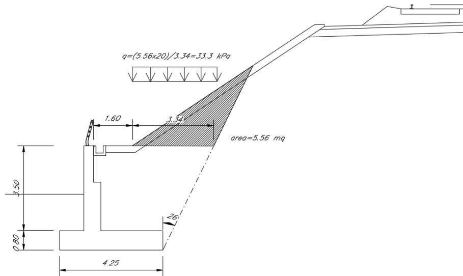
Figura 9 – Sezione muro H=3.5m
