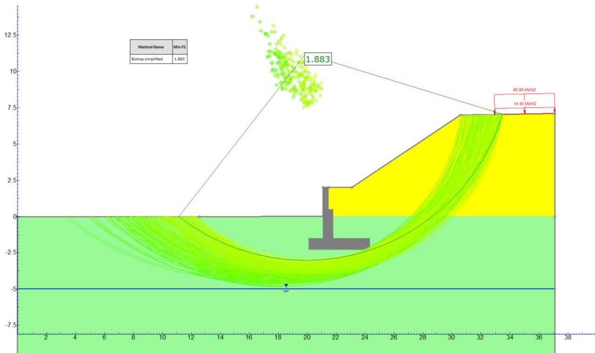
Figura 29 – Superfici di scorrimento-SLU
