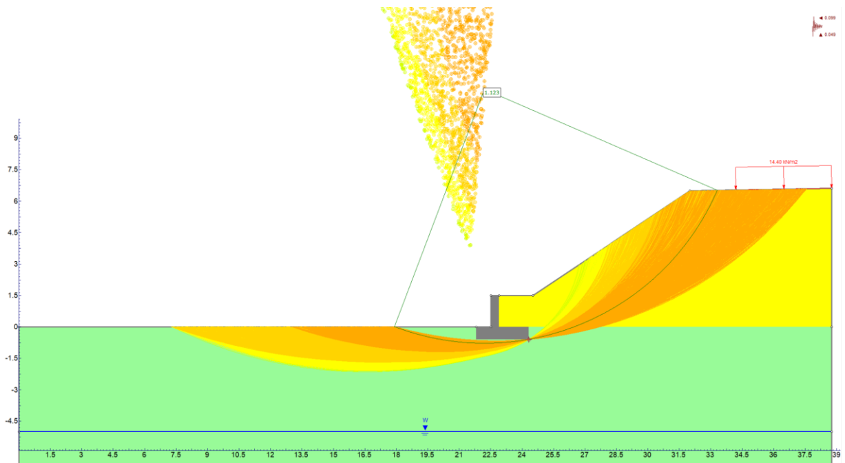
Figura 15 – Superfici di scorrimento-SLV(-)
