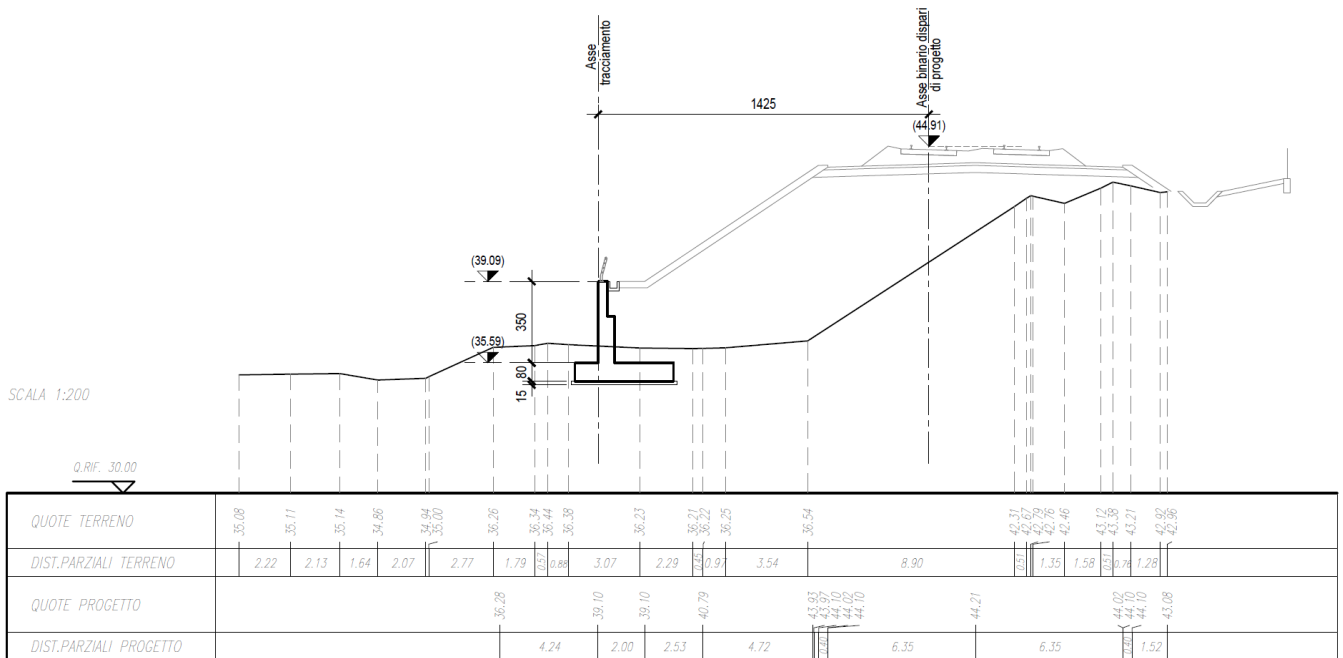
Figura 3 – Sezione trasversale tipo
