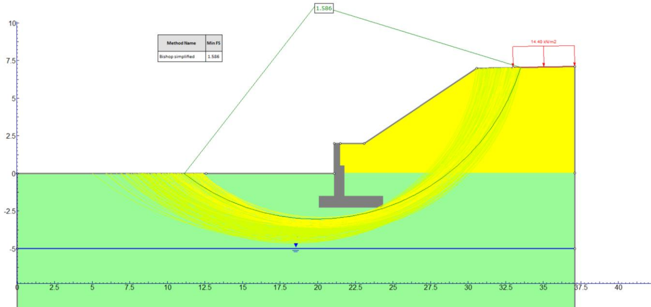
Figura 30 – Superfici di scorrimento-SLV (+)
