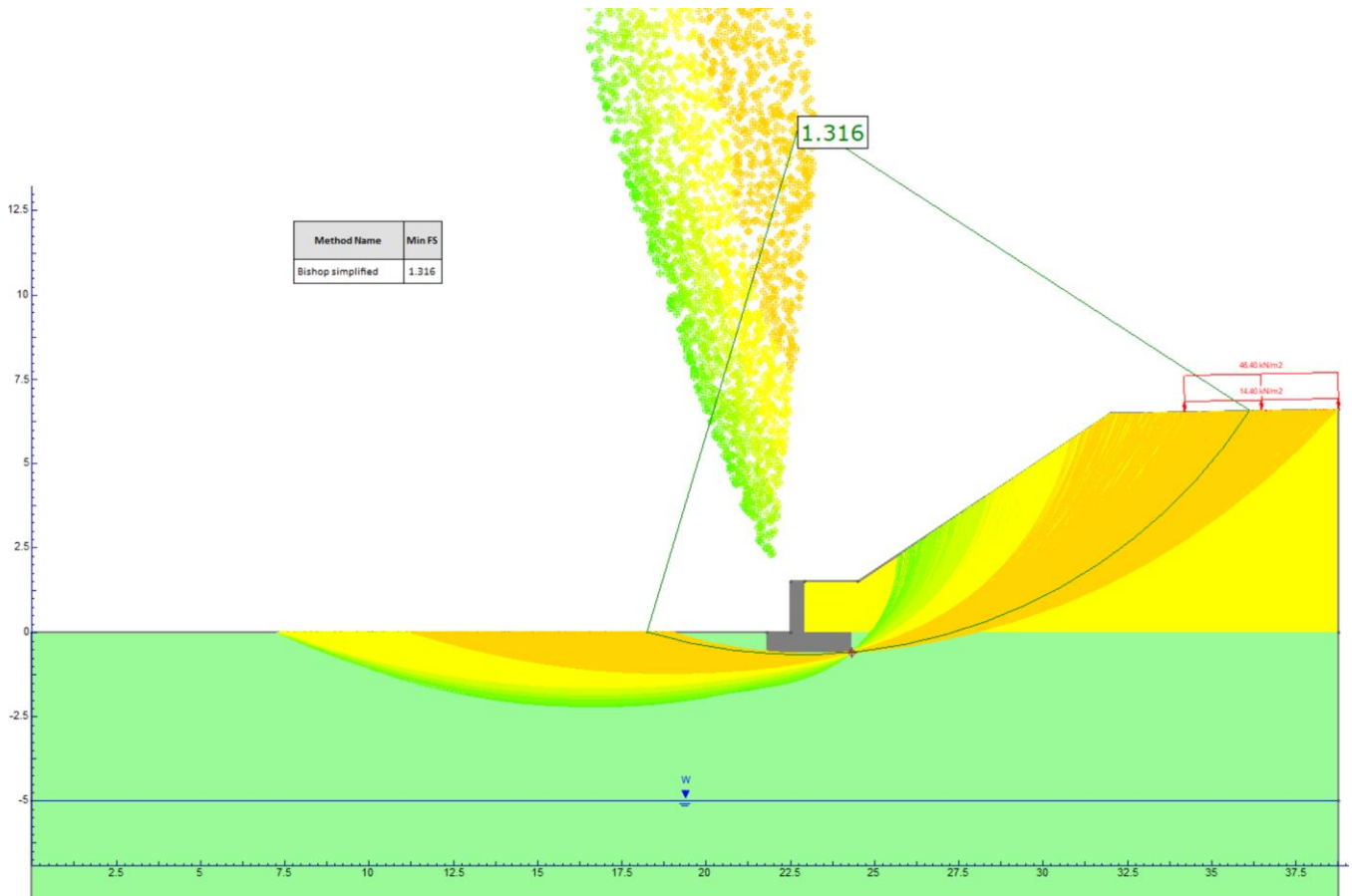
Figura 13 – Superfici di scorrimento-SLU
