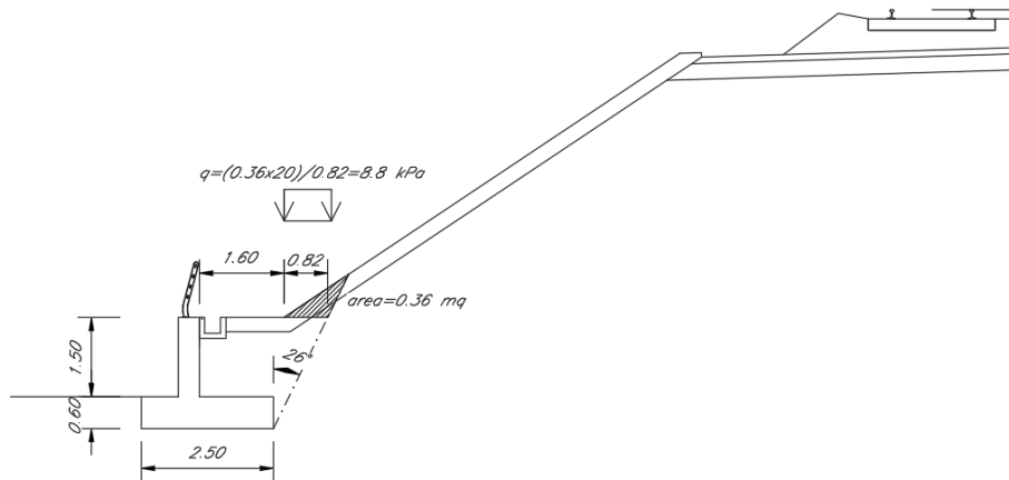
Figura 5 – Sezione muro H=1.5m
