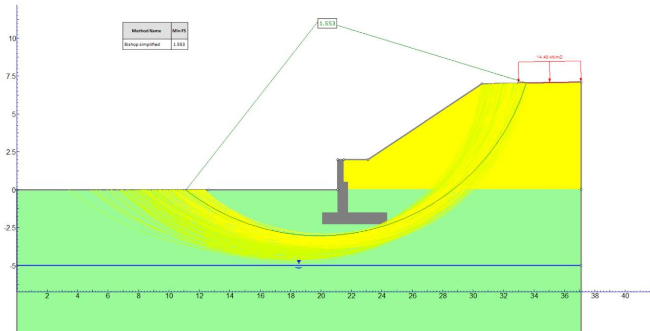
Figura 31 – Superfici di scorrimento-SLV(-)
