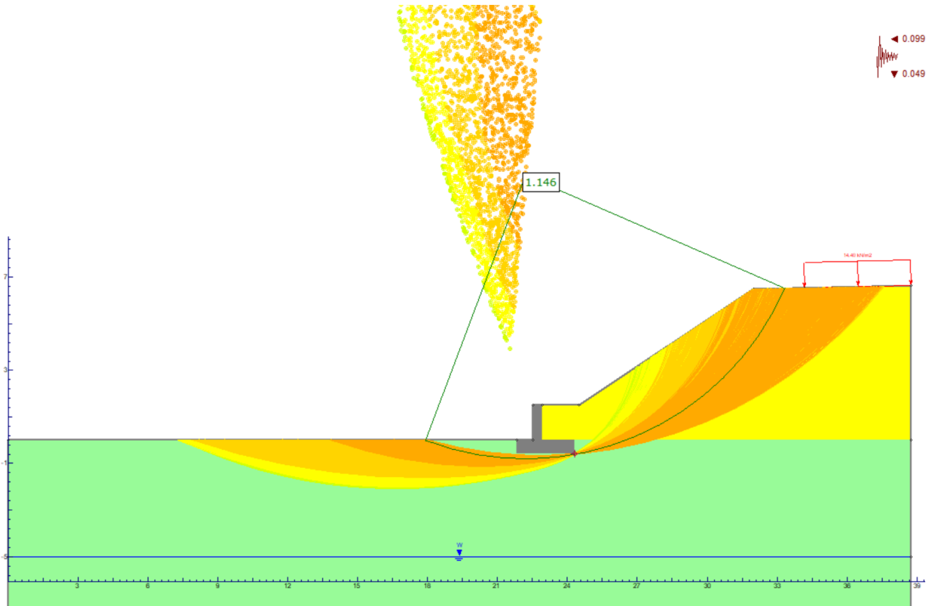
Figura 14 – Superfici di scorrimento-SLV (+)
