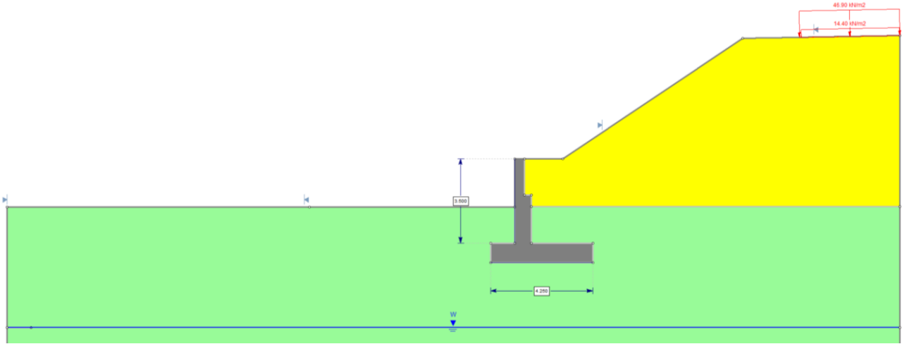
Figura 28 – Dominio di calcolo
