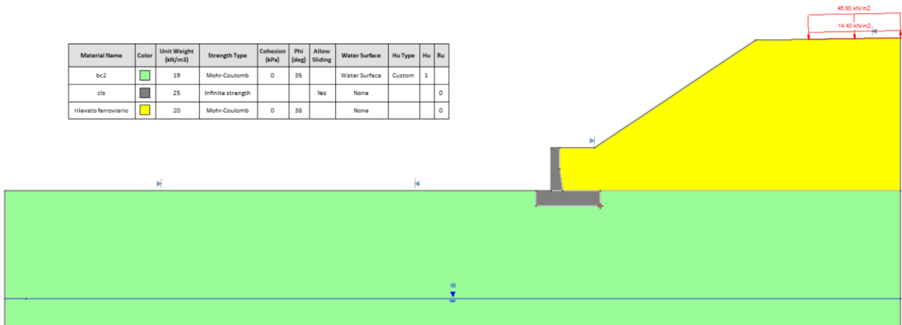
Figura 16 – Dominio di calcolo
