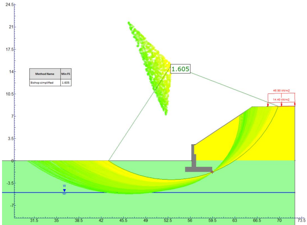
Figura 29 – Superfici di scorrimento-SLU
