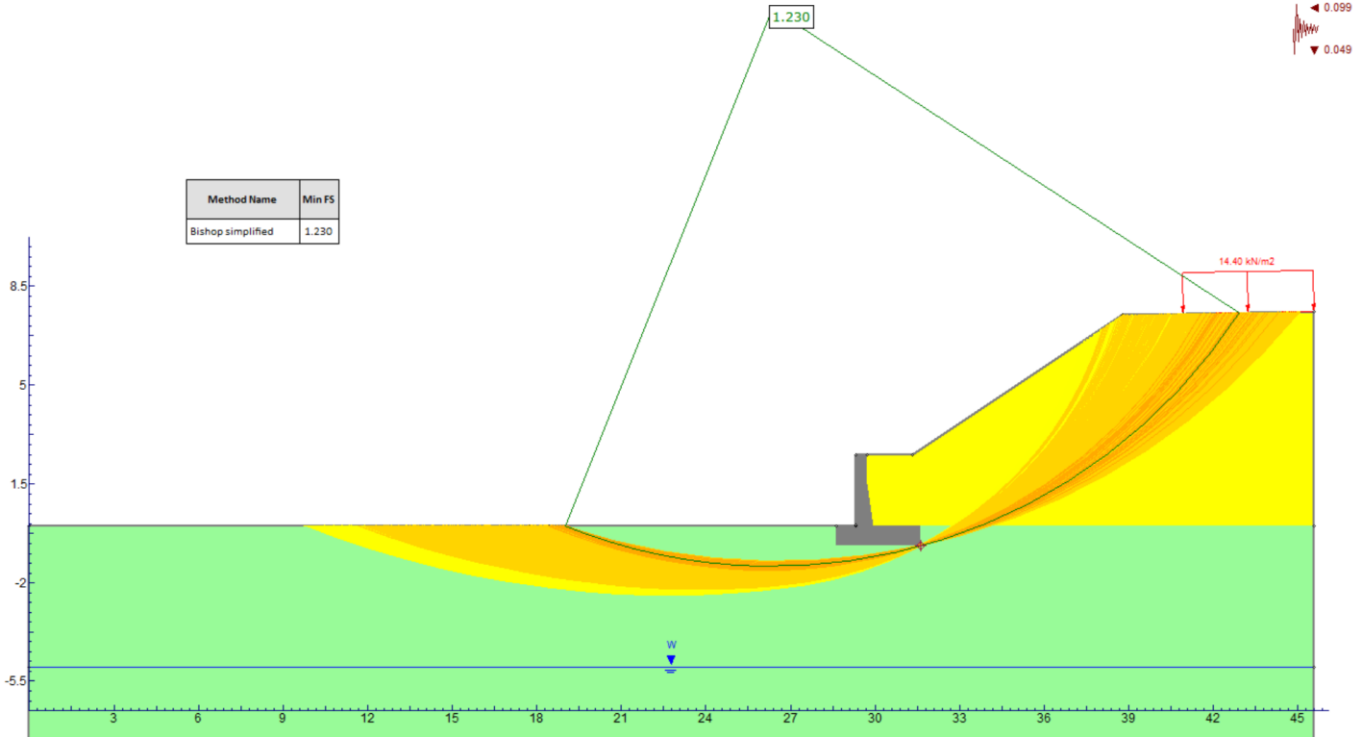
Figura 22 – Superfici di scorrimento-SLV (+)
