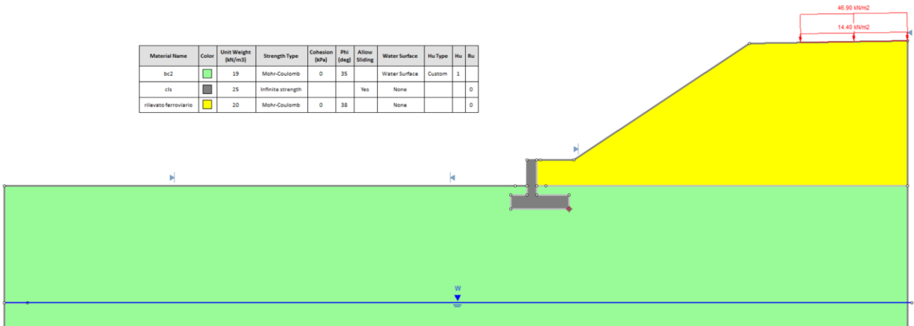
Figura 12 – Dominio di calcolo
