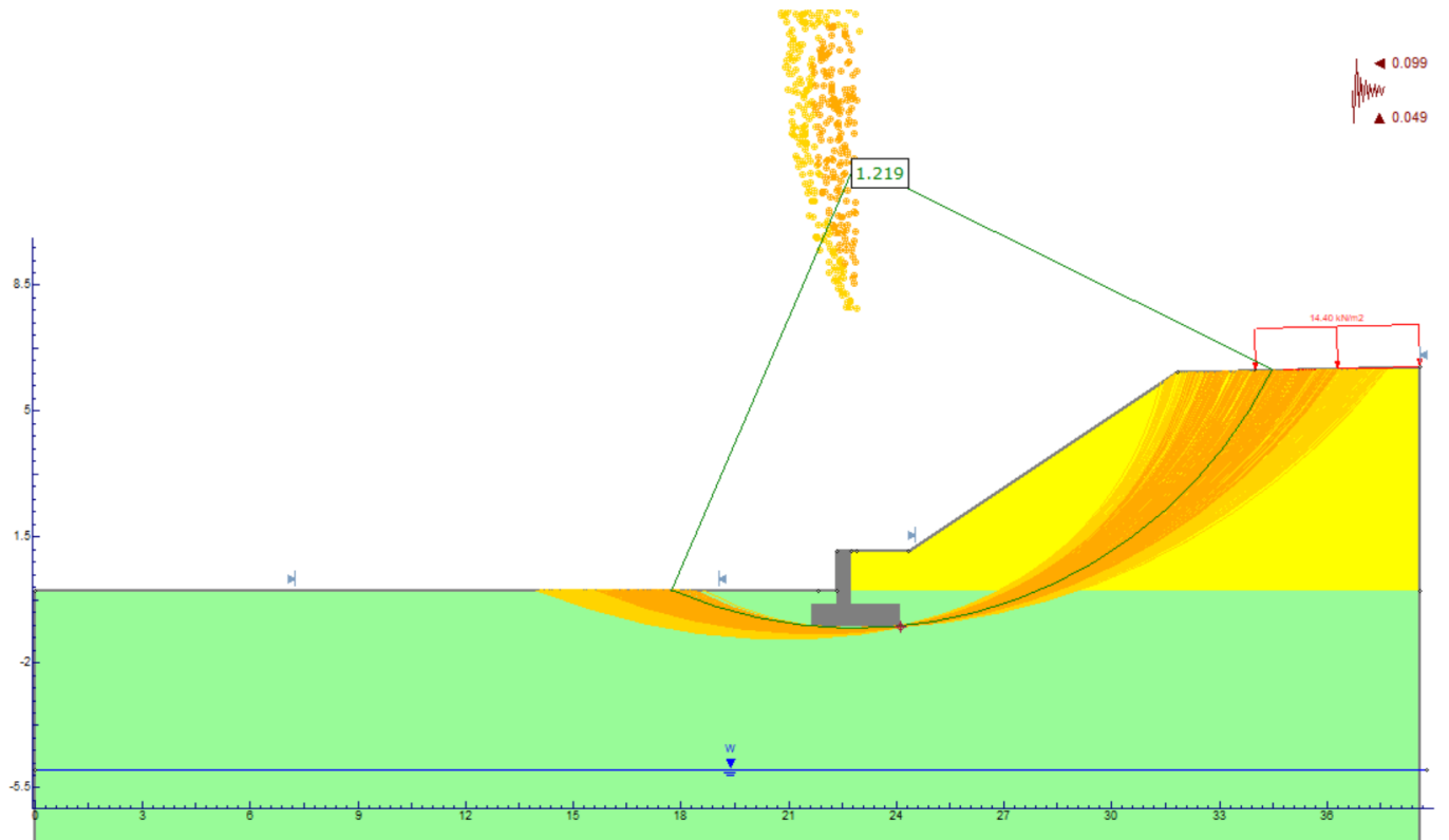
Figura 15 – Superfici di scorrimento-SLV(-)
