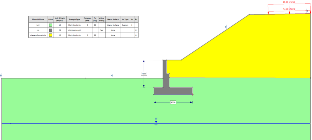
Figura 24 – Dominio di calcolo
