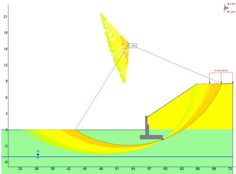
Figura 30 – Superfici di scorrimento-SLV(+)
