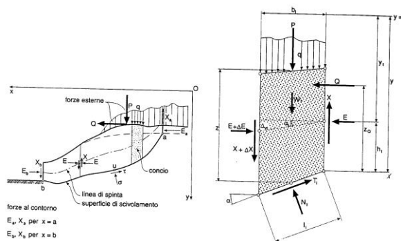
Figura 11 – Schematizzazione di calcolo del metodo delle strisce
