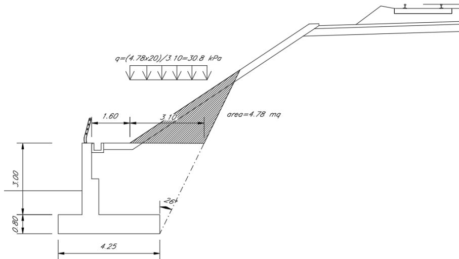
Figura 8 - Sezione muro H=3.0m
