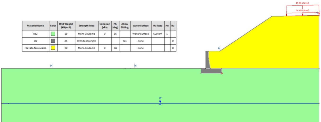
Figura 20 – Dominio di calcolo
