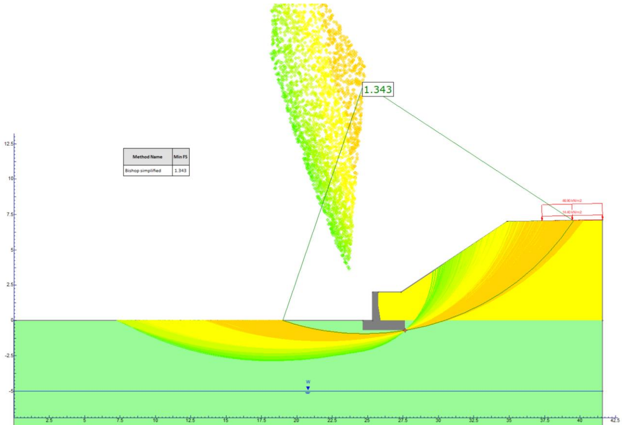
Figura 17 – Superfici di scorrimento-SLU
