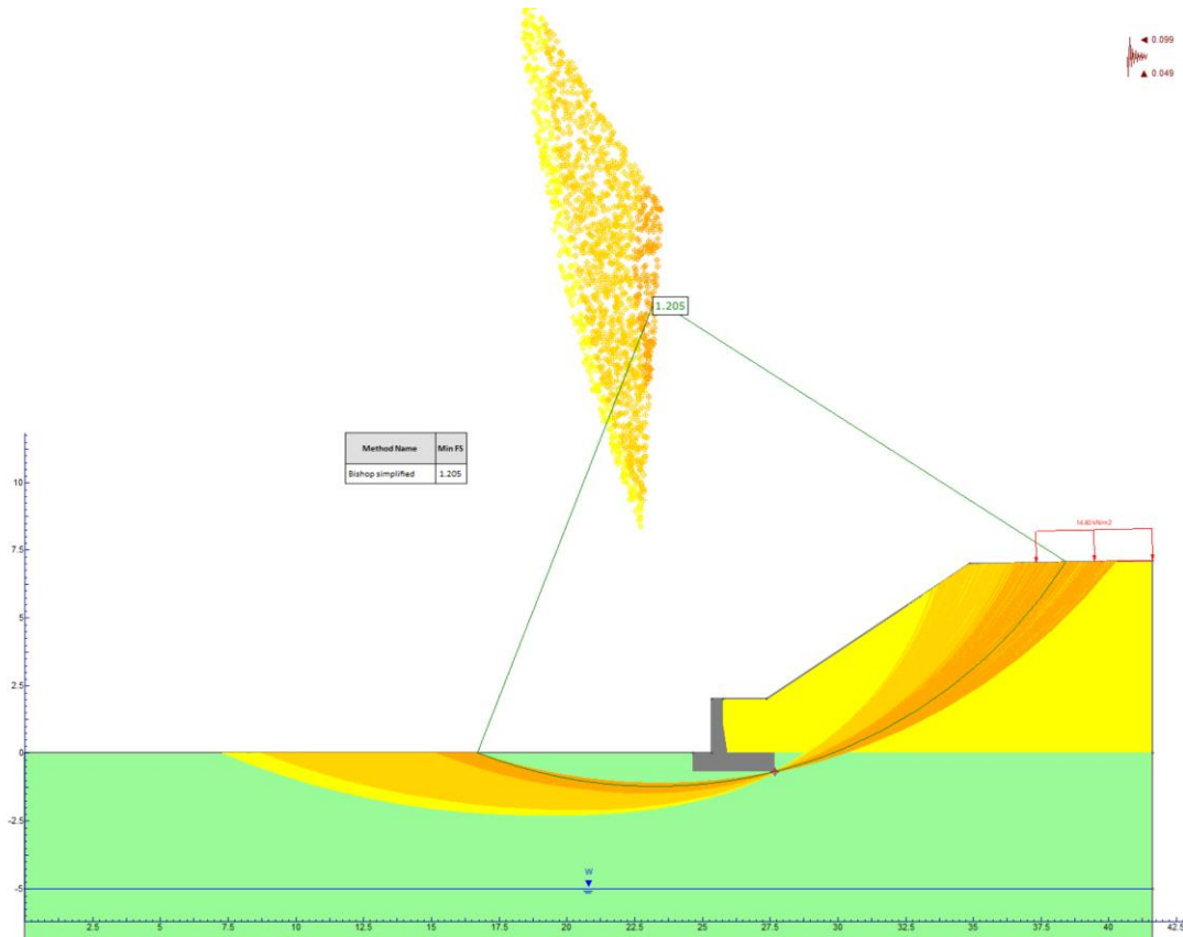
Figura 19 – Superfici di scorrimento-SLV(-)
