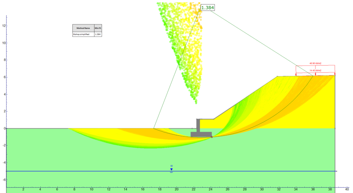
Figura 13 – Superfici di scorrimento-SLU
