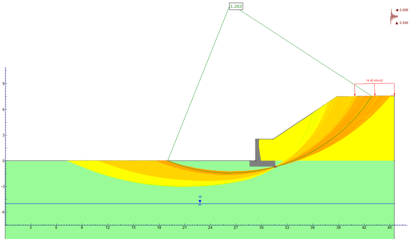
Figura 23 – Superfici di scorrimento-SLV(-)
