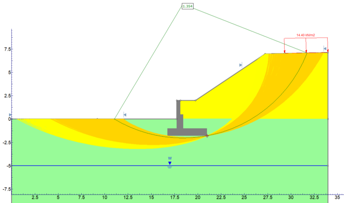
Figura 27 – Superfici di scorrimento-SLV(-)
