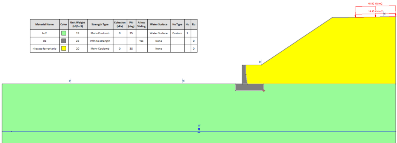
Figura 16 – Dominio di calcolo
