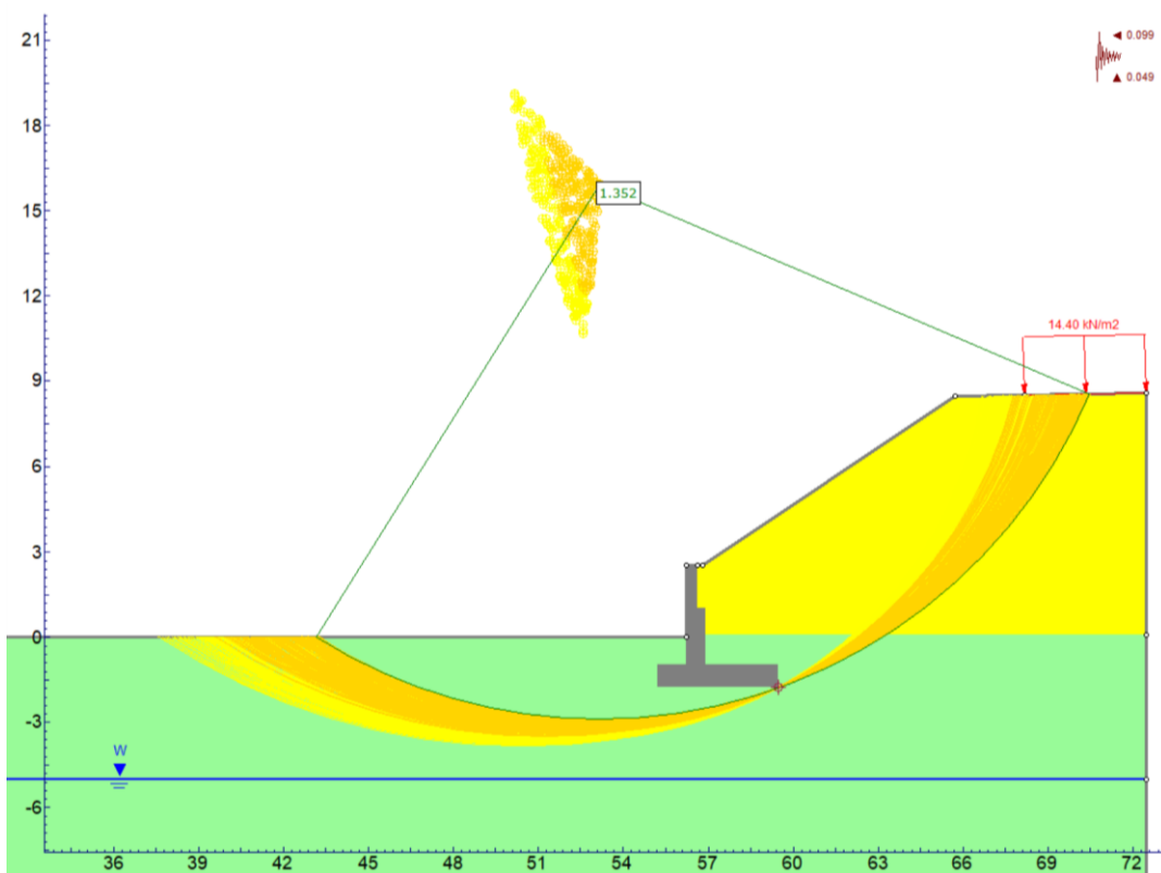
Figura 31 – Superfici di scorrimento-SLV(-)
