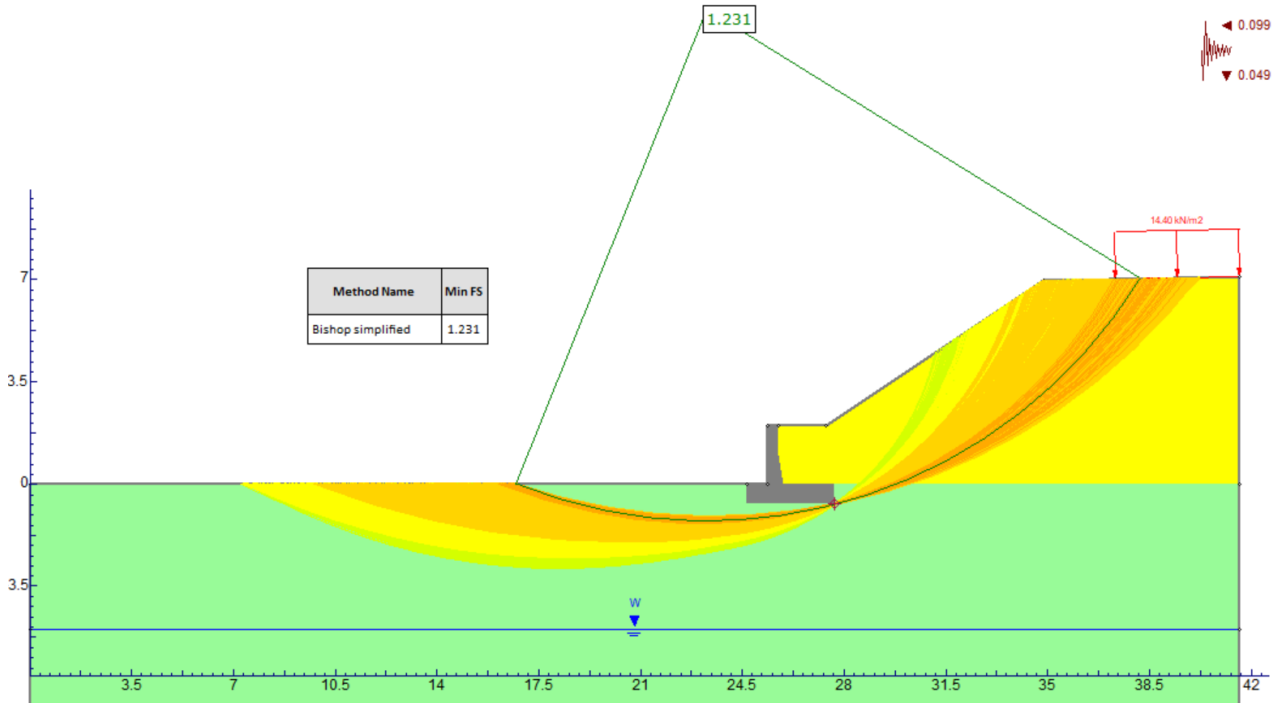
Figura 18 – Superfici di scorrimento-SLV(+)
