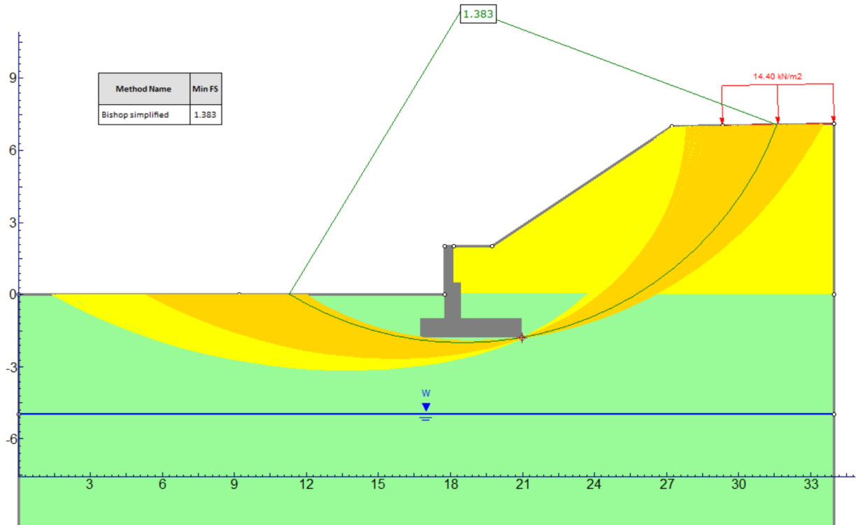
Figura 26 – Superfici di scorrimento-SLV (+)
