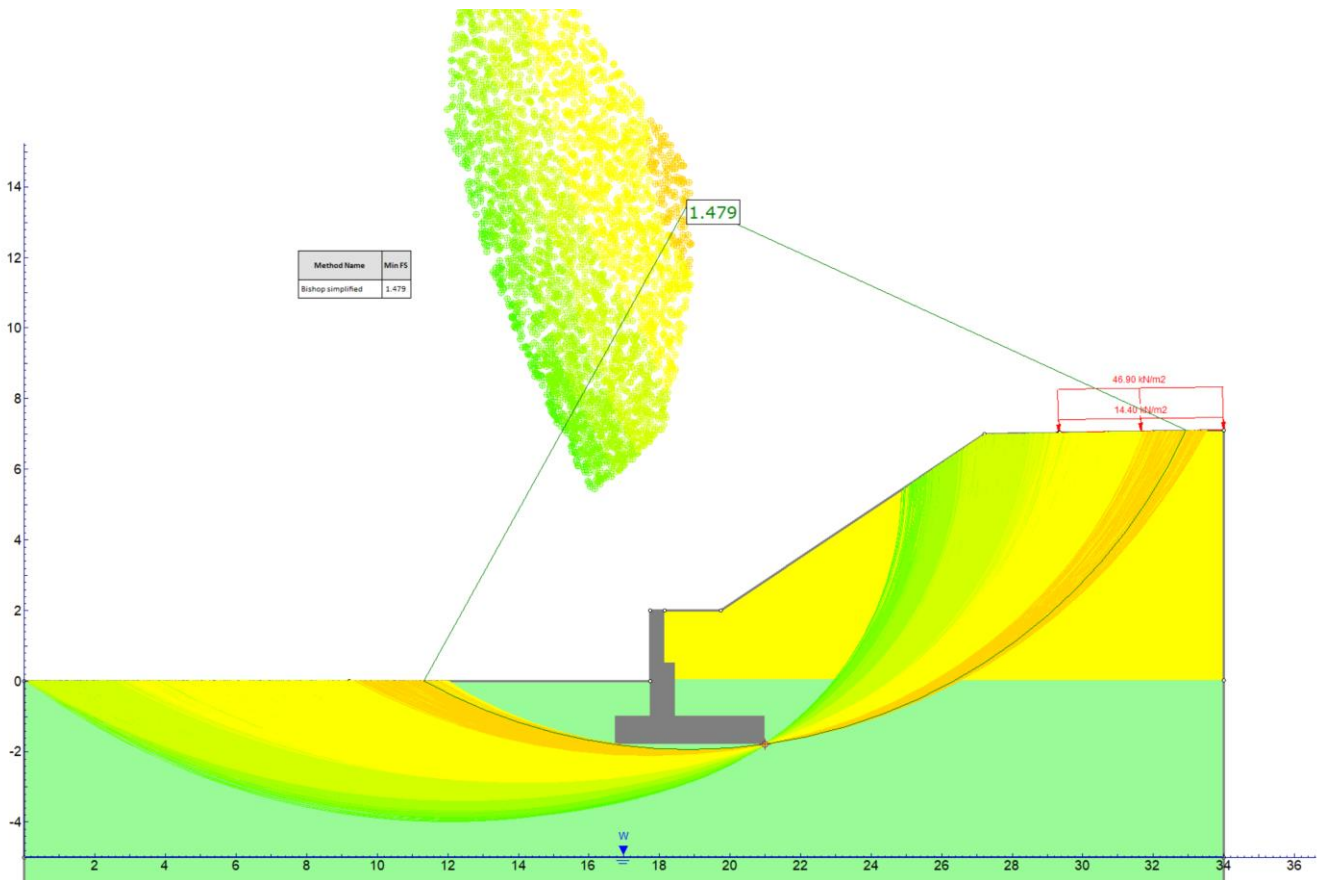
Figura 25 – Superfici di scorrimento-SLU
