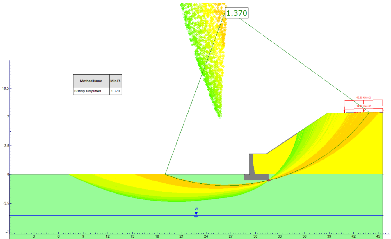
Figura 21 – Superfici di scorrimento-SLU
