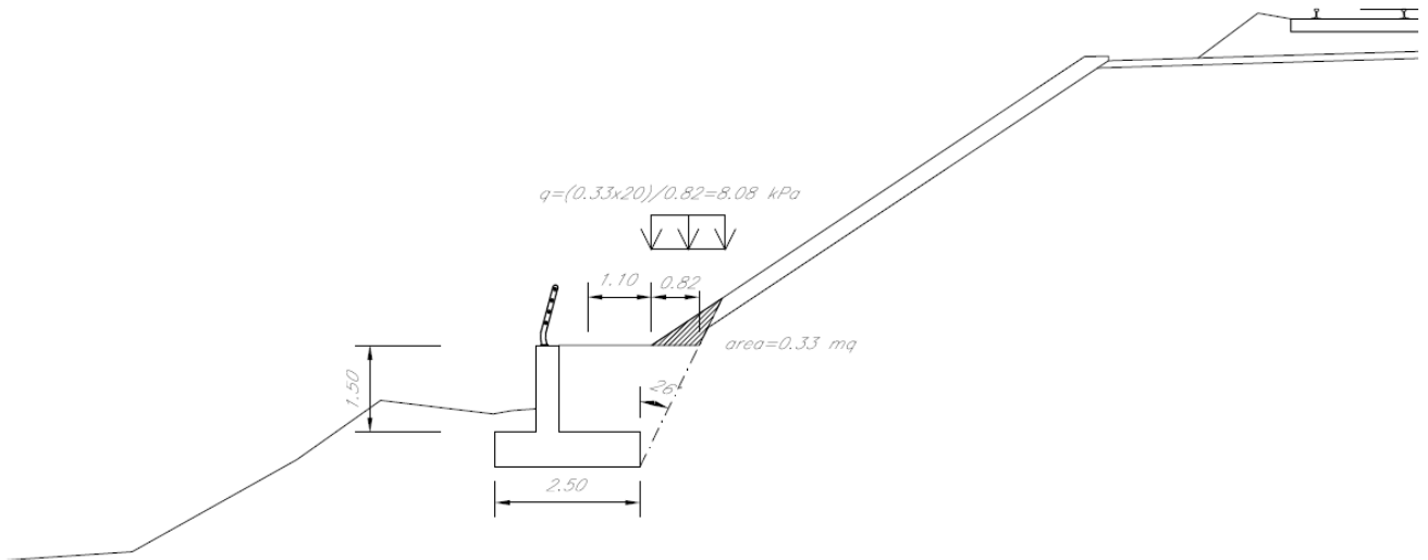
Figura 5 – Sezione muro H=1.5m
