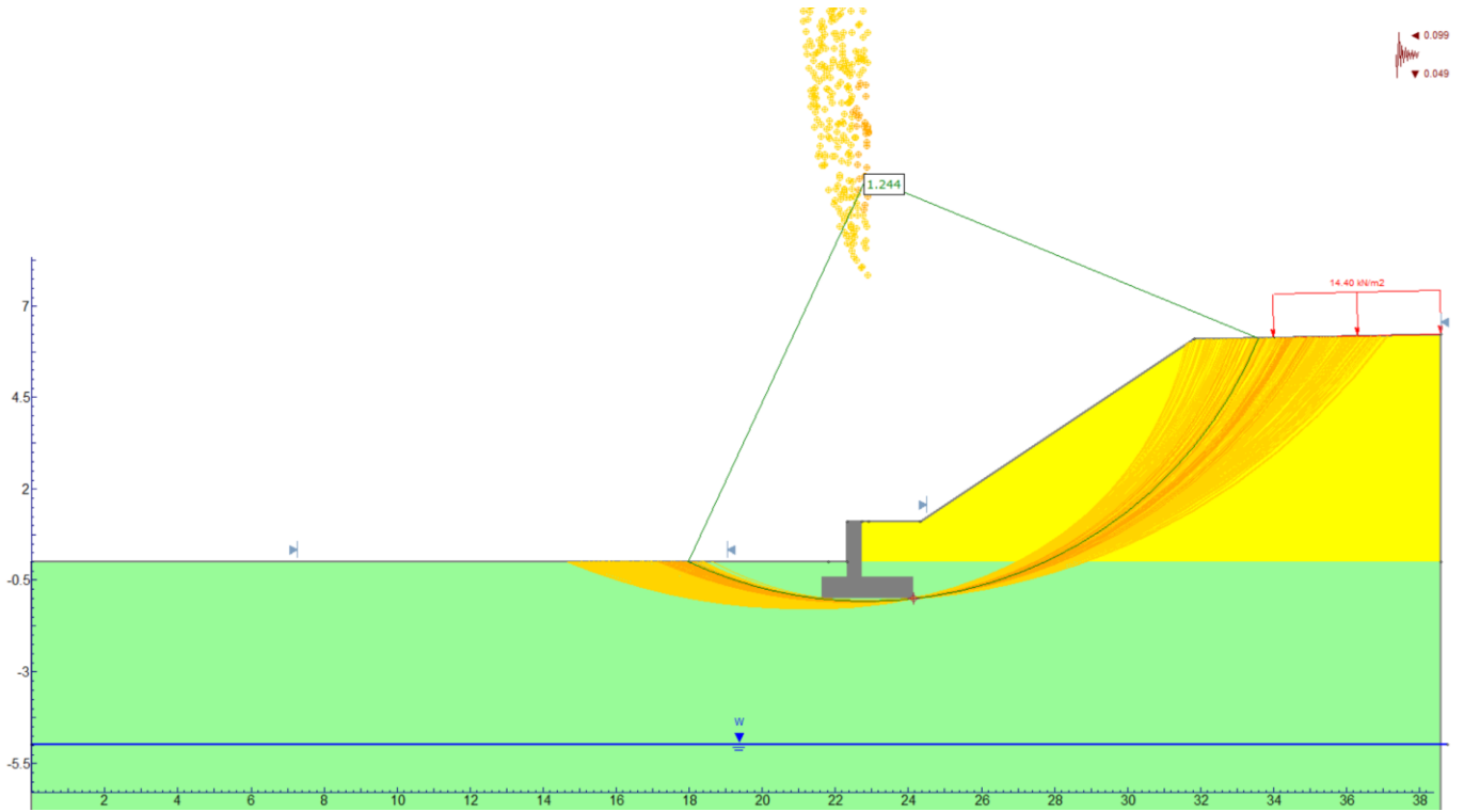
Figura 14 – Superfici di scorrimento-SLV (+)
