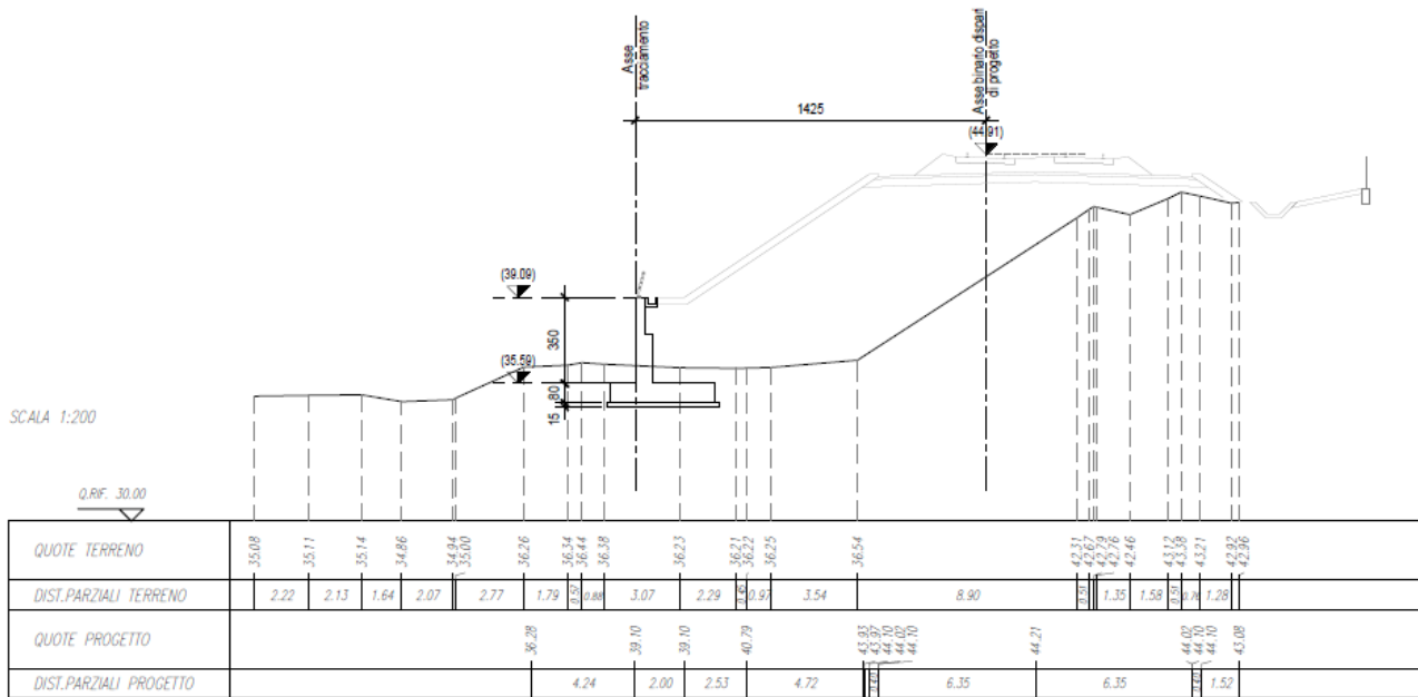
Figura 3 – Sezione trasversale tipo
