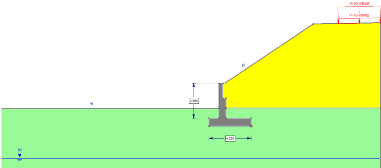
Figura 28 – Dominio di calcolo
