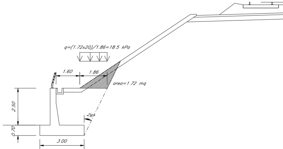
Figura 7 - Sezione muro H=2.5m
