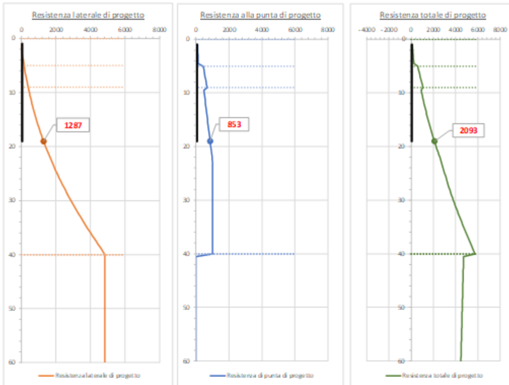
DIAGRAMMI CAPACITA' PORTANTE A FORZE ASSIALI DI COMPRESIONE
