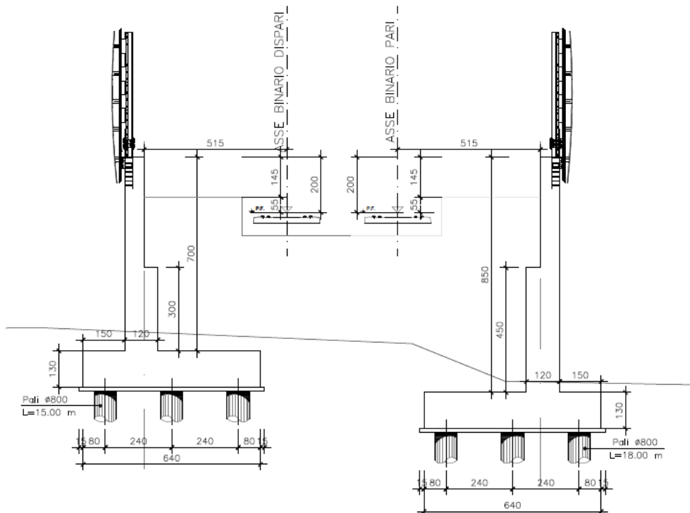
Figura 5 – Sezione trasversale tipo
