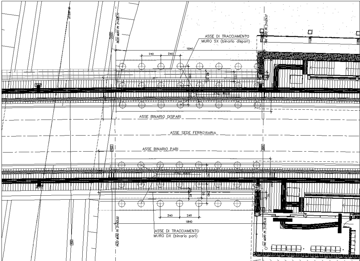
Figura 3 – Pianta Fondazioni
