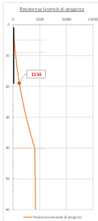
DIAGRAMMA CAPACITA' PORTANTE A FORZE ASSIALI DI TRAZIONE
