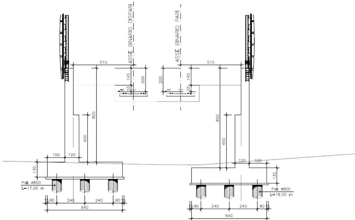
Figura 4 – Sezione trasversale tipo
