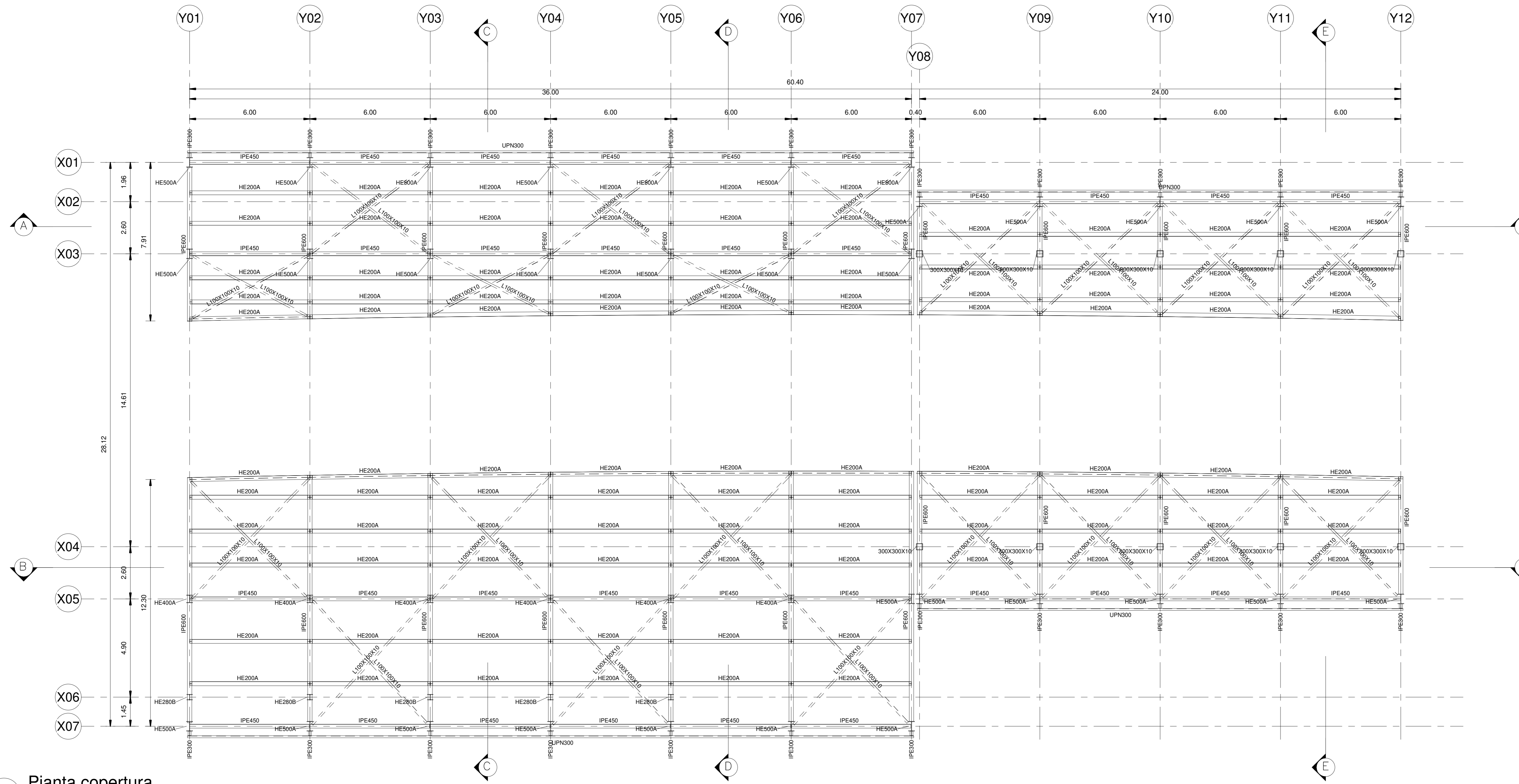
1 Pianta copertura PA.FV.01.0.0.005 1 : 100
