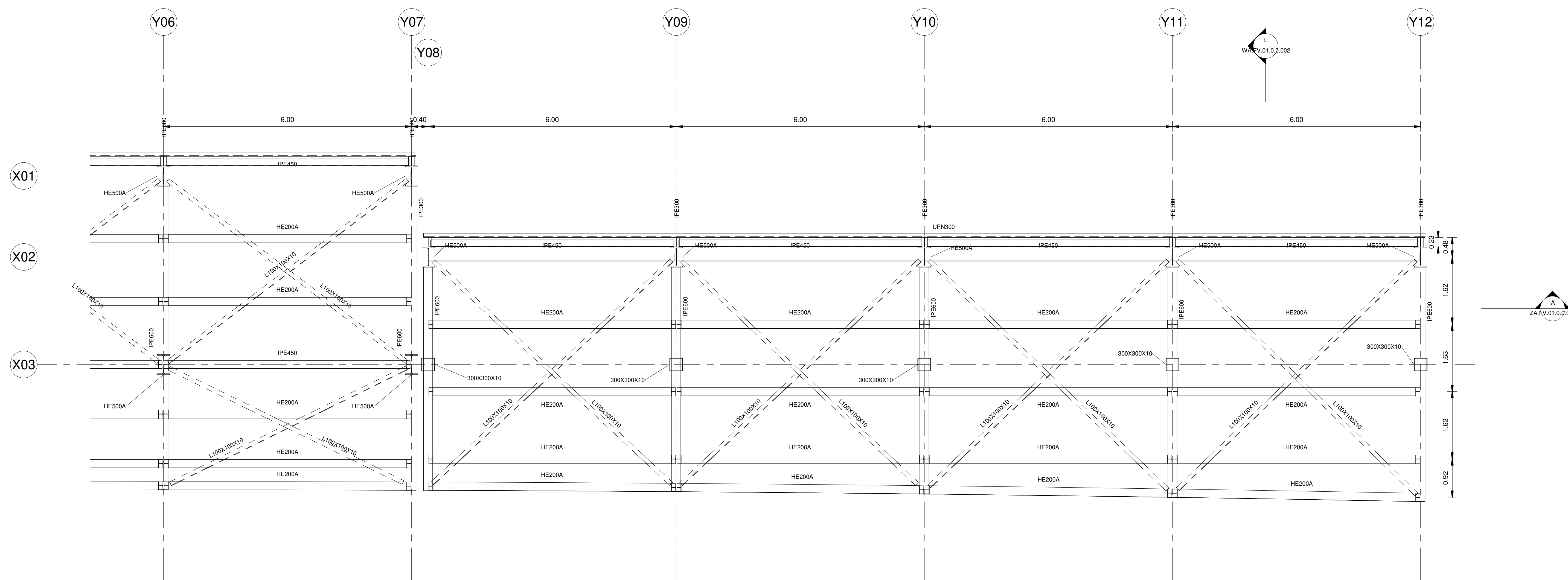
1 Pensilina BD - Pianta copertura PB.FV.01.0.0.002 1:50
