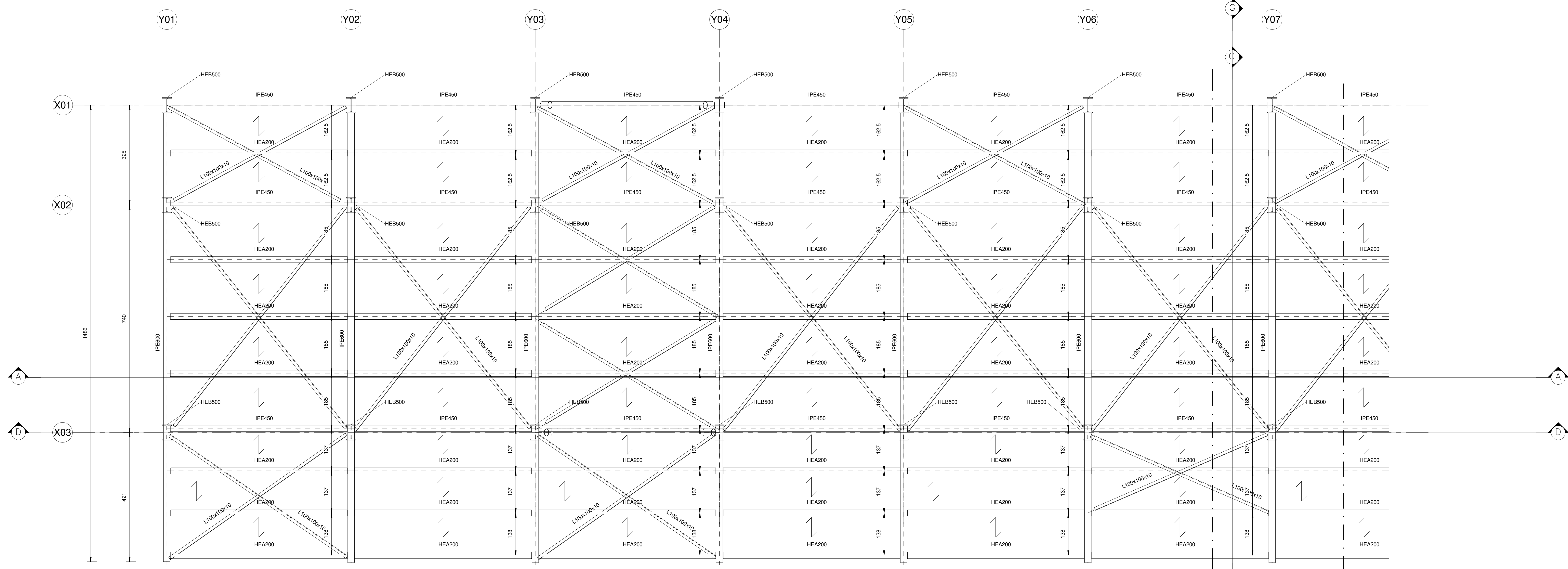
1 Pensilina Fabricato viaggiatori - Pianta copertura 1 : 50
