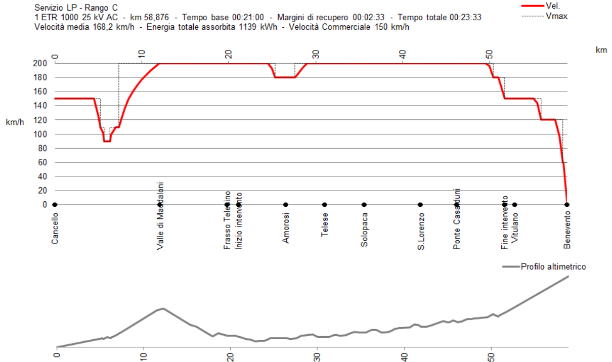
Figura 5: Diagramma spazio-velocità per il servizio Lunga percorrenza con ETR1000, nel senso di marcia Canello-Benevento.
