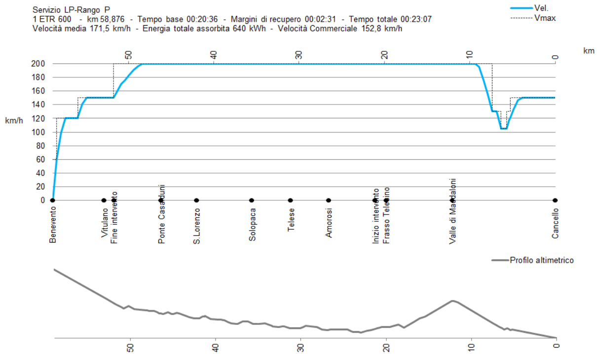
Figura 8: Diagramma spazio-velocità per il servizio Lunga percorrenza con ETR600, nel senso di marcia Benevento-Canello.
