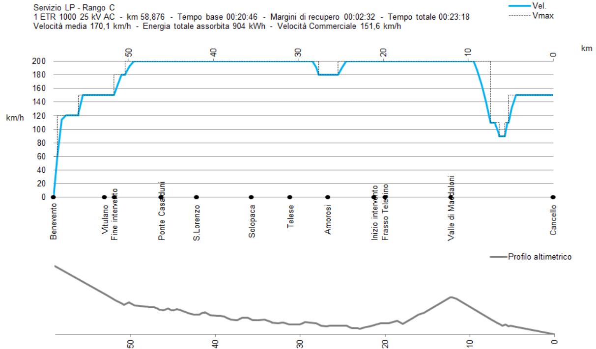
Figura 6: Diagramma spazio-velocità per il servizio Lunga percorrenza con ETR1000, nel senso di marcia Benevento- Canello.
