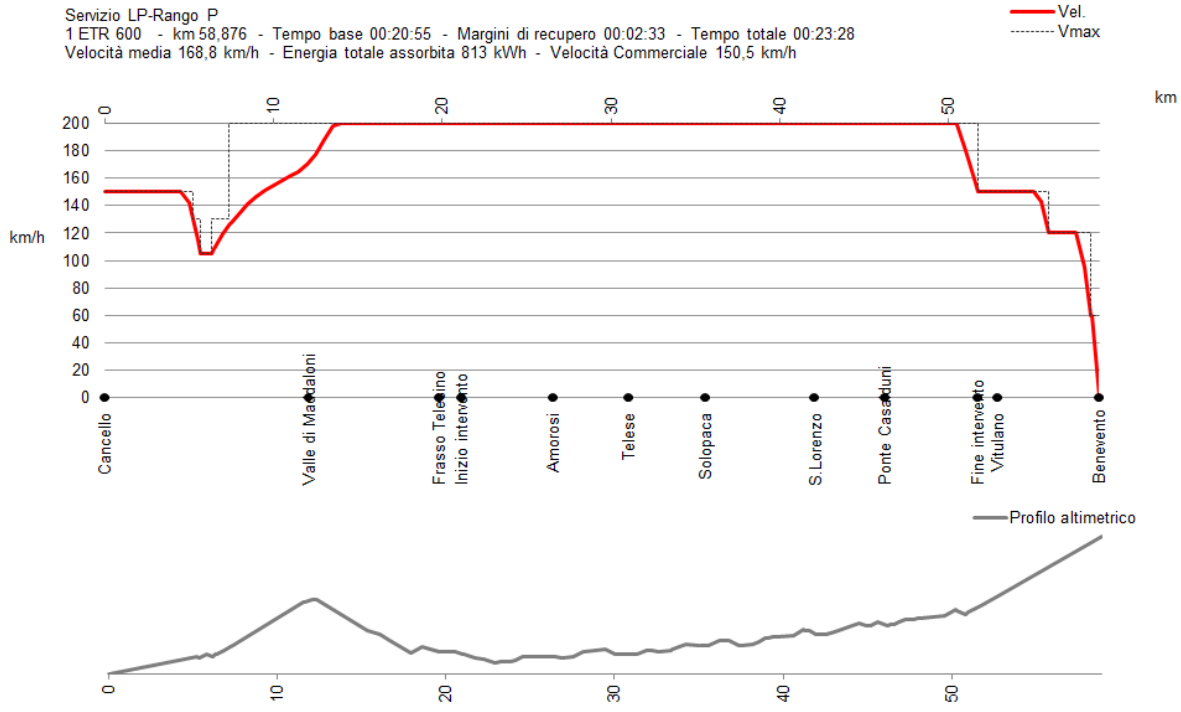
Figura 7: Diagramma spazio-velocità per il servizio Lunga percorrenza con ETR600, nel senso di marcia Canello-Benevento.
