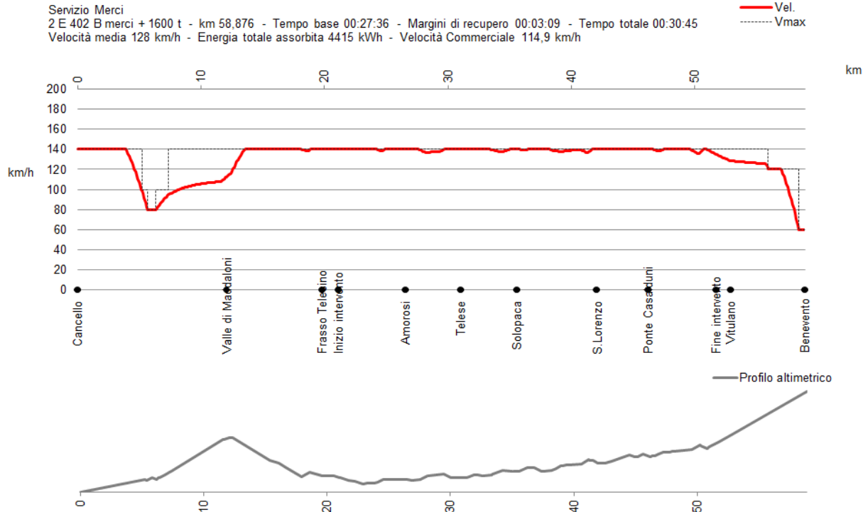
Figura 11: Diagramma spazio-velocità per il servizio merci, nel senso di marcia Canello-Benevento.
