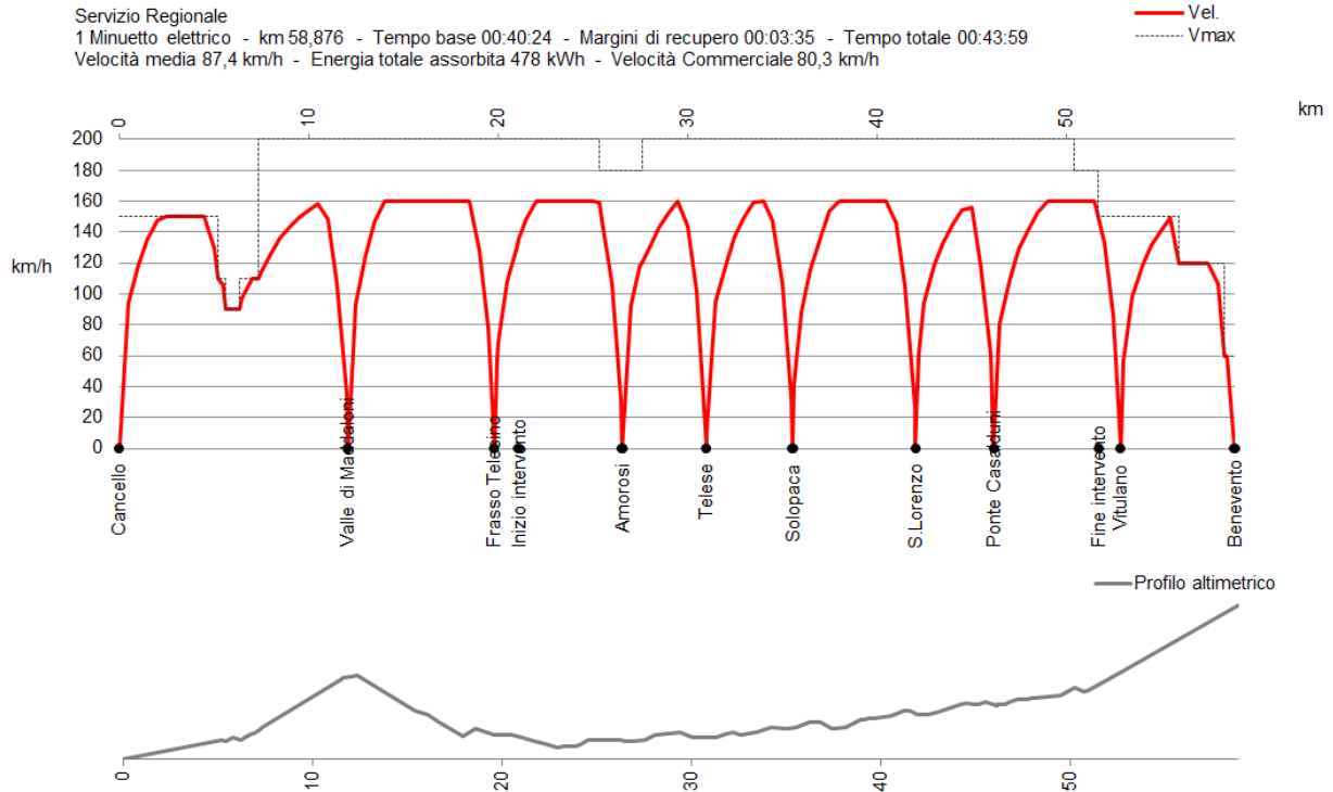
Figura 9: Diagramma spazio-velocità per il servizio regionale, nel senso di marcia Canello-Benevento.
