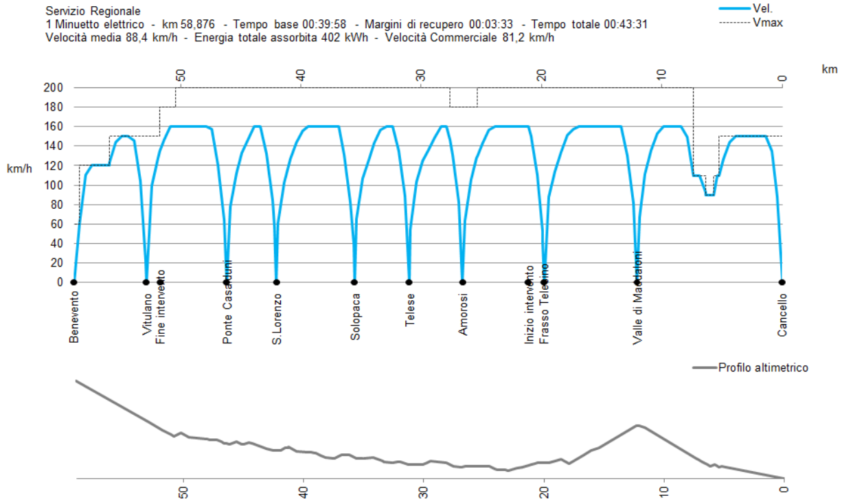
Figura 10: Diagramma spazio-velocità per il servizio regionale, nel senso di marcia Benevento-Canello.
