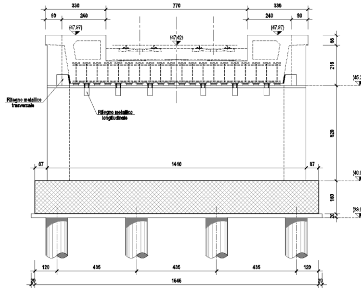
Figura 3 – Spalla S1
