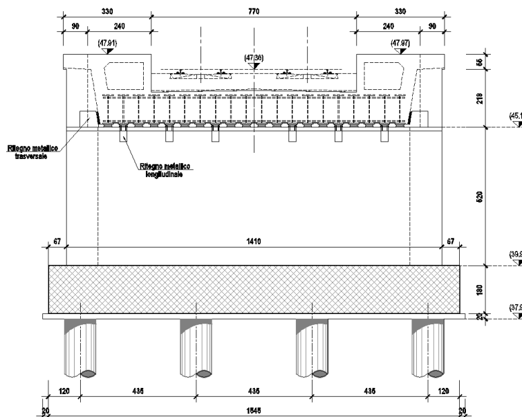
Figura 4 – Spalla S2
