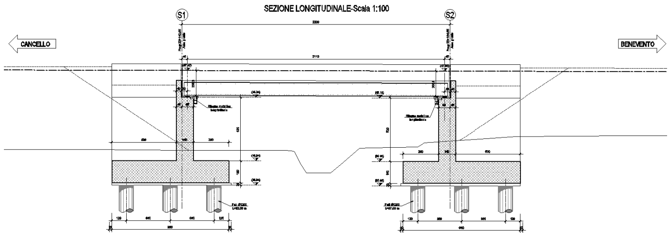
Figura 1 – Sezione Longitudinale
