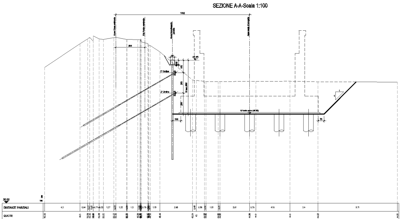
Figura 6 – Opere provvisionali (presidio spalla S1)
