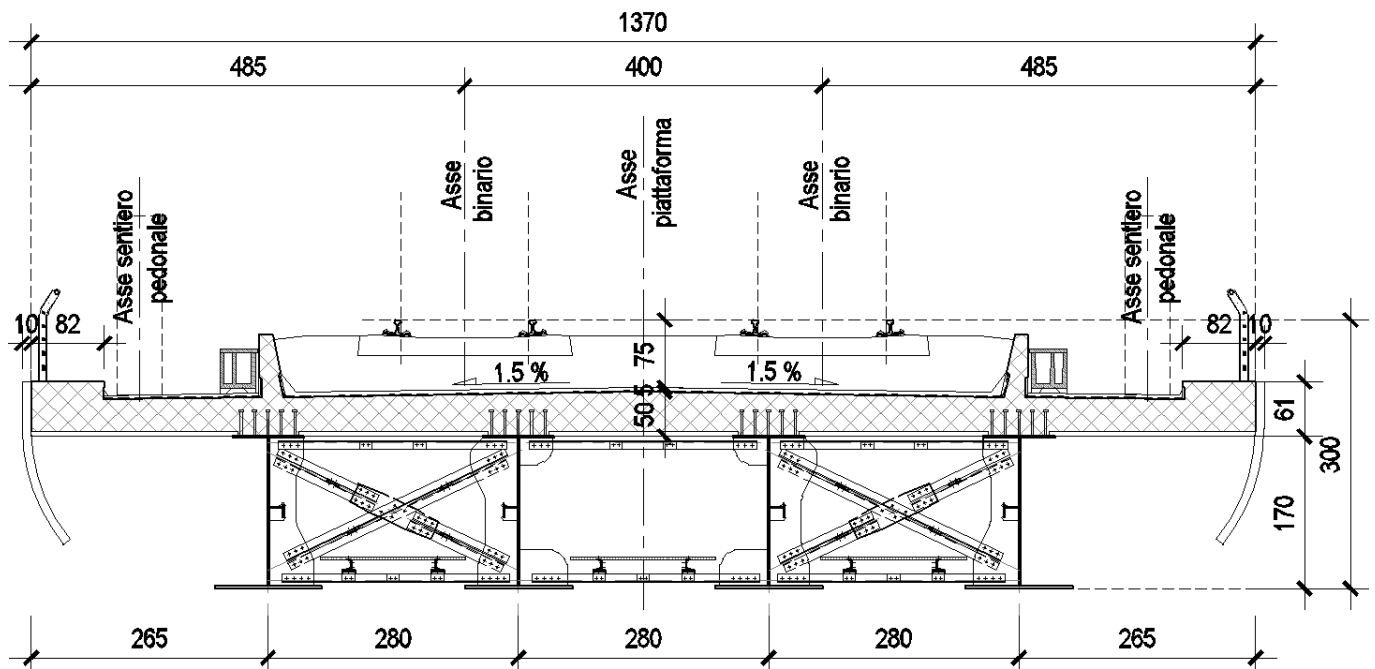
Figura 2 – Impalcato a travatura metallica acciaio-clt
