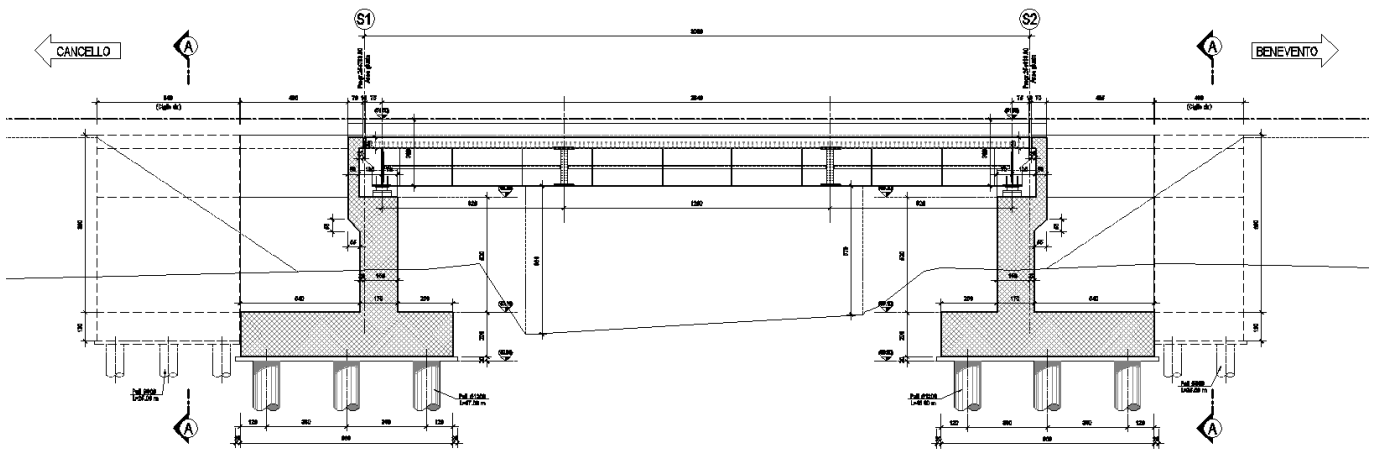
Figura 1 – Sezione Longitudinale
