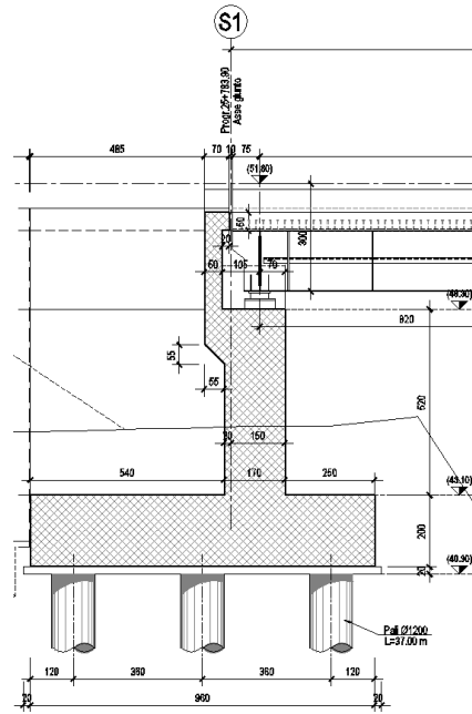
Figura 3 – Spalla S1
