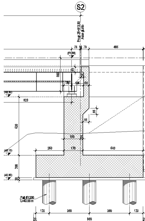
Figura 4 – Spalla S2
