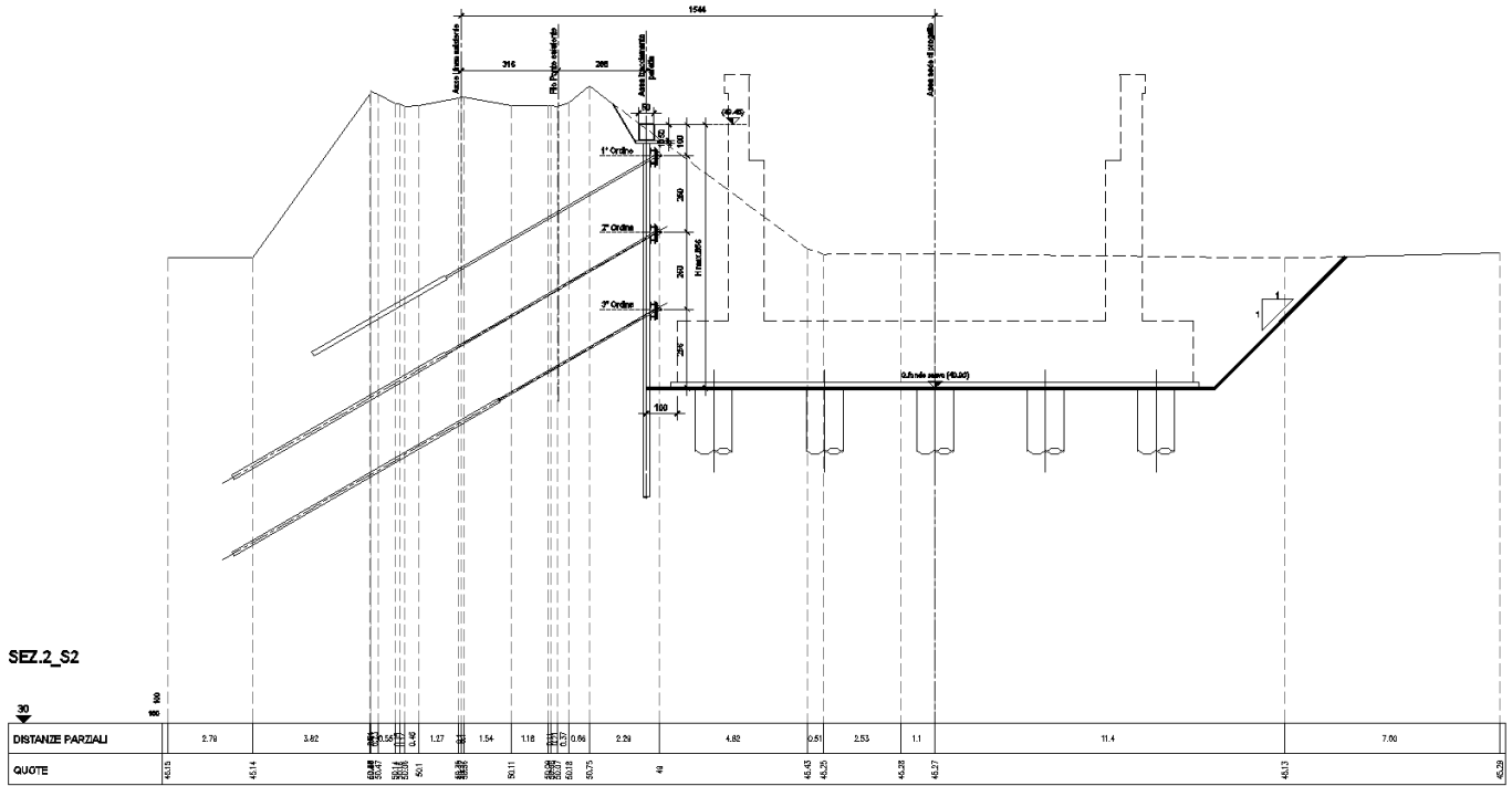
Figura 7 – Opere provvisorie fase II (presidio spalla S2)
