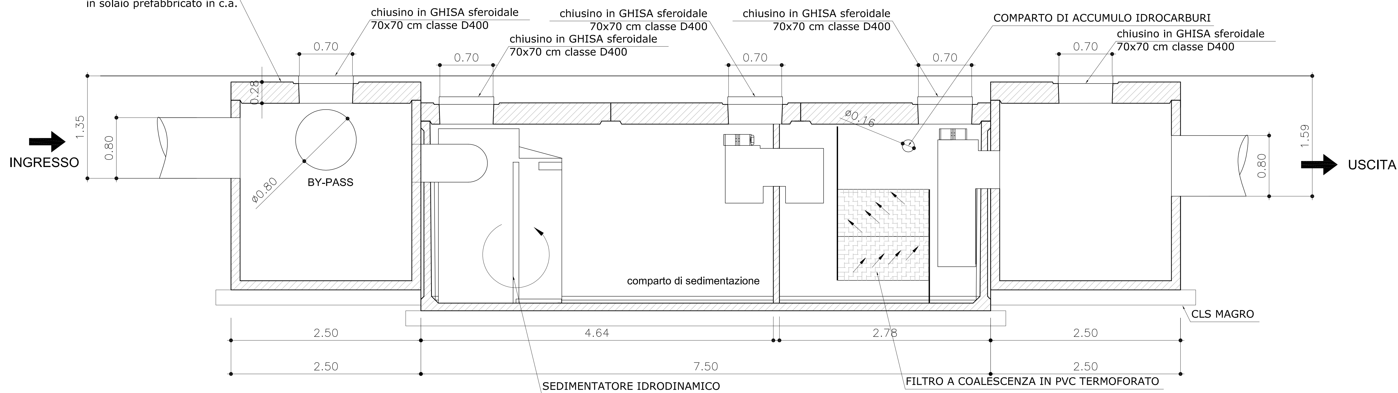
SEZIONE A-A (SCALA 1:25)
