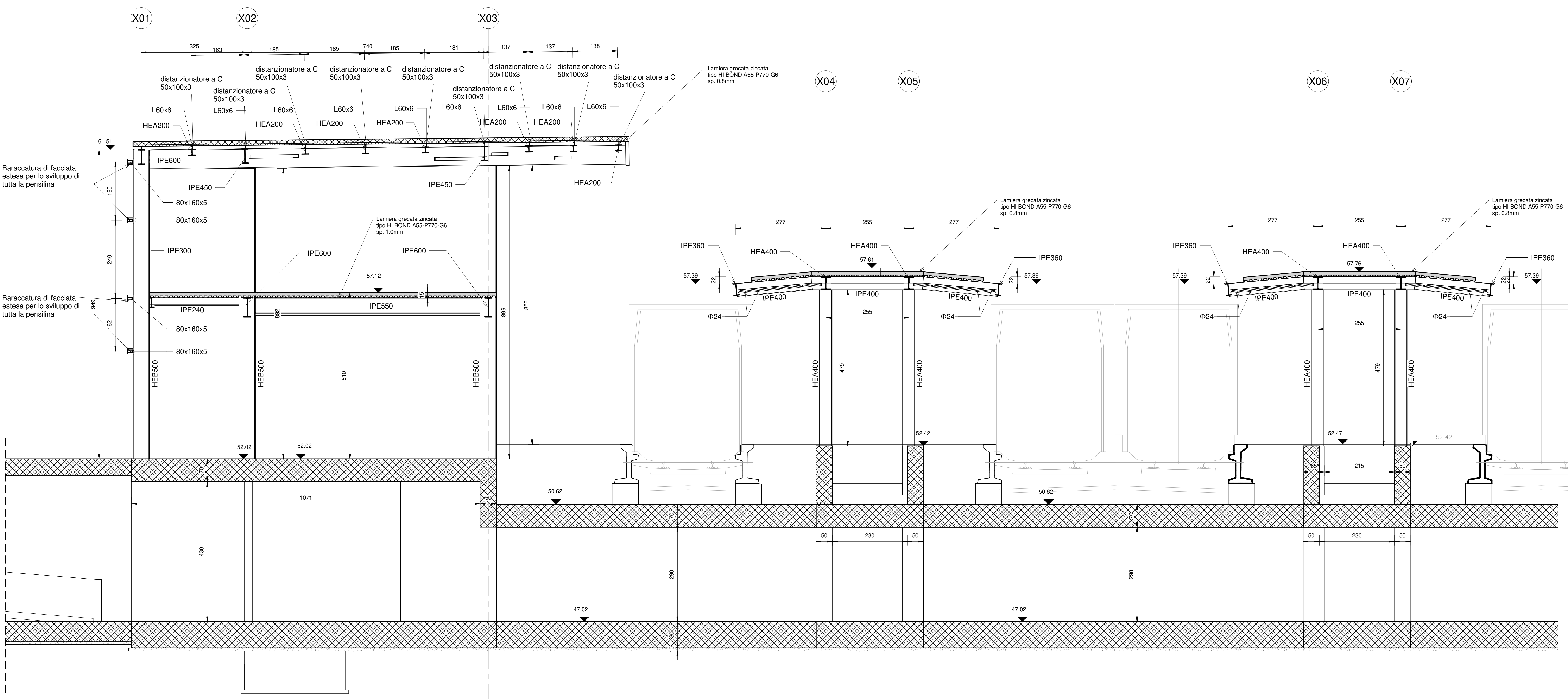
C Pensilia BD - Sezione C-C 1 : 50
