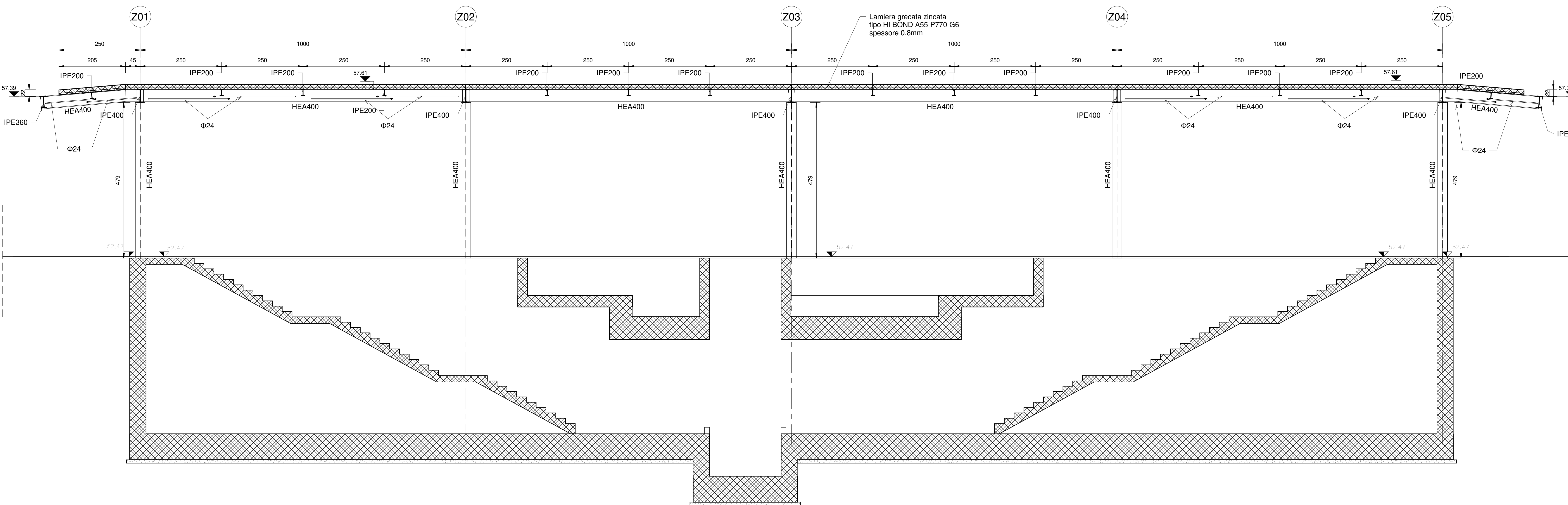
B Pensilia BD - Sezione B-B 1 : 50
