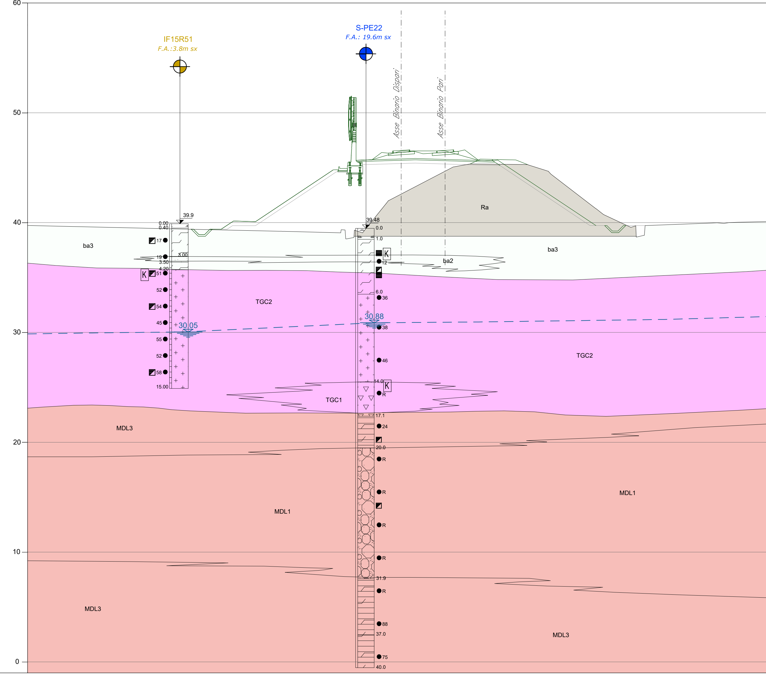
Sez. B-B' - Progr. 17+391.32
