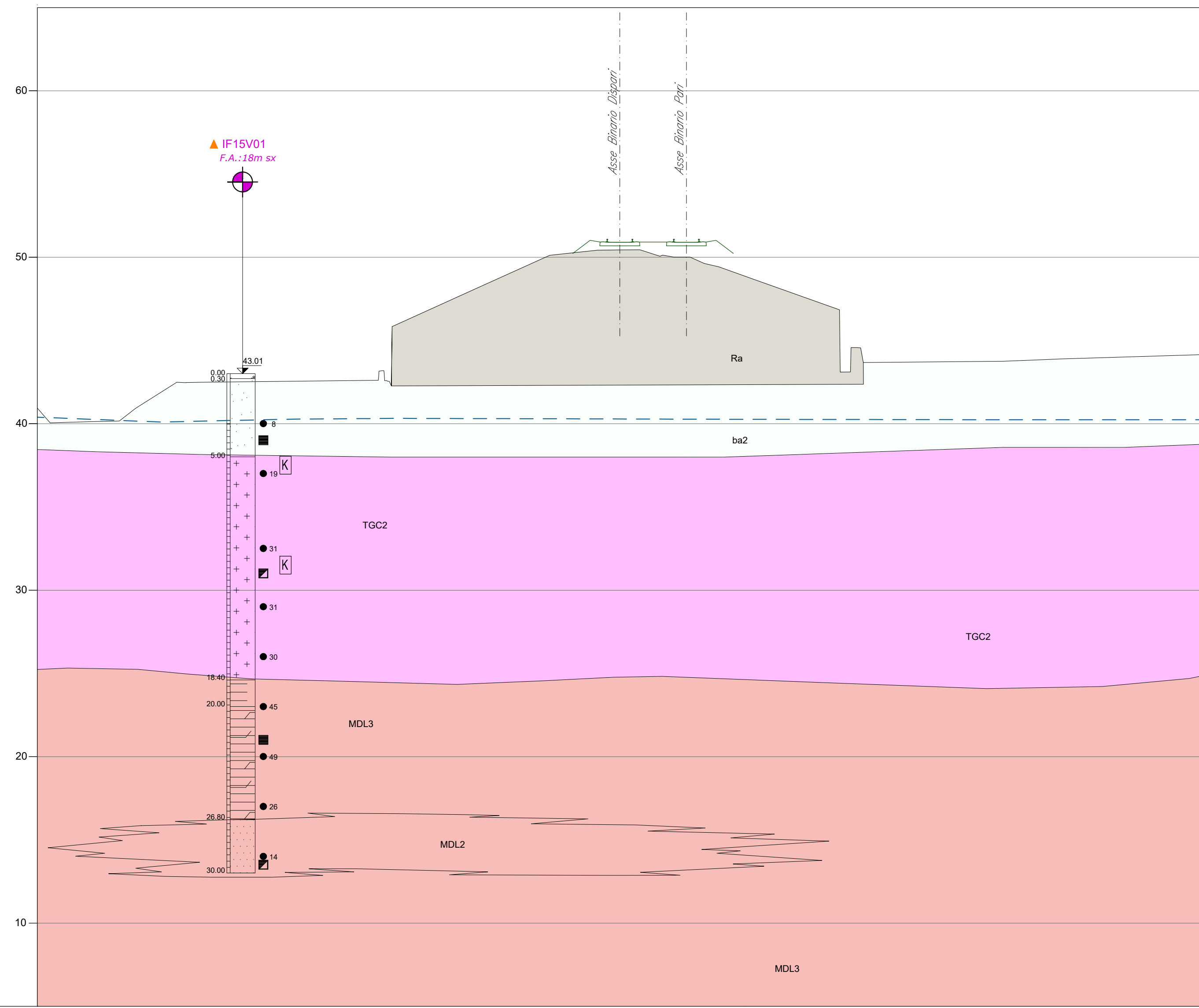
Sez. A-A' - Progr. 16+861.02
