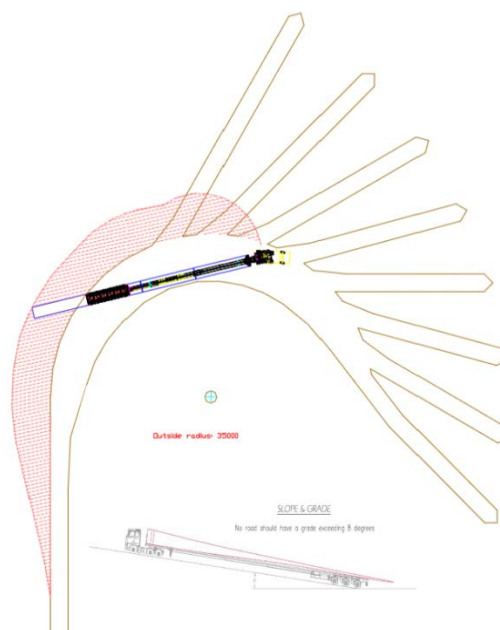
Figura 4 - Raggi minimi di curvatura ed ingombri da assicurare per il transito dei mezzi eccezionali sulla viabilità esterna al parco
