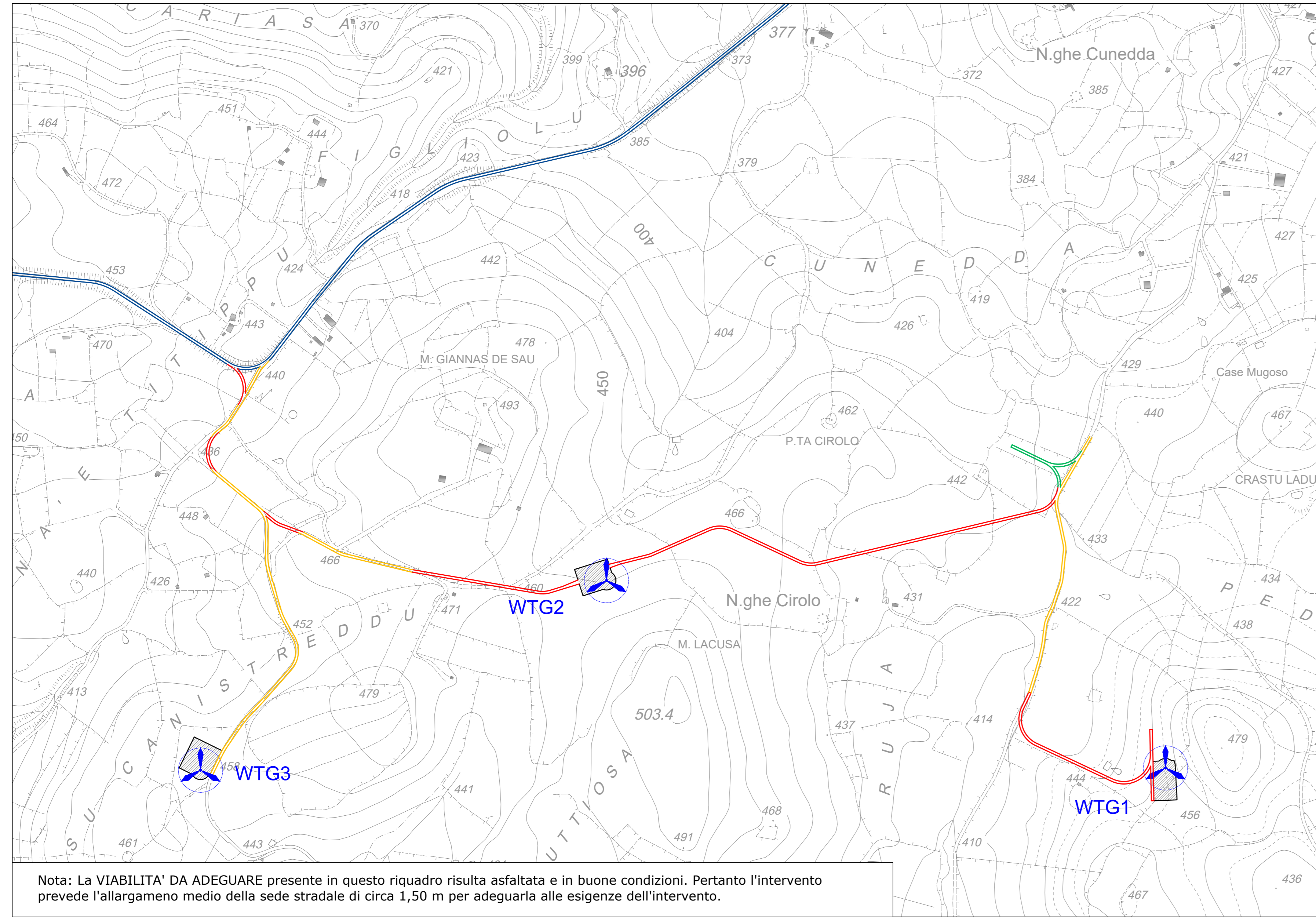
QUADRO A - VIABILITA' PIAZZOLE ED AREE DI CANTIERE ADEGUAMENTI E NUOVA VIABILITÀ - Scala 1:5.000
