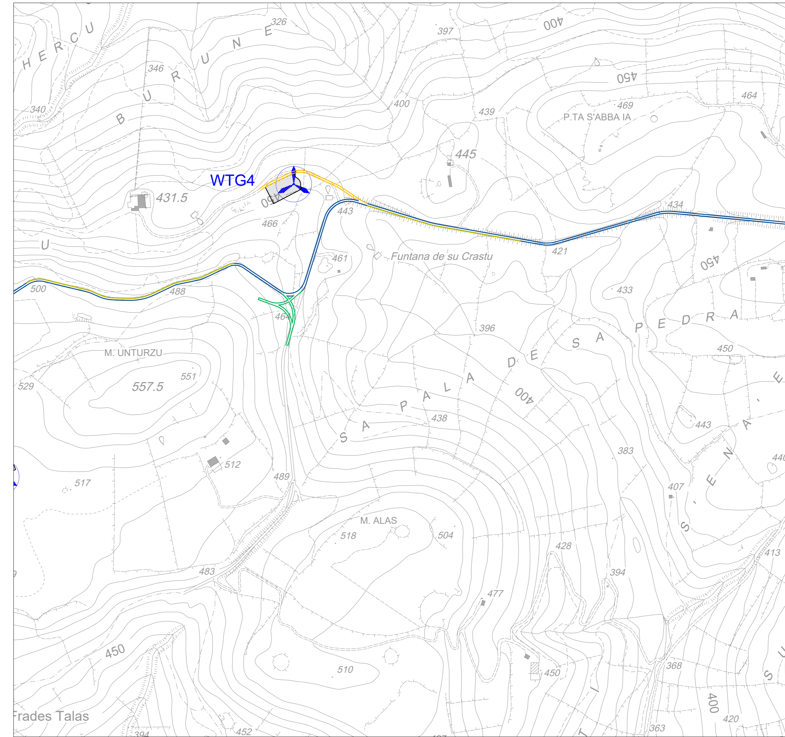
QUADRO B - VIABILITA' PIAZZOLE ED AREE DI CANTIERE ADEGUAMENTI E NUOVA VIABILITÀ - Scala 1:5.000
