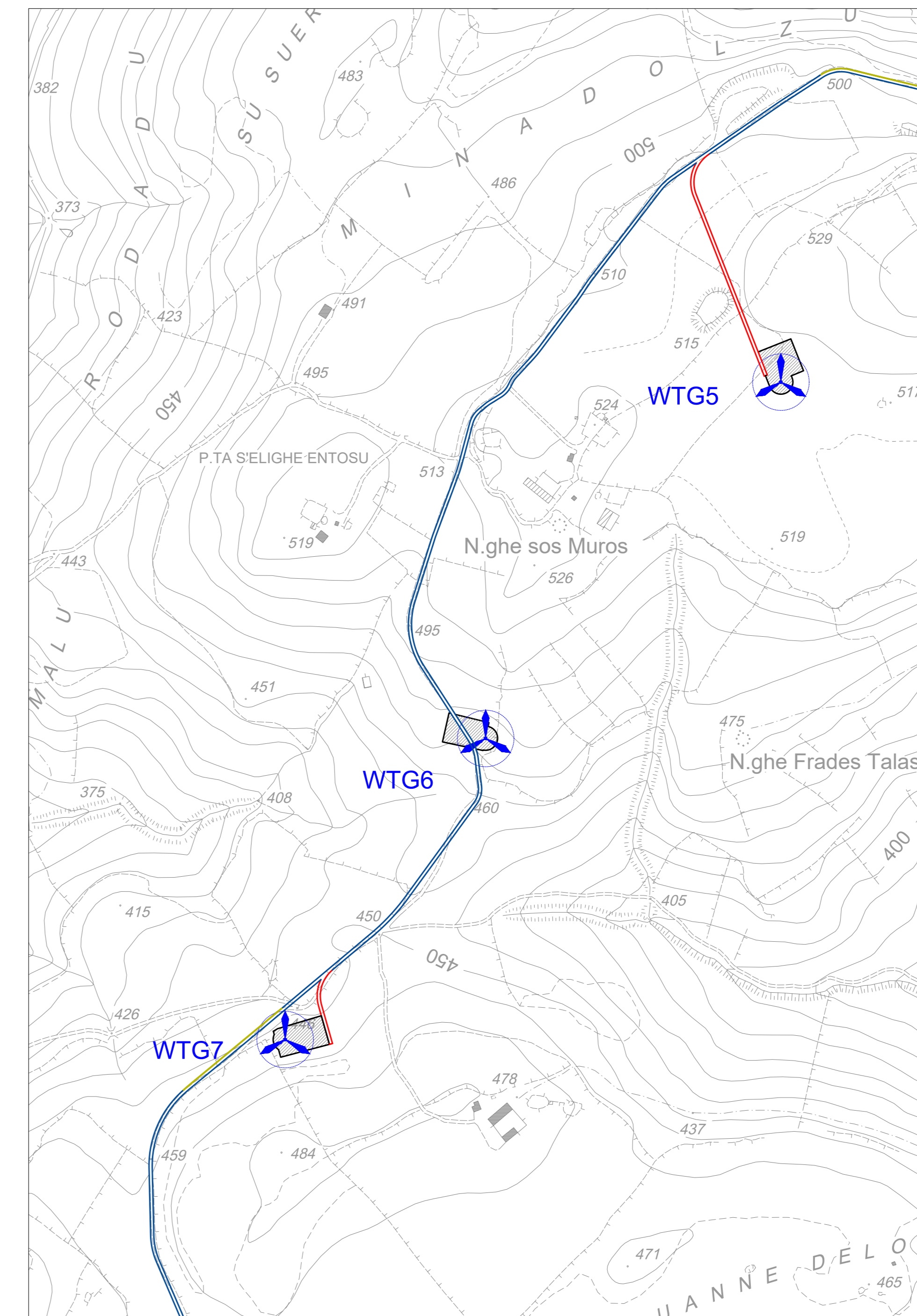
QUADRO D - VIABILITA' PIAZZOLE ED AREE DI CANTIERE ADEGUAMENTI E NUOVA VIABILITÀ - Scala 1:5.000
