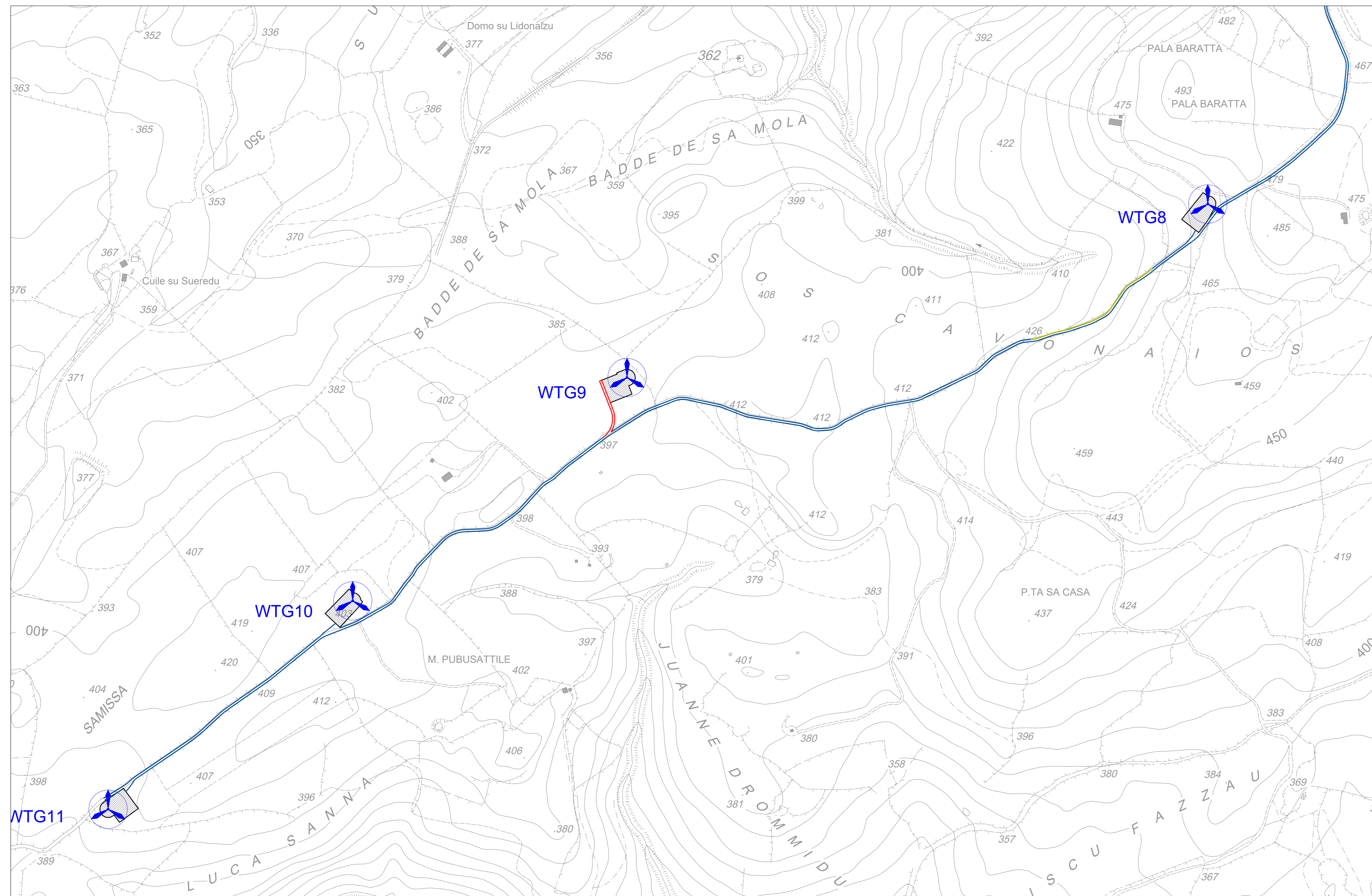
QUADRO C - VIABILITA' PIAZZOLE ED AREE DI CANTIERE ADEGUAMENTI E NUOVA VIABILITÀ - Scala 1:5.000
