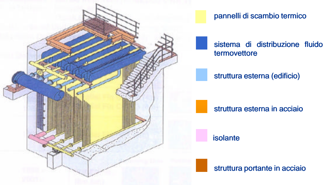
Fig. 10.3 – Schema di un vaporizzatore “Open Rack” con indicazione dei componenti fondamentali.
