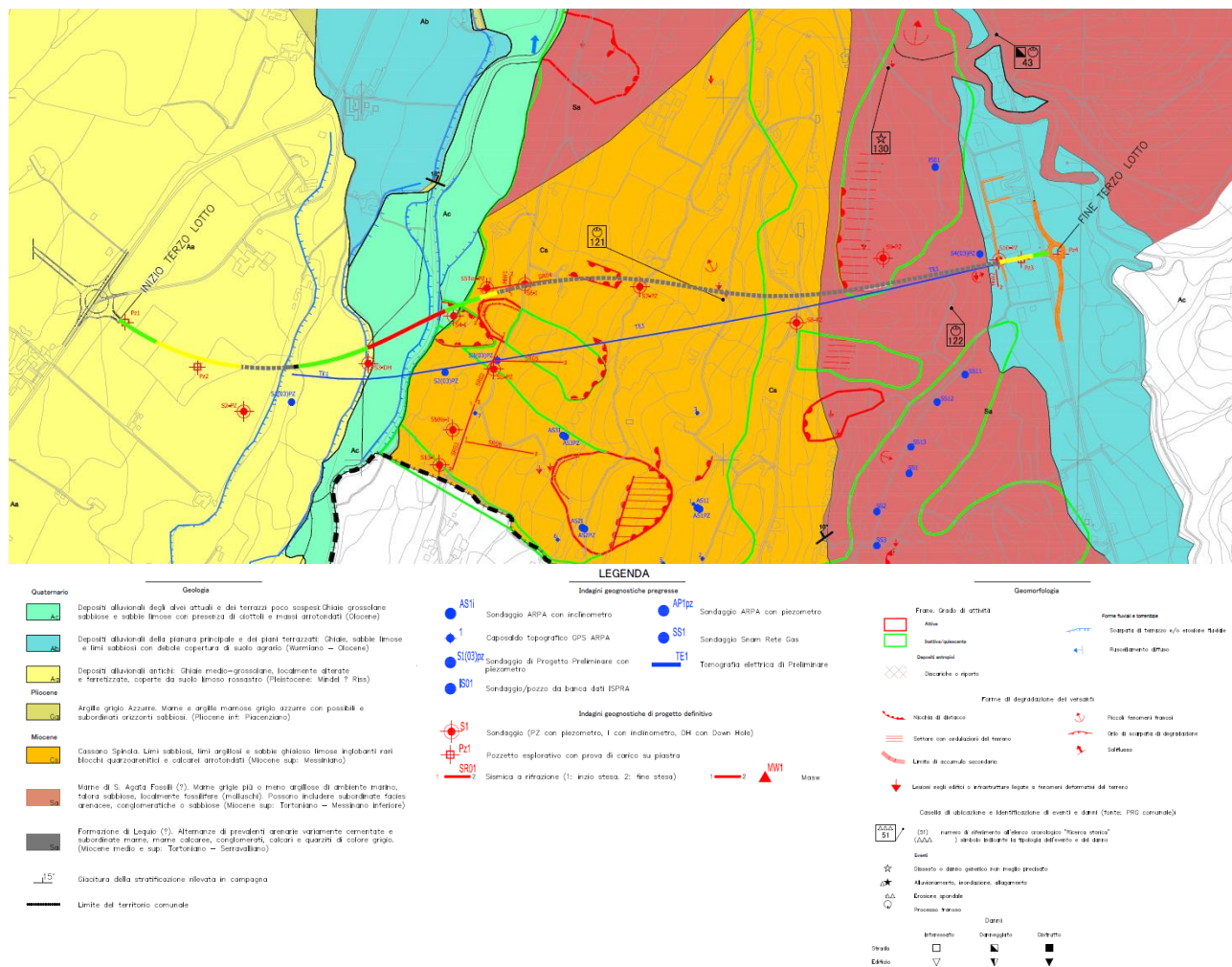
Figura 42 Stralcio carta Geologica e geomorfologica.
