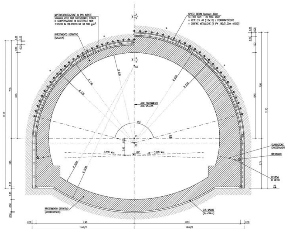
Figura 33: – Sezione tipo B0V
