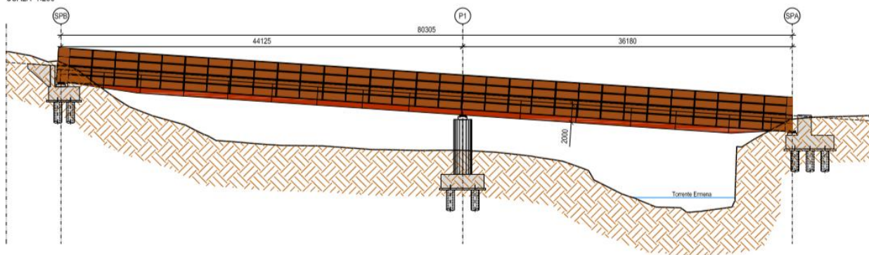
Figura 28: Ponte sul Torrente Ermena - Profilo longitudinale
