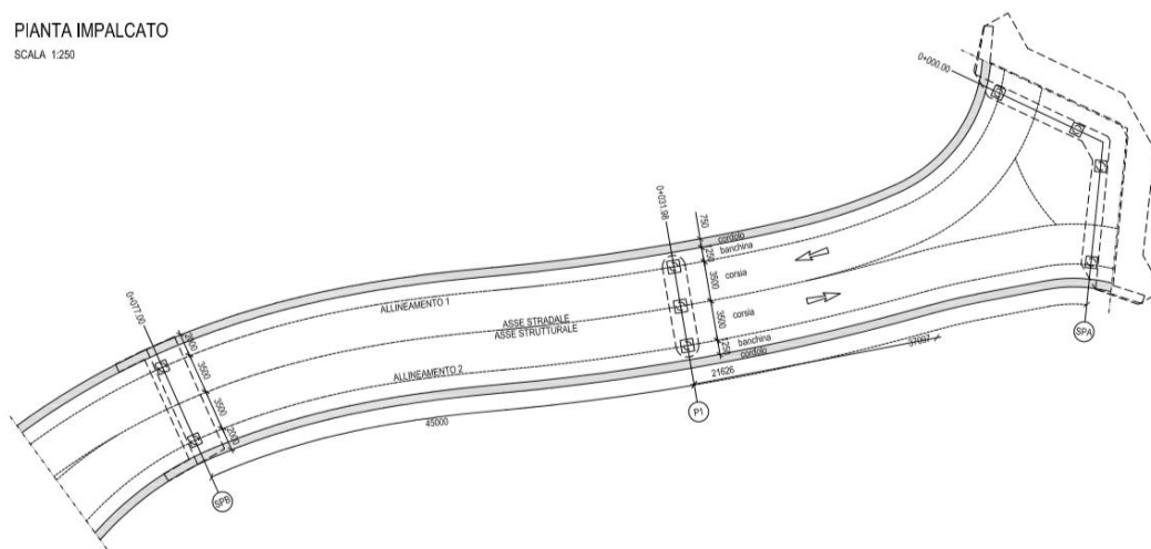
Figura 29: Ponte sul Torrente Ermena – pianta
