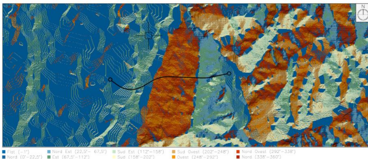
Figura 40 DTM Esposizione.
