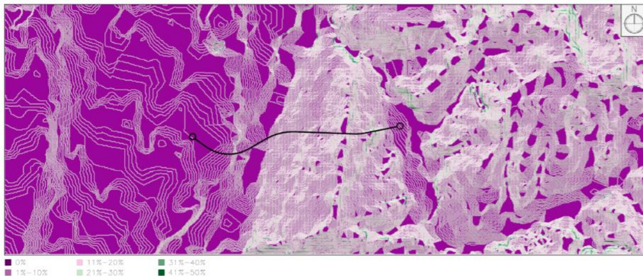
Figura 41 DTM Clivometria.
