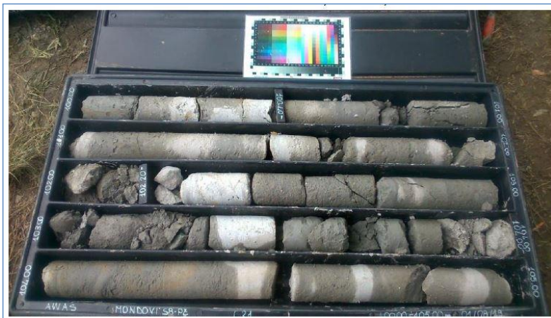
Figura 16 Arenarie della F.ne di Lequio nel sondaggio S8 fra 100-105 m da p.c.
