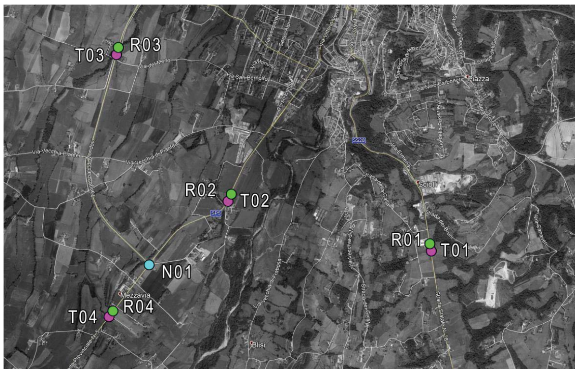
Figura 2.1 – Planimetria dell'area oggetto delle osservazioni di traffico.
