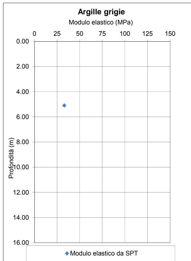
Figura 7.9 Argille Grigio Azzurre. Coesione efficace da prove di laboratorio, coesione non drenata e modulo elastico da SPT
