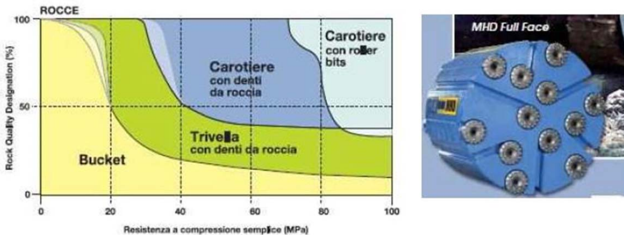
Figura 9.2 A sinistra tipologia di attrezzatura per lo scavo di pali trivellati in funzione della resistenza del terreno. A destra MHD per l'attraversamento di materiali lapidei aventi resistenza fino a 300 MPa (immagine tratta dal catalogo Bauer Maschinen GmbH)
