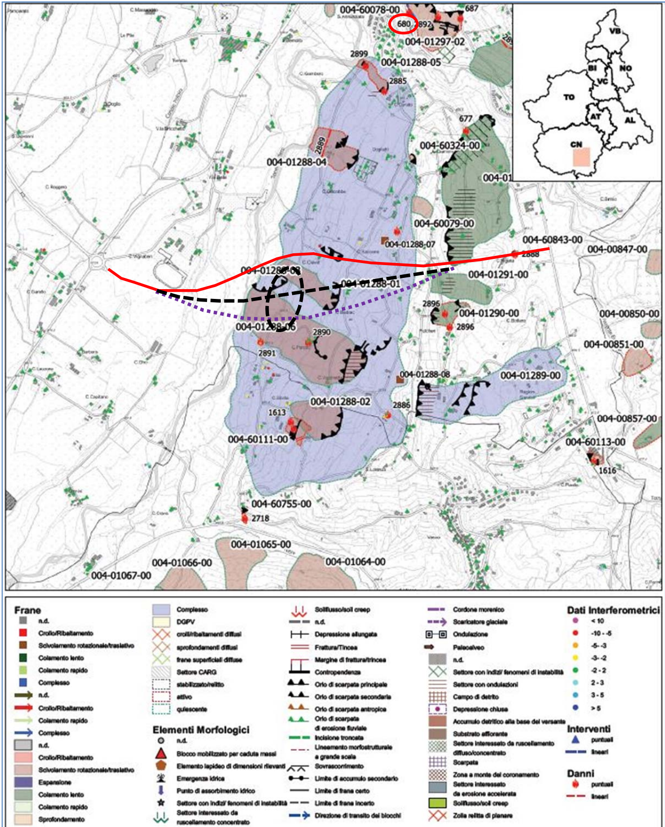
Figura 4.1 Scheda SIFRAP con indicazione del tracciato stradale di progetto definitivo (linea continua rossa). Tratteggiato nero la soluzione di progetto preliminare con l'area impegnata dallo svincolo. Puntinato viola la variante sud. All'estremo nord della carta la posizione del ponte sul Rione Borgato
