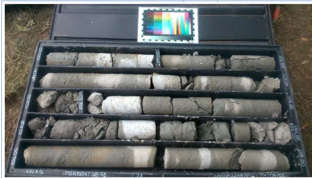
Foto 9.1 Arenarie (della F.ne di Lequio) nel sondaggio S8 fra 100-105 m da p.c.
