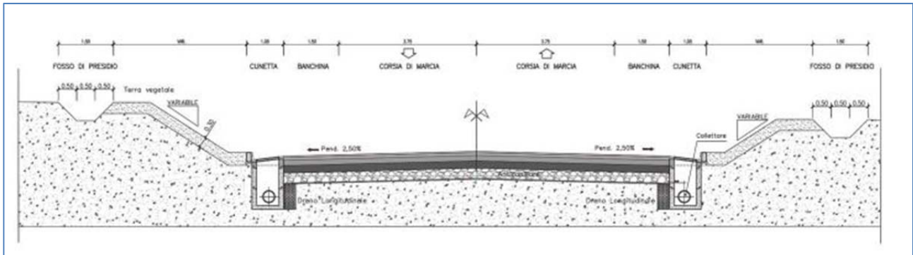
Figura 9.1 Sezione tipo scavi in trincea
