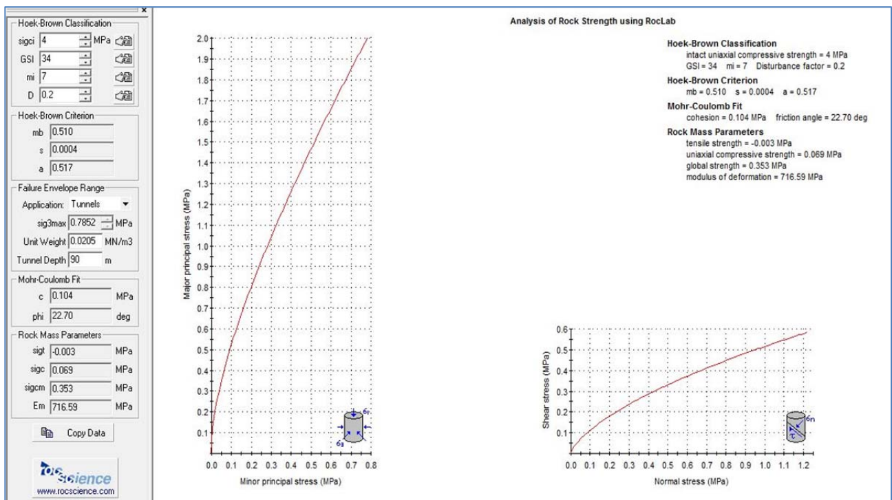
Figura 7.25 Marne di S. Agata Fossili: caratterizzazione secondo il criterio di Hoek-Brown e Mohr-Coulomb per copertura 90m.
