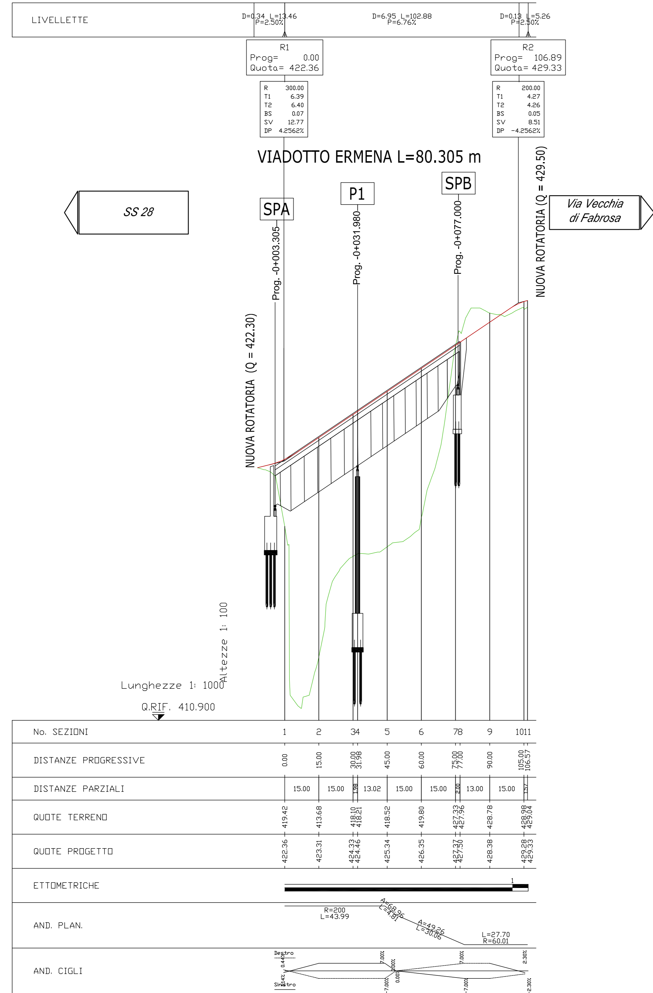
Profilo longitudinale Scala 1:1.000
