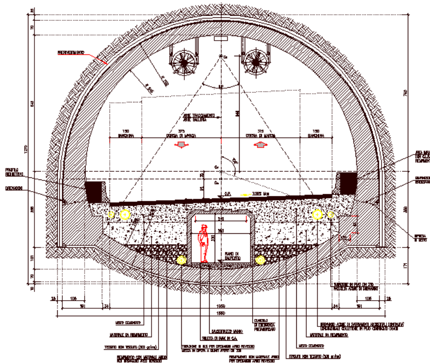
Figura 5.2 Sezione tipo della galleria San Lorenzo
