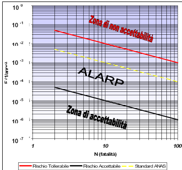
Figura 9.11 Criterio ALARP
