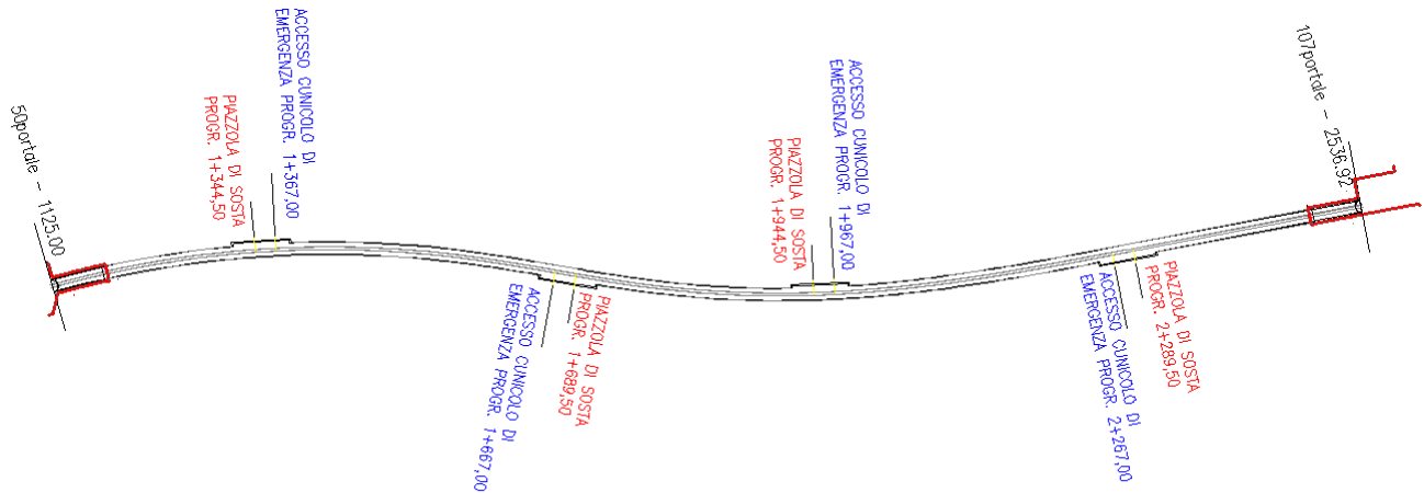
Figura 5.1 Planimetria della galleria San Lorenzo
