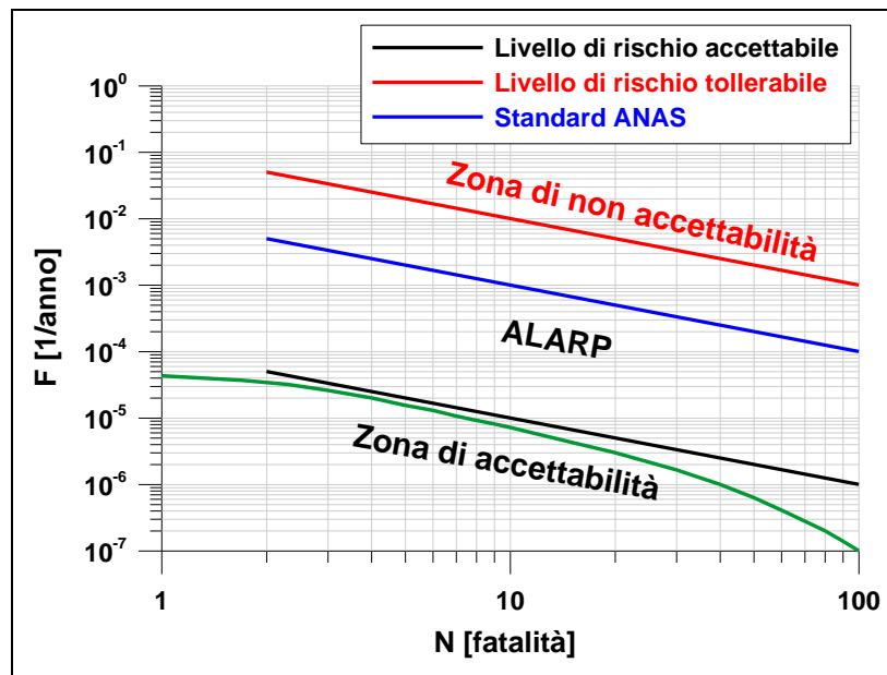
Figura 9.12 Curva F-N cumulata complementare complessiva
