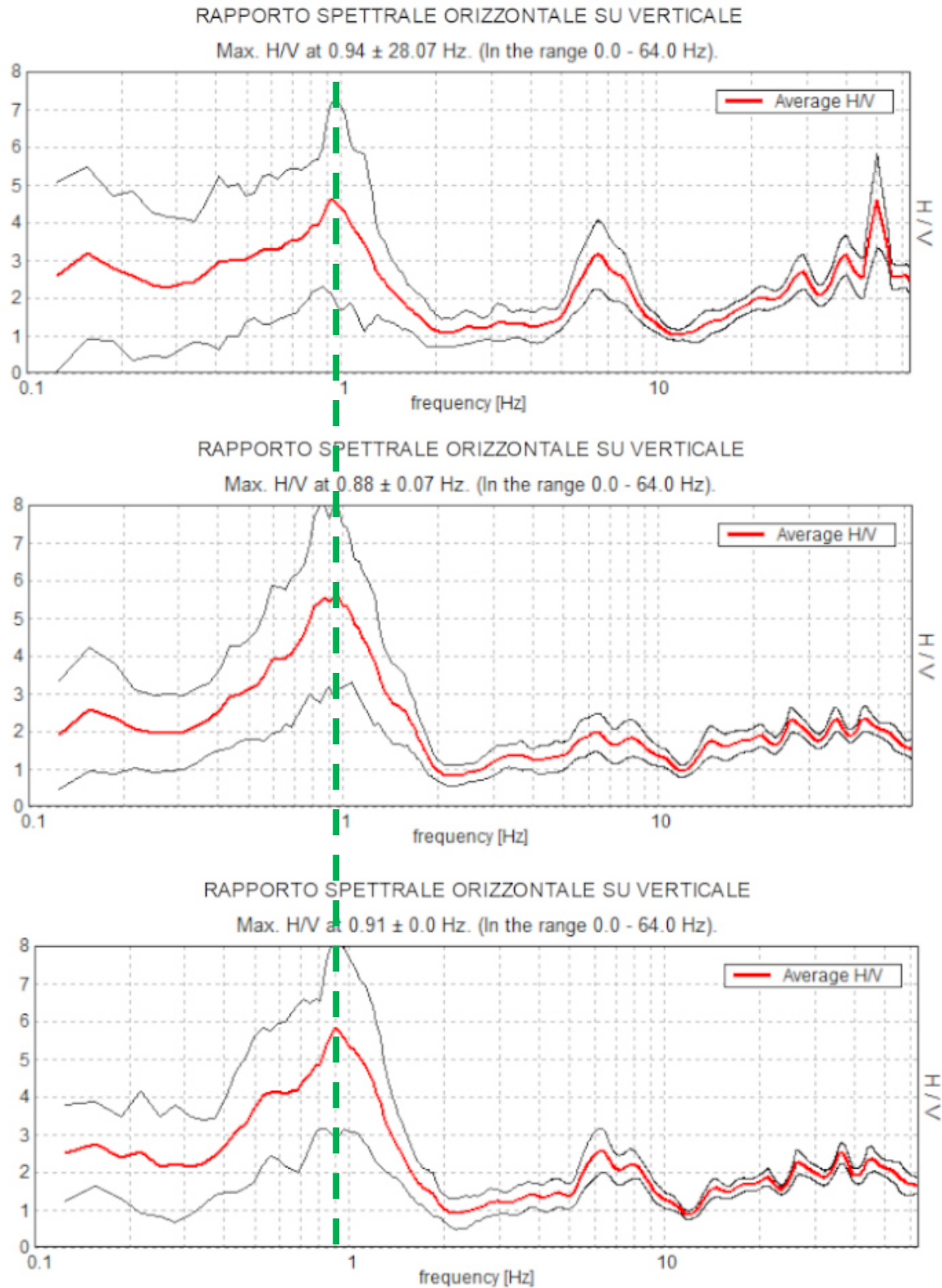
FIGURA 5-1 - RISULTATI DETERMINAZIONI H/V - HV08.
