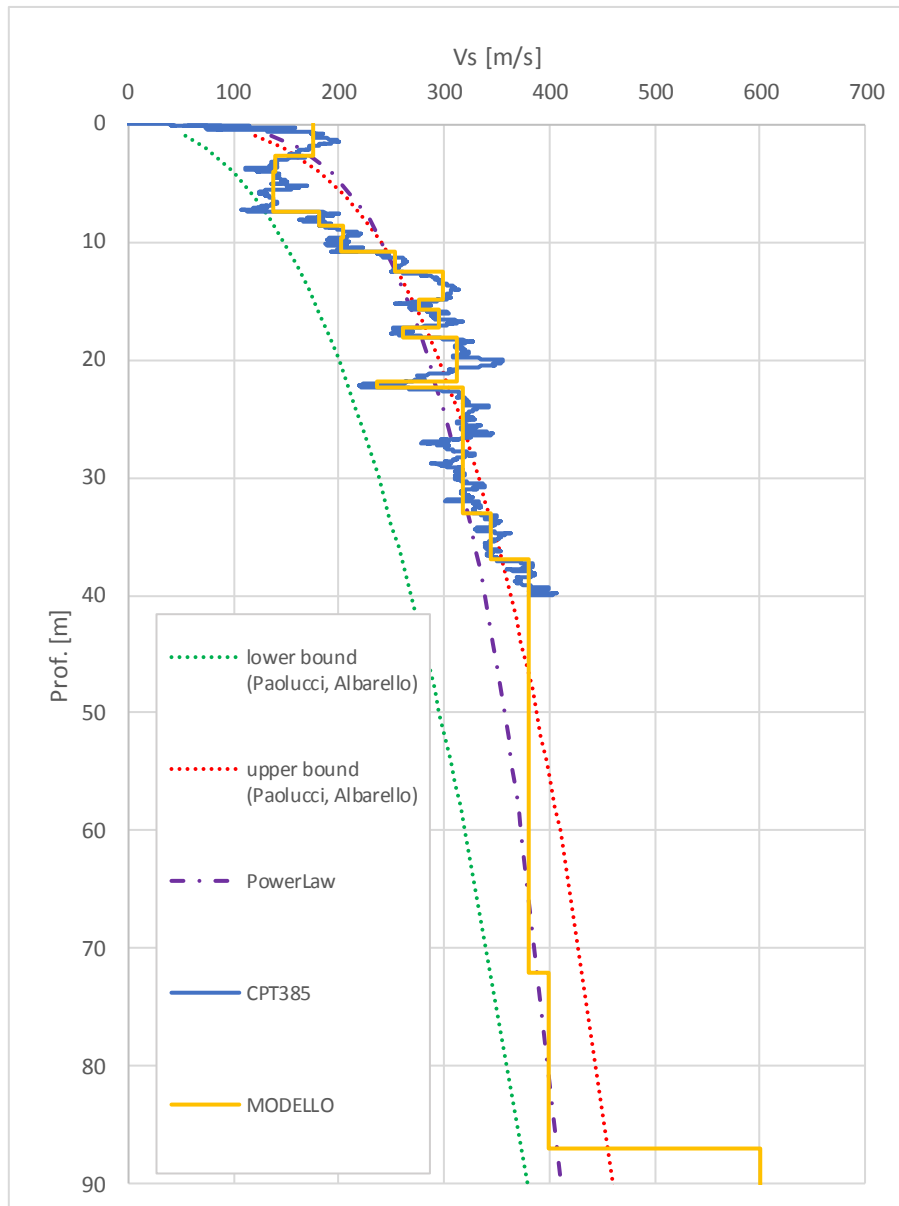
FIGURA 4-1 - PROFILO DI VS LUNGO LA VERTICALE DI INDAGINE CPTU 385.
