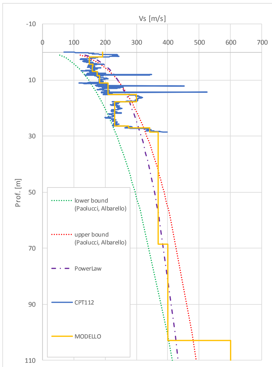
FIGURA 4-1 - PROFILO DI VS LUNGO LA VERTICALE DI INDAGINE CPTU 112.
