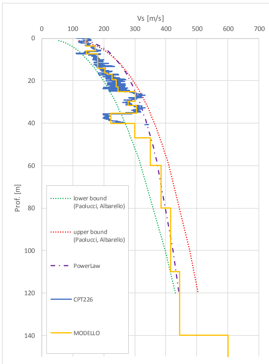
FIGURA 4-1 - PROFILO DI Vs LUNGO LA VERTICALE DI INDAGINE CPTU 226.
