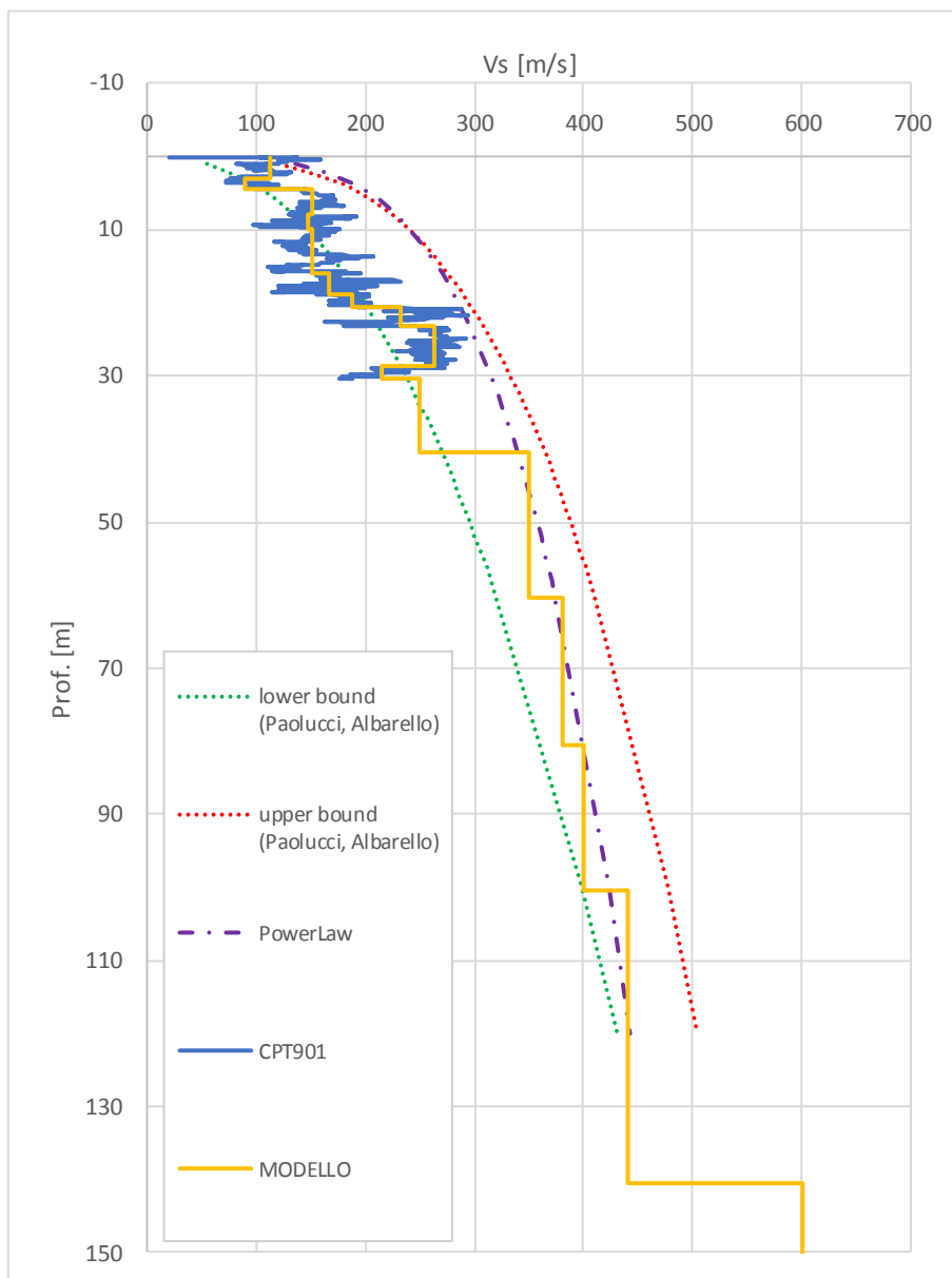
FIGURA 4-1 - PROFILO DI Vs LUNGO LA VERTICALE DI INDAGINE CPTU 901.
