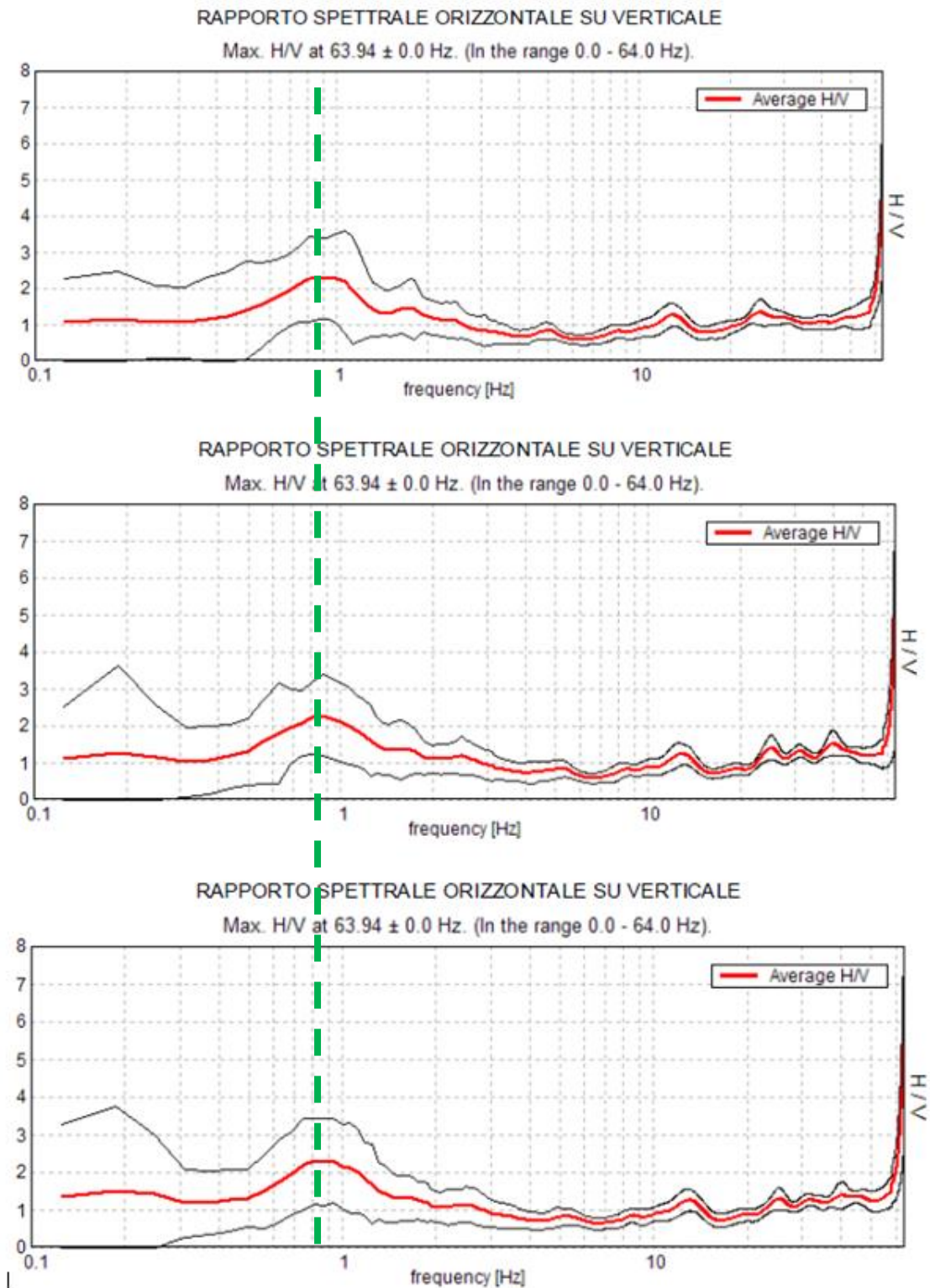
FIGURA 5-1 - RISULTATI DETERMINAZIONI H/V - HV02.
