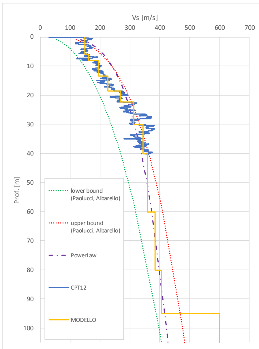
FIGURA 4-1 - PROFILO DI Vs LUNGO LA VERTICALE DI INDAGINE CPTU 12.
