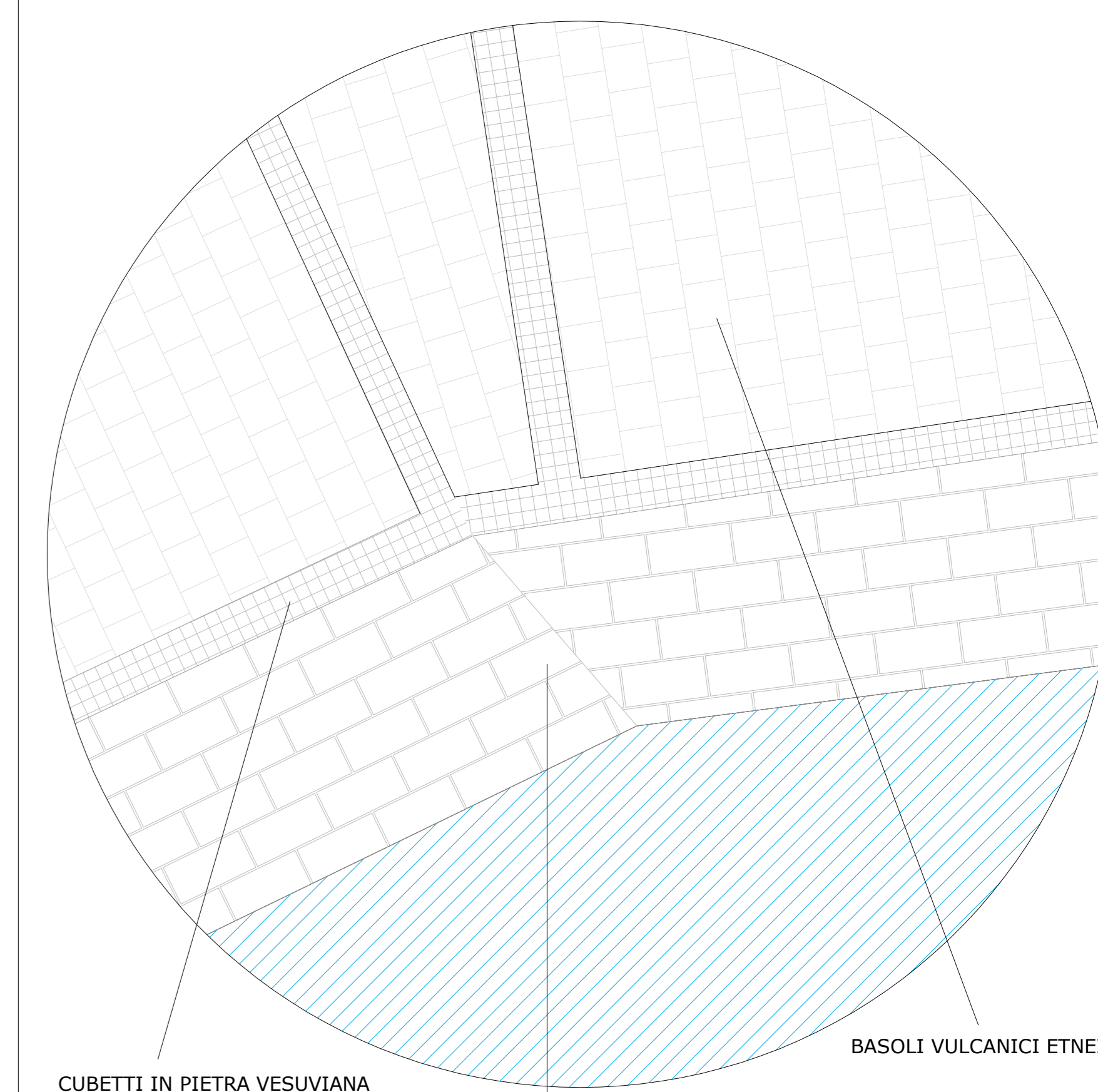
CUBETTI IN PIETRA VESUVIANA PAVIMENTAZIONE ESISTENTE IN BASOLI VESUVIANI BASOLI VULCANICI ETNEI
