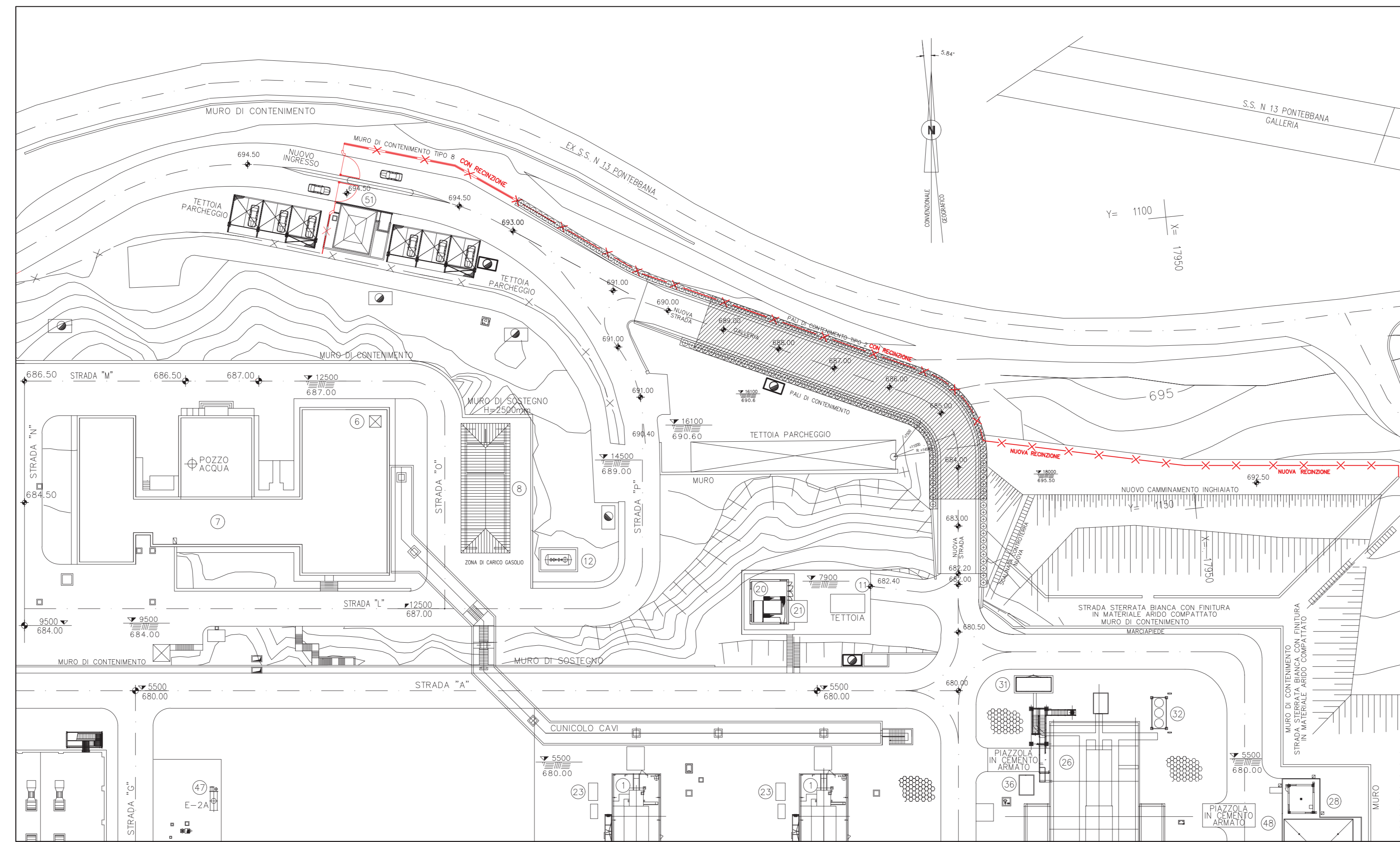
PIANTA CHIAVE - AREA IMPIANTO SNAM
