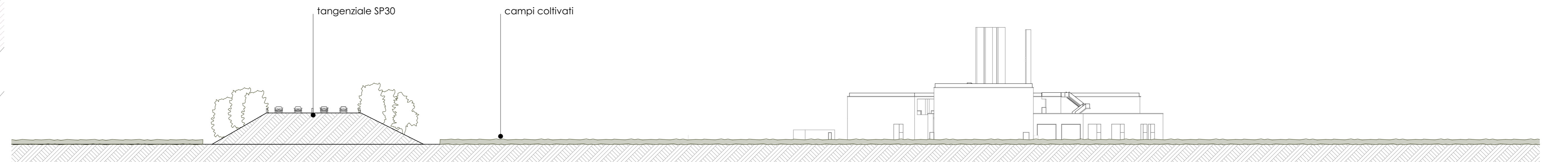
Approfondimento Sezione ambientale bb', scala 1:500 VOLUMETRIE GIA' ESISTENTI
