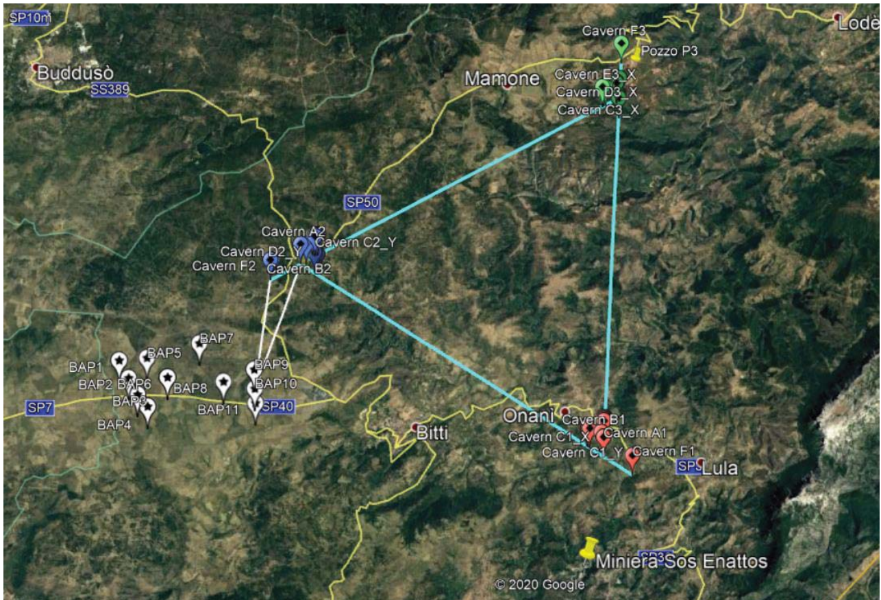
Figura 2 – Tracciato complessivo (in azzurro) di Einstein Telescope; pale eoliche contrassegnate da segnaposto bianco.
