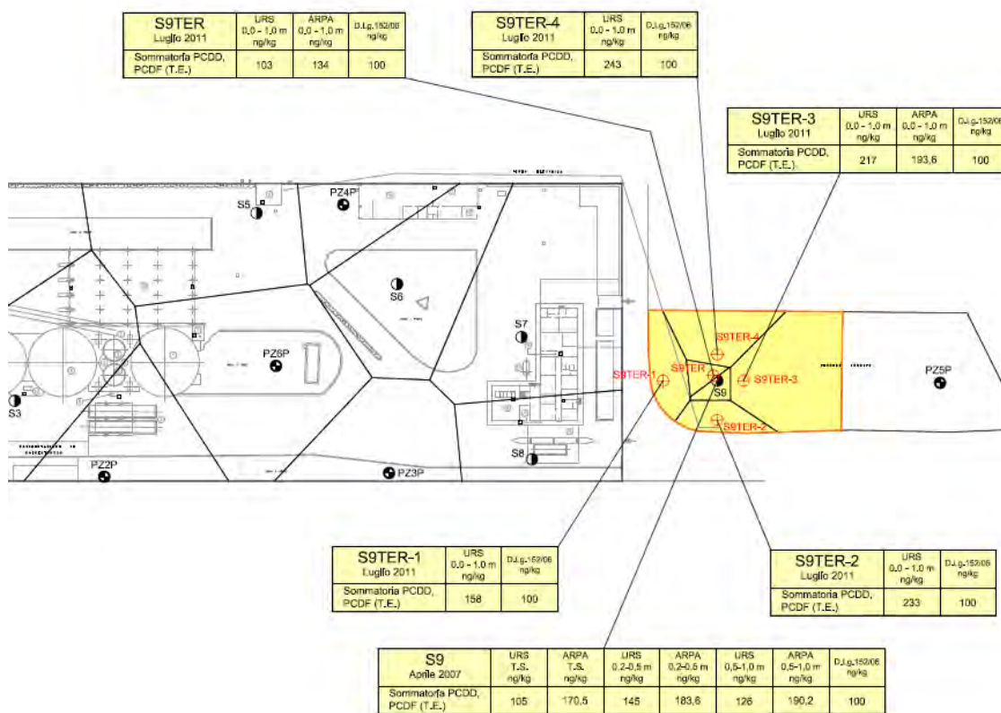
Fig. 4.3 - Superamenti terreni – Sorgente S9 – Suolo Superficiale
