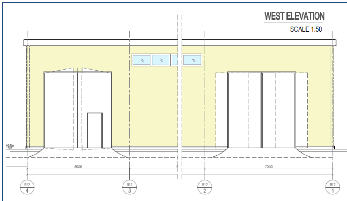
Figura 2 Prospetto Ovest "Edificio ausiliari"
