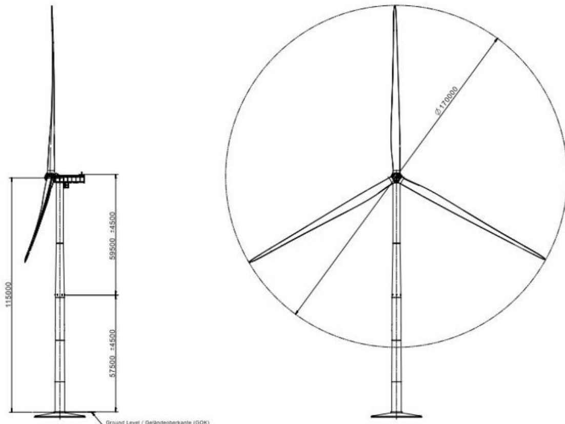
Figura 2: Vista e caratteristiche dell'aerogeneratore di riferimento
