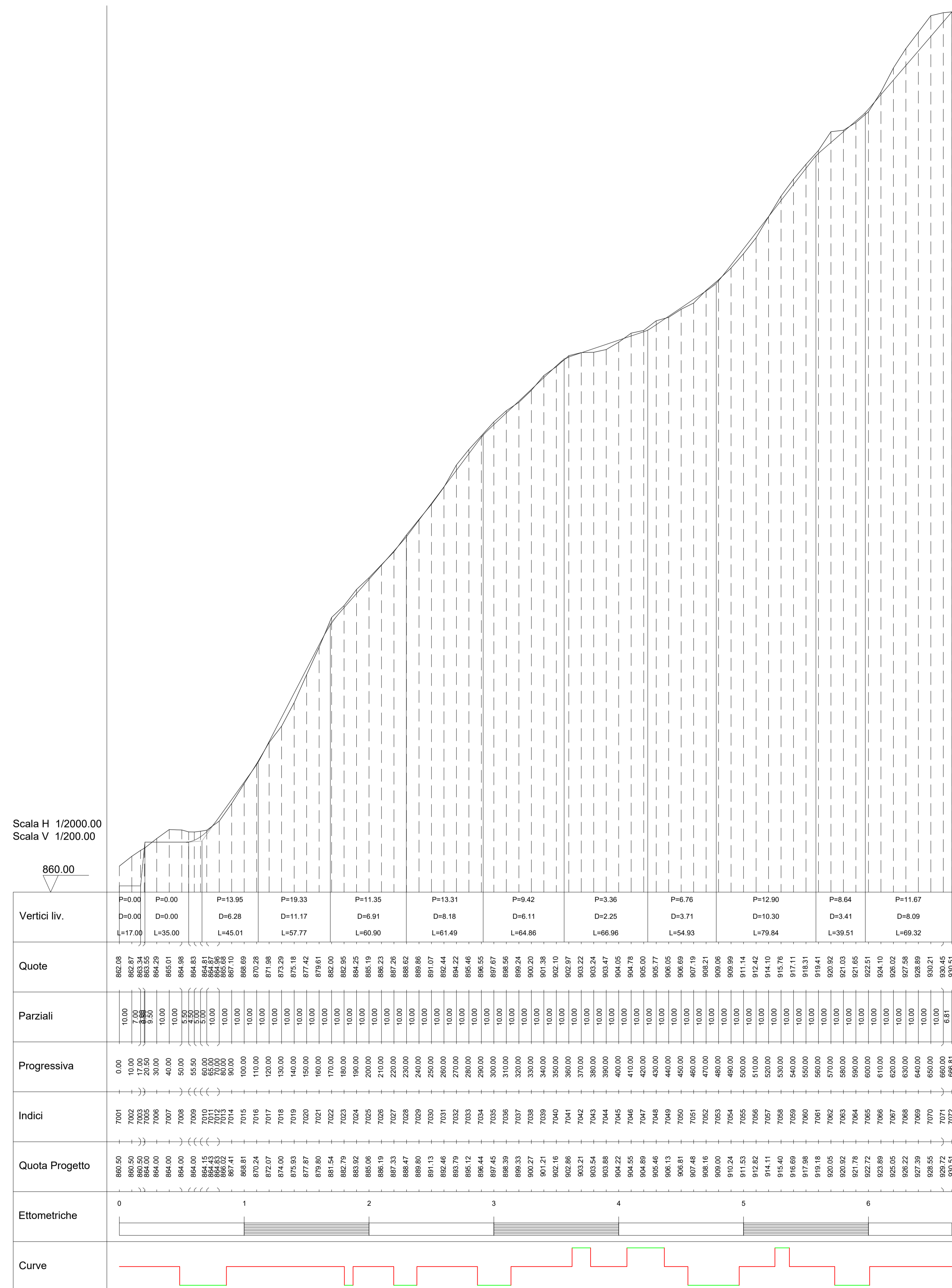
WTG 07 - PROFILO LONGITUDINALE
