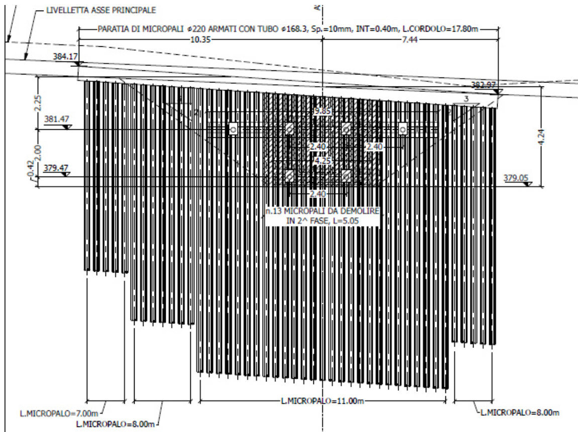
Figura 1-2: Prospetto
