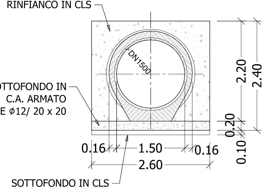
TUBO IN C.A. DN 1500 SEZIONE A-A scala 1:50
